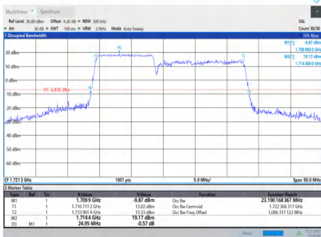
66-66-10MHz-15MHz-QPSK-QPSK-132351-132471-50RB#0-75RB#0
