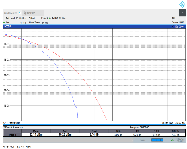
66-66-10MHz-10MHz-QPSK-QPSK-132373-132472-50RB#0-50RB#0
