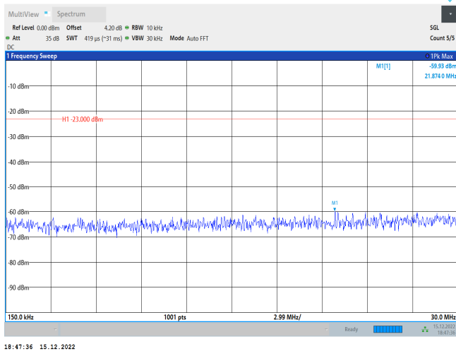
66-66-10MHz-10MHz-QPSK-QPSK-132022-132121-1RB#0-0RB#0-0.15~30MHz
