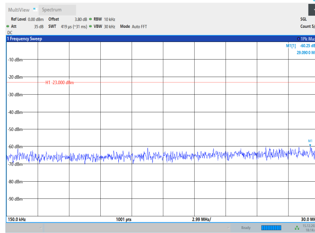
Band26-10MHz-QPSK-26740-1RB#0-Range2:0.15~30MHz
