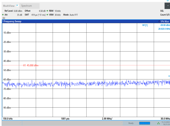
Band7-20MHz-QPSK-20850-1RB#0-Range2:0.15~30MHz
