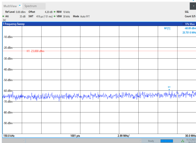
Band4-20MHz-QPSK-20050-1RB#0-Range2:0.15~30MHz
