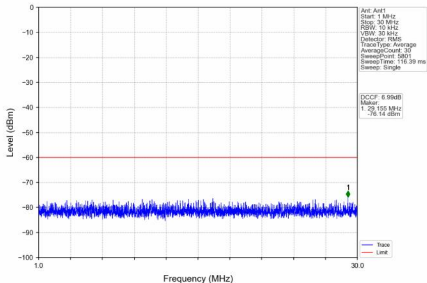
n48_30kHz_SISO_NTNV_40MHz_CP-OFDM QPSK_3570MHz_Inner_1RB_Left
