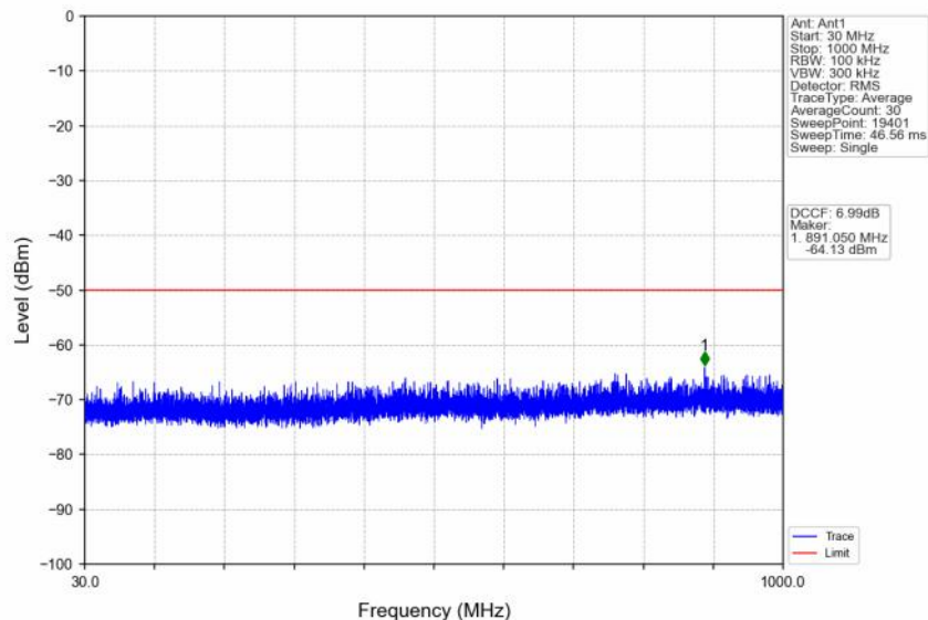
n48_30kHz_SISO_NTNV_40MHz_DFT-s-OFDM_QPSK_3570MHz_Inner_1RB_Left
