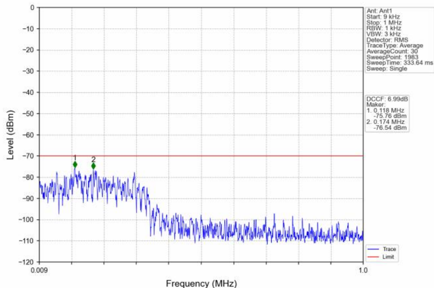
n48_30kHz_SISO_NTNV_40MHz_DFT-s-OFDM_QPSK_3570MHz_Inner_1RB_Left
