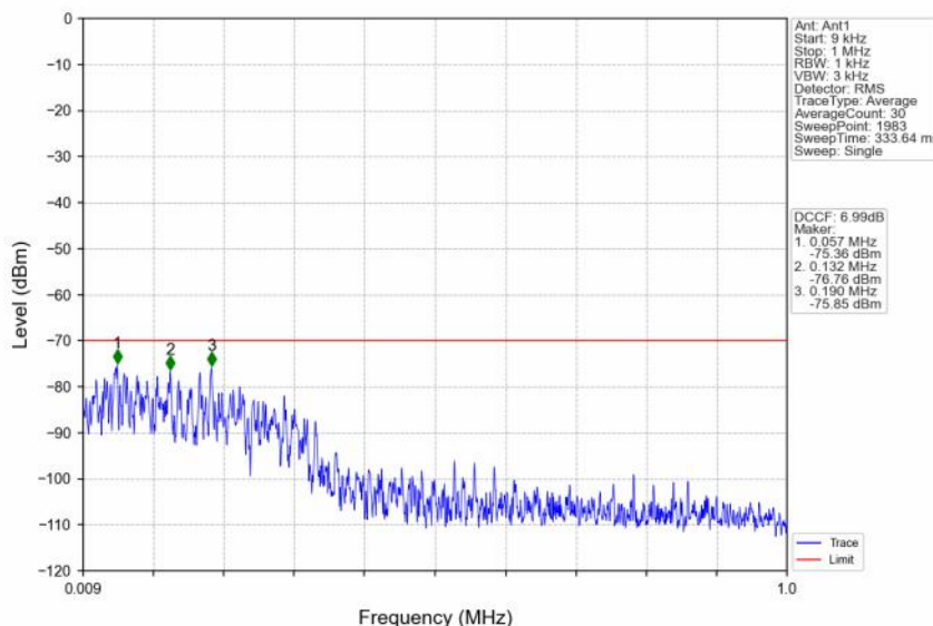
n48_30kHz_SISO_NTNV_40MHz_CP-OFDM QPSK_3570MHz_Edge_1RB_Left
