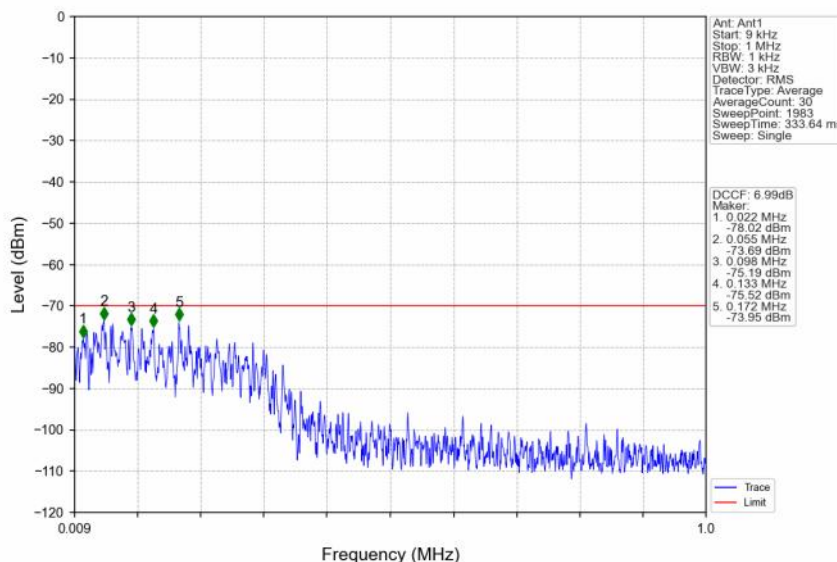
n48_30kHz_SISO_NTNV_40MHz_CP-OFDM QPSK_3570MHz_Inner_1RB_Left
