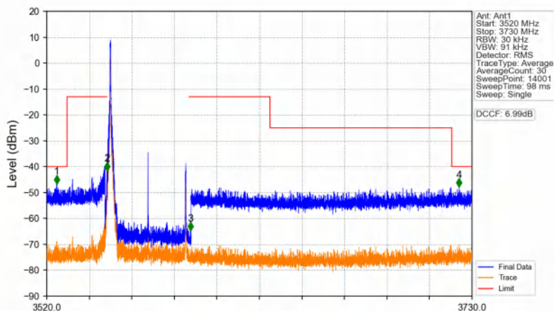
n48_30kHz_SISO_NTNV_40MHz_DFT-s-OFDM PI/2 BPSK_3570MHz_Inner_1RB_Left
