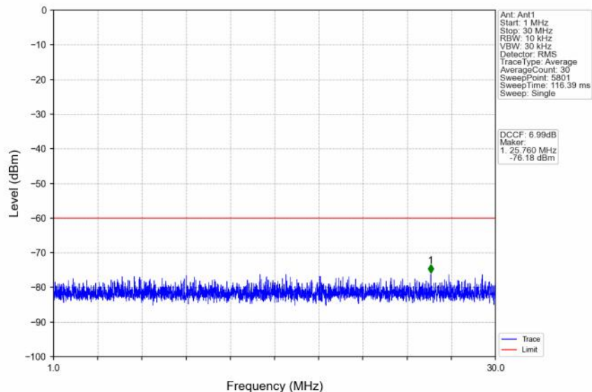
n48_30kHz_SISO_NTNV_40MHz_CP-OFDM QPSK_3570MHz_Edge_1RB_Left
