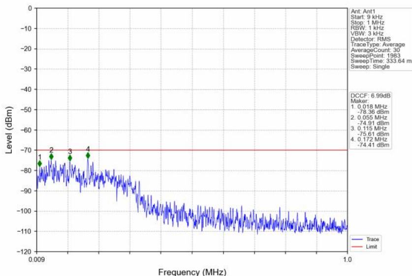
n48_30kHz_SISO_NTNV_20MHz_CP-OFDM QPSK_3560.01MHz_Inner_1RB_Left
