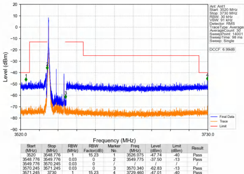
n48_30kHz_SISO_NTNV_20MHz_CP-OFDM QPSK_3560.01MHz_Inner_1RB_Left
