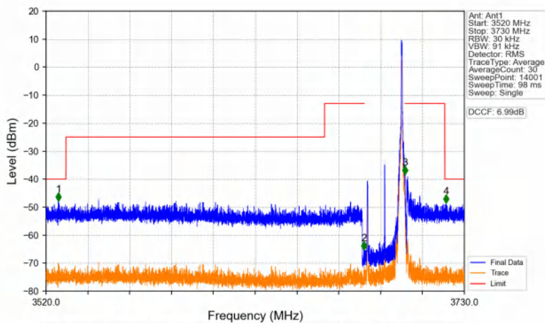
n48_30kHz_SISO_NTNV_20MHz_DFT-s-OFDM QPSK_3690MHz_Inner_1RB_Right
