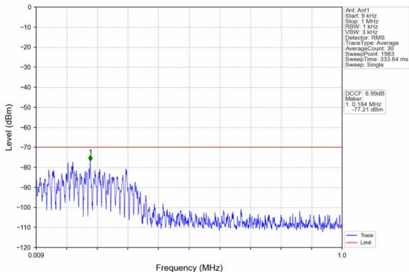
n48_30kHz_SISO_NTNV_20MHz_DFT-s-OFDM QPSK_3690MHz_Inner_1RB_Right
