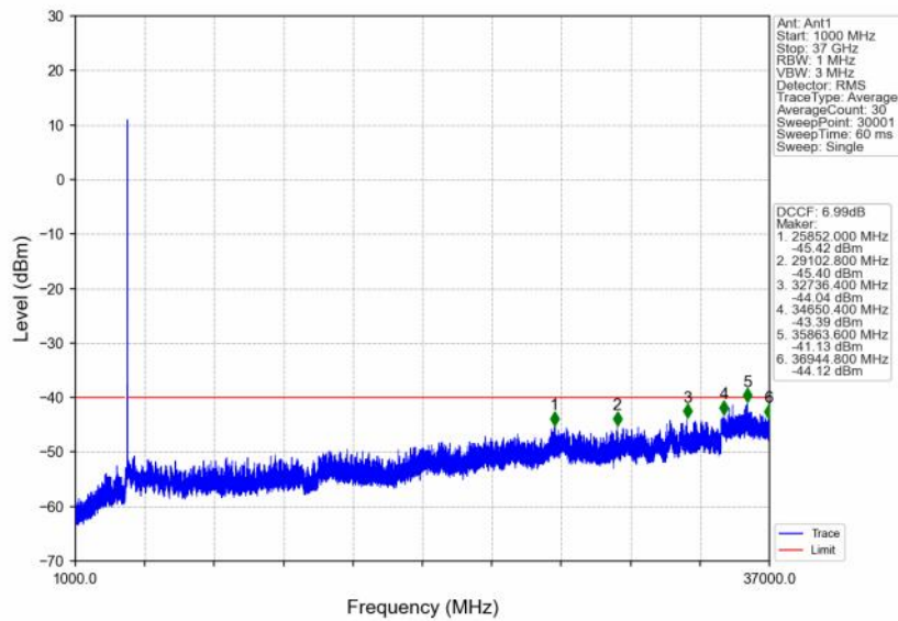
n48_30kHz_SISO_NTNV_20MHz_CP-OFDM QPSK_3690MHz_Inner_1RB_Right
