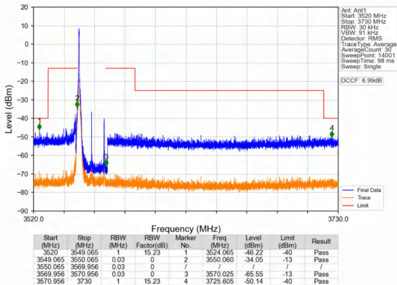
n48_30kHz_SISO_NTNV_20MHz_DFT-s-OFDM PI/2 BPSK_3560.01MHz_Inner_1RB_Left
