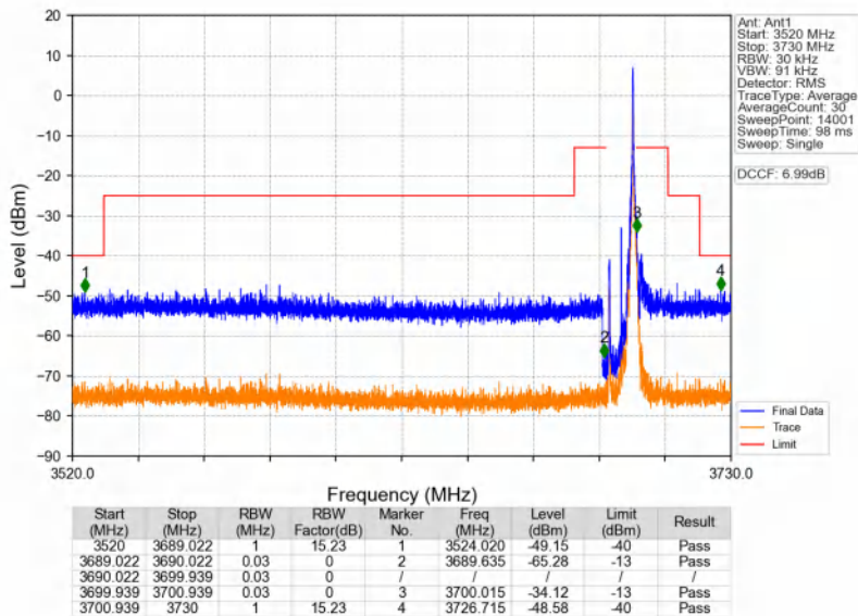
n48_30kHz_SISO_NTNV_10MHz_DFT-s-OFDM PI/2 BPSK_3694.98MHz_Inner_1RB_Right
