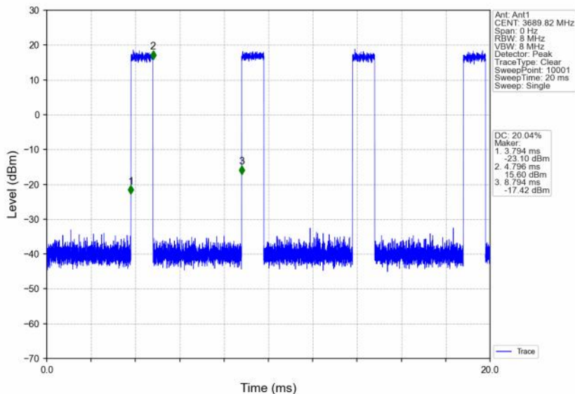
n48_30kHz_SISO_NTNV_20MHz_DFT-s-OFDM QPSK_3690MHz_Inner_Full
