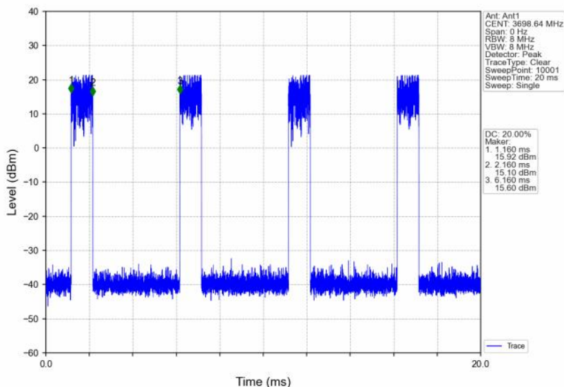
n48_30kHz_SISO_NTV_20MHz_CP-OFDM 16 QAM_3690MHz_Inner_1RB_Right
