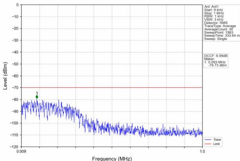
n48_30kHz_SISO_NTV_40MHz_CP-OFDM QPSK_3679.98MHz_Inner_1RB_Right
