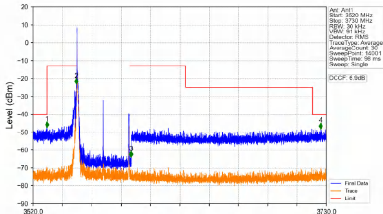
n48_30kHz_SISO_NTNV_40MHz_DFT-s-OFDM PI/2 BPSK_3570MHz_Inner_1RB_Left
