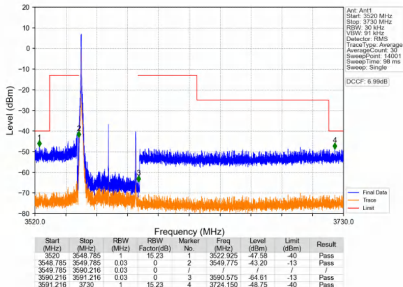
n48_30kHz_SISO_NTNV_40MHz_CP-OFDM_QPSK_3570MHz_Inner_1RB_Left
