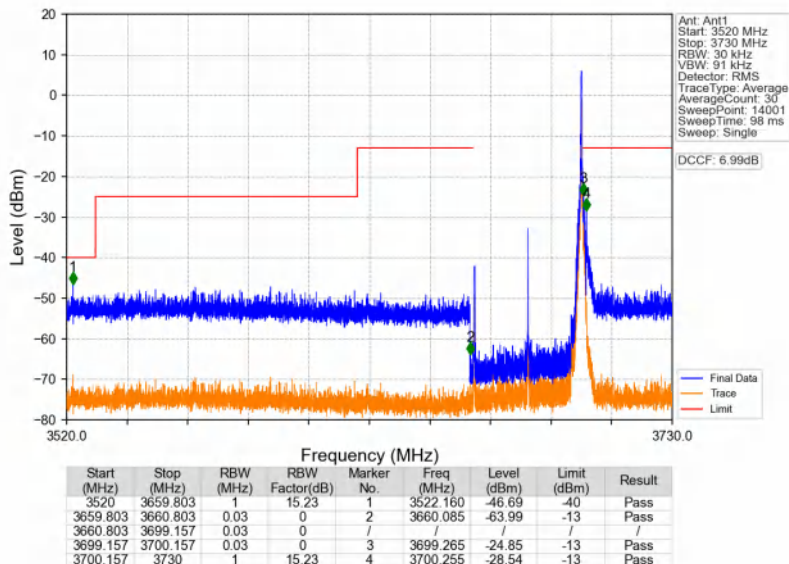
n48_30kHz_SISO_NTV_40MHz_CP-OFDM QPSK_3679.98MHz_Inner_1RB_Right
