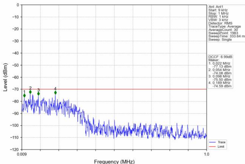
n48_30kHz_SISO_NTNV_10MHz_CP-OFDM QPSK_3555MHz_Inner_1RB_Left
