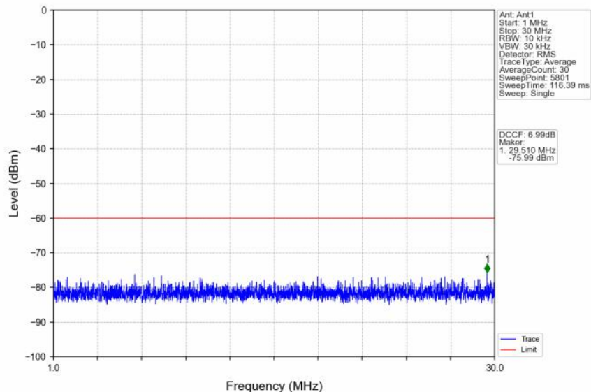
n48_30kHz_SISO_NTNV_20MHz_CP-OFDM QPSK_3560.01MHz_Inner_1RB_Left
