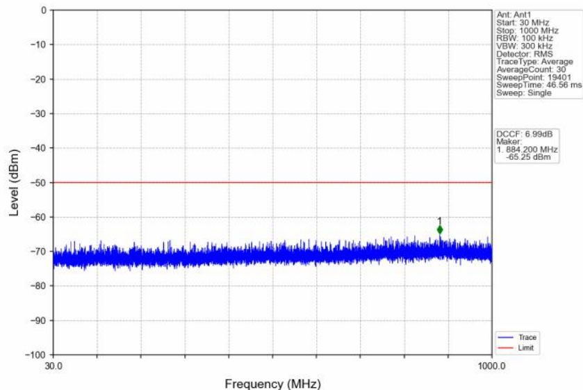
n48_30kHz_SISO_NTNV_20MHz_CP-OFDM QPSK_3624.99MHz_Edge_1RB_Left
