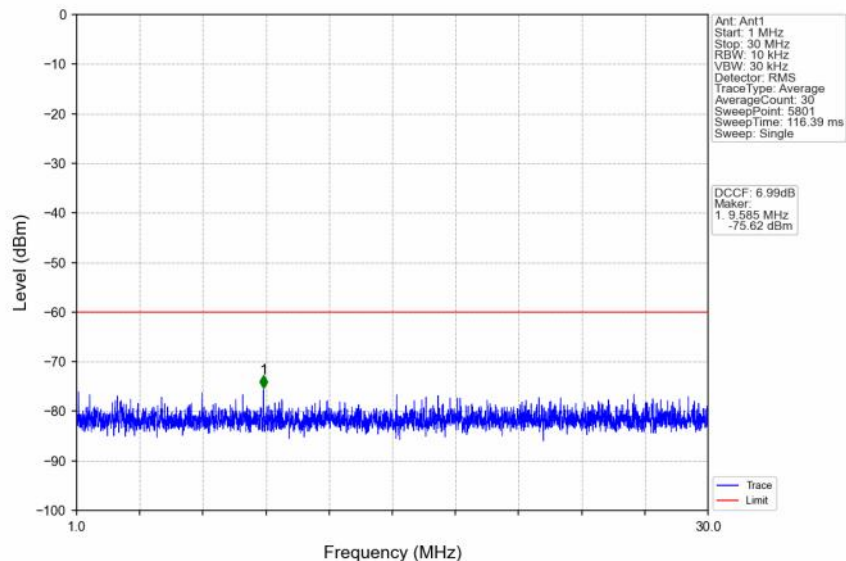
n48_30kHz_SISO_NTNV_10MHz_CP-OFDM QPSK_3555MHz_Inner_1RB_Left
