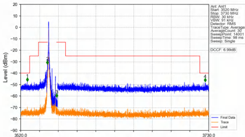
n48_30kHz_SISO_NTNV_10MHz_CP-OFDM QPSK_3555MHz_Inner_1RB_Left
