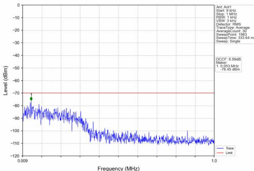
n48_30kHz_SISO_NTNV_20MHz_CP-OFDM QPSK_3690MHz_Inner_1RB_Right
