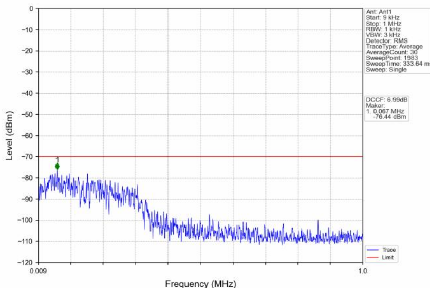
n48_30kHz_SISO_NTNV_10MHz_CP-OFDM QPSK_3555MHz_Edge_1RB_Left
