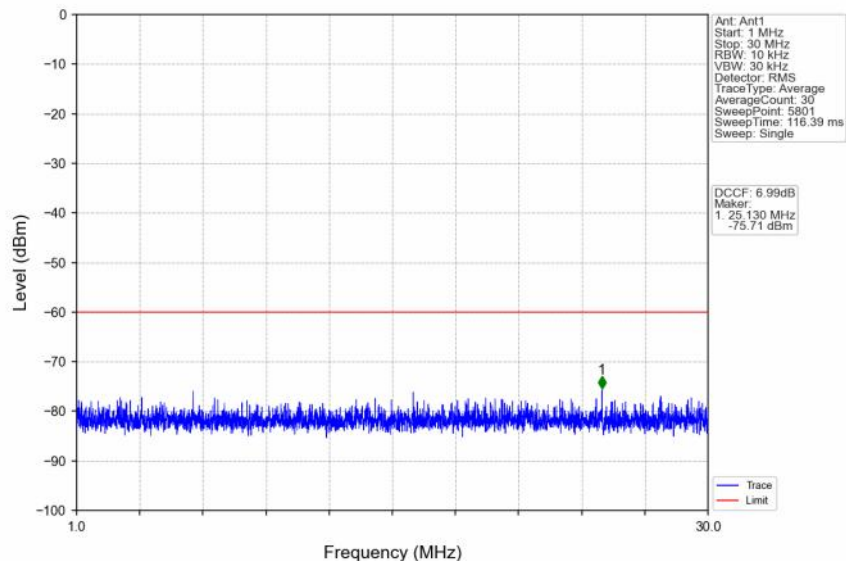
n48_30kHz_SISO_NTNV_10MHz_CP-OFDM QPSK_3555MHz_Edge_1RB_Left
