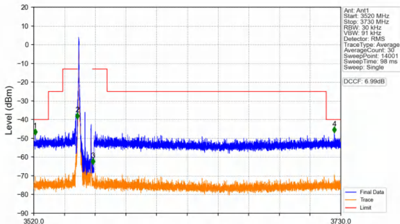
n48_30kHz_SISO_NTNV_10MHz_CP-OFDM QPSK_3555MHz_Edge_1RB_Left
