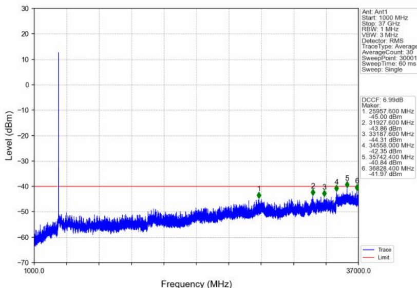
n48_30kHz_SISO_NTNV_20MHz_DFT-s-OFDM QPSK_3690MHz_Inner_1RB_Right
