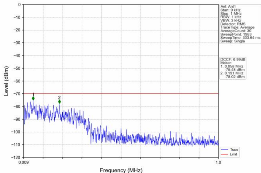
n48_30kHz_SISO_NTNV_20MHz_CP-OFDM QPSK_3624.99MHz_Edge_1RB_Left
