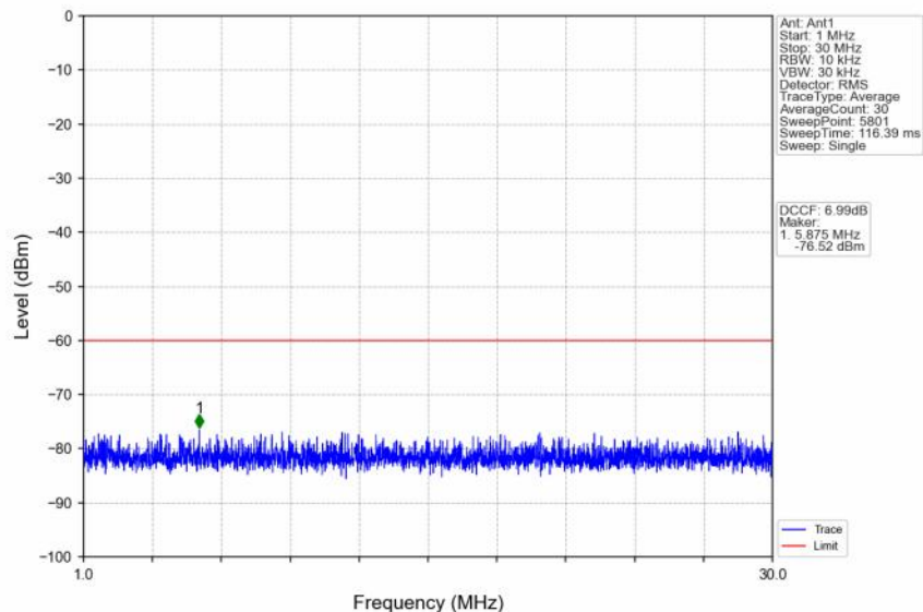
n48_30kHz_SISO_NTNV_20MHz_CP-OFDM QPSK_3690MHz_Inner_1RB_Right
