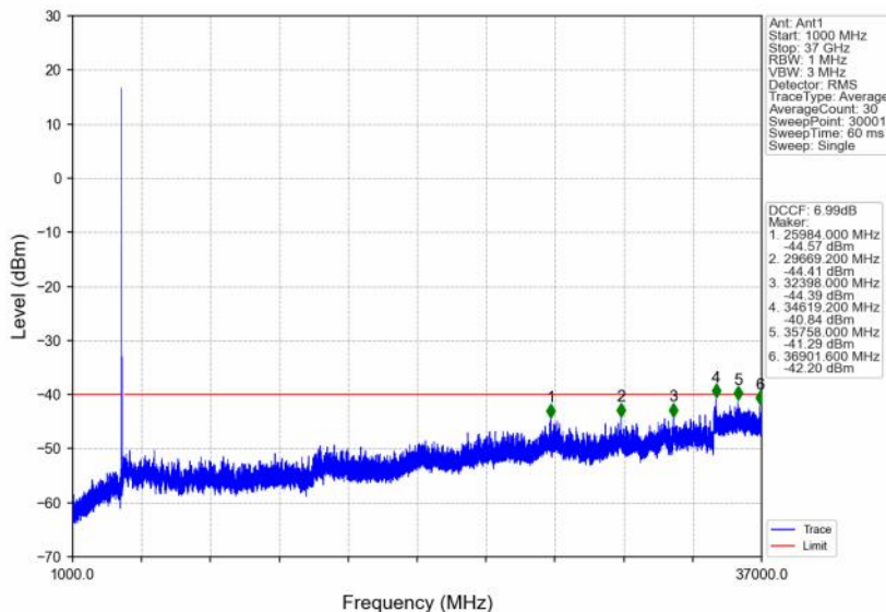
n48_30kHz_SISO_NTNV_20MHz_CP-OFDM QPSK_3624.99MHz_Edge_1RB_Left
