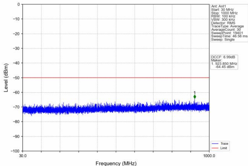
n48_30kHz_SISO_NTNV_20MHz_DFT-s-OFDM QPSK_3560.01MHz_Inner_1RB_Left
