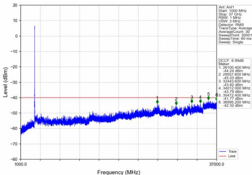
n48_30kHz_SISO_NTNV_20MHz_DFT-s-OFDM QPSK_3560.01MHz_Inner_1RB_Left
