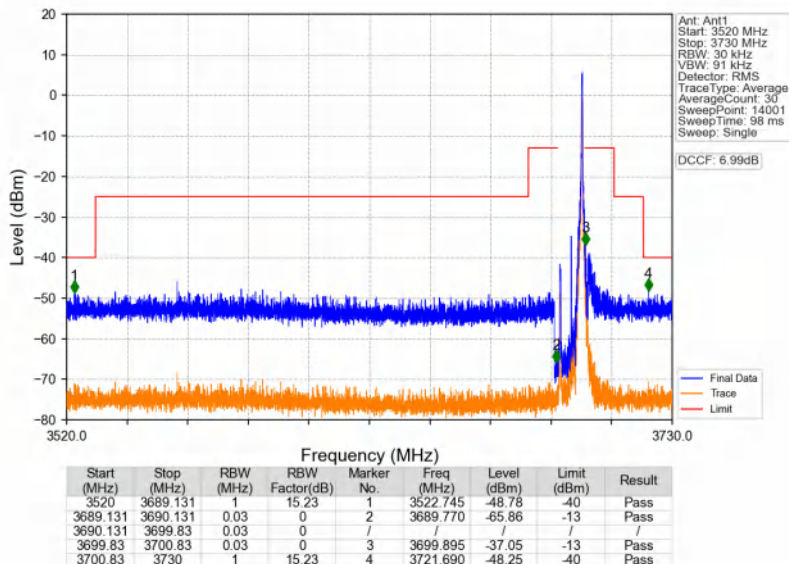
n48_30kHz_SISO_NTV_10MHz_CP-OFDM QPSK_3694.98MHz_Inner_1RB_Right
