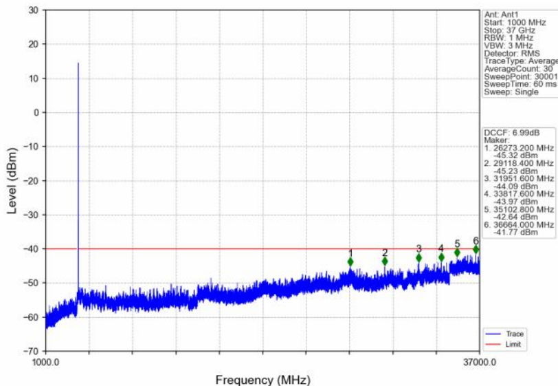
n48_30kHz_SISO_NTNV_10MHz_DFT-s-OFDM QPSK_3555MHz_Edge_1RB_Left
