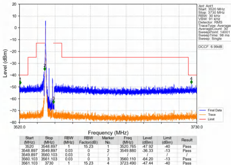
n48_30kHz_SISO_NTNV_10MHz_DFT-s-OFDM QPSK_3555MHz_Edge_1RB_Left
