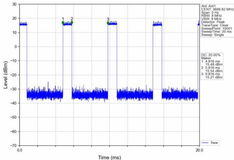
n48_30kHz_SISO_NTNV_20MHz_DFT-s-OFDM PI/2 BPSK_3690MHz_Inner_Full
