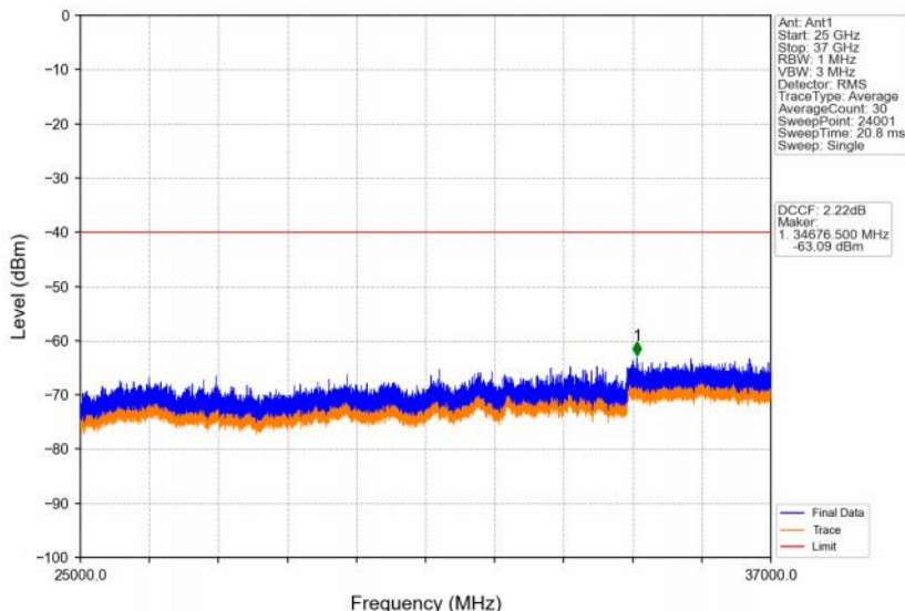
Band48_15MHz_QPSK_HCH_3692.5MHz_RB_1_74_NTNV
