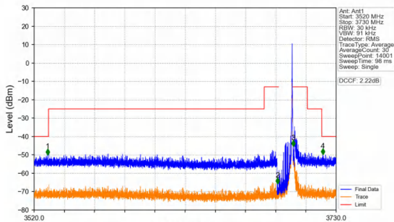
Band48_10MHz_64QAM_HCH_3695MHz_RB_1_49_NTNV
