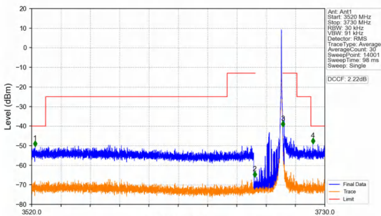
Band48_20MHz_64QAM_HCH_3690MHz_RB_1_99_NTNV
