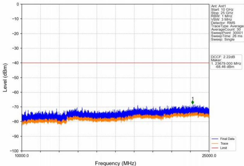
Band48_20MHz_QPSK_LCH_3560MHz_RB_1_0_NTNV
