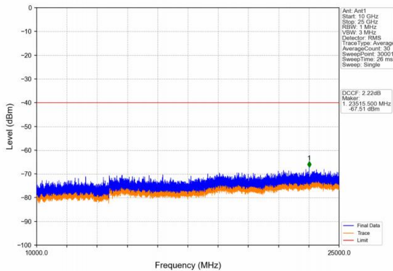
Band48_10MHz_256QAM_LCH_3555MHz_RB_1_0_NTNV
