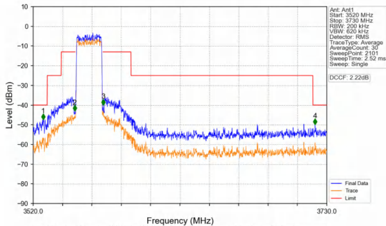
Band48_20MHz_256QAM_LCH_3560MHz_RB_100_0_NTNV
