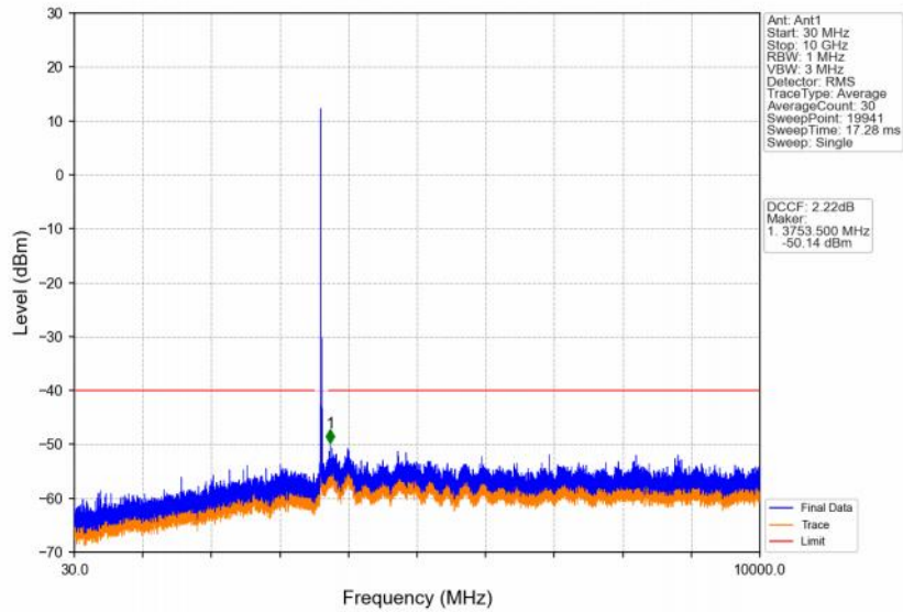
Band48_20MHz_256QAM_MCH_3625MHz_RB_1_0_NTNV
