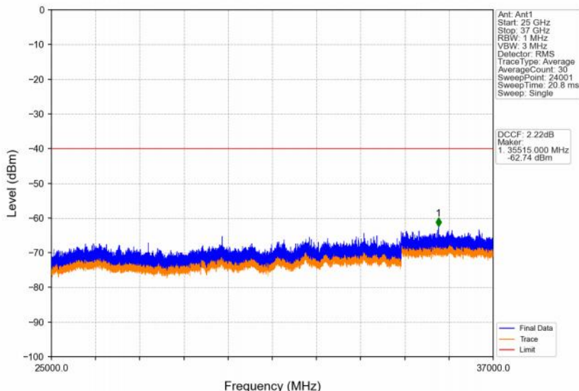
Band48_20MHz_64QAM_HCH_3690MHz_RB_1_99_NTNV
