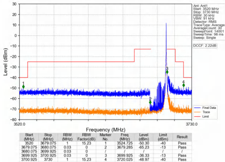
Band48_20MHz_QPSK_HCH_3690MHz_RB_1_99_NTNV
