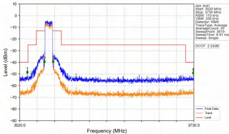
Band48_10MHz_256QAM_LCH_3555MHz_RB_50_0_NTNV
