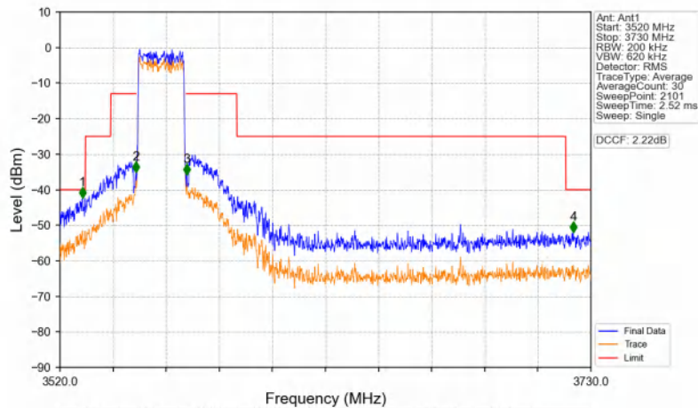
Band48_20MHz_16QAM_LCH_3560MHz_RB_100_0_NTNV
