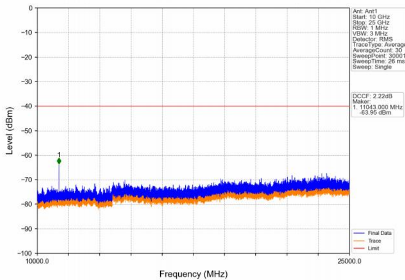
Band48_20MHz_QPSK_HCH_3690MHz_RB_1_0_NTNV
