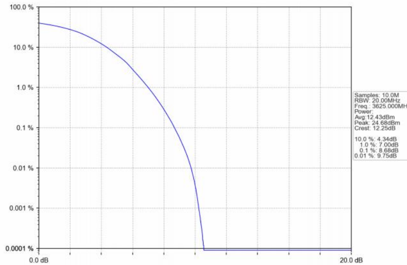
Band48_20MHz_16QAM_MCH_3625MHz_RB_100_0_NTNV
