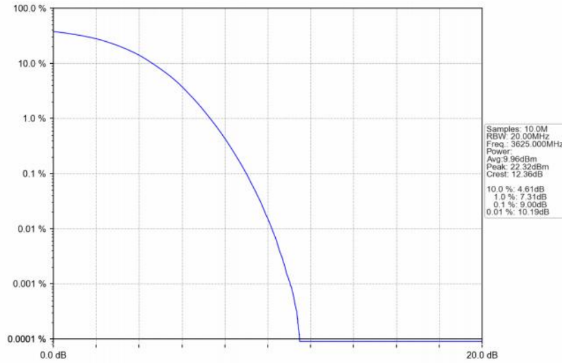
Band48_20MHz_256QAM_MCH_3625MHz_RB_100_0_NTNV
