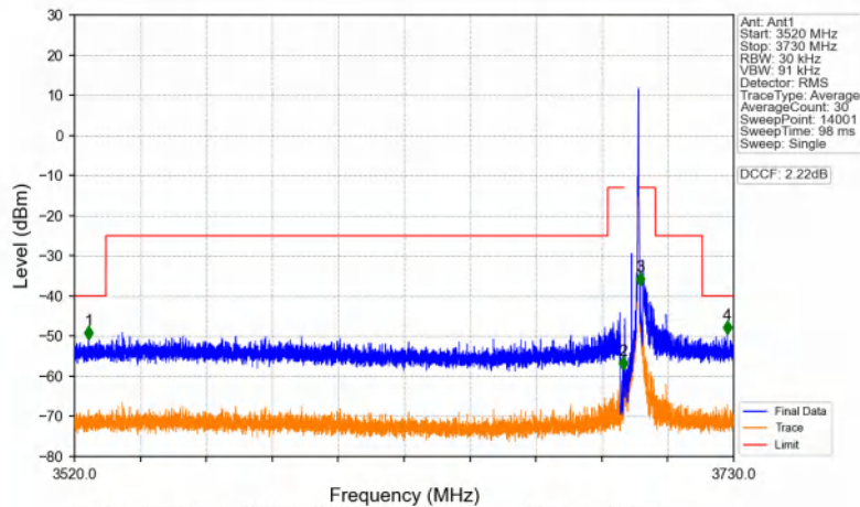
Band48_5MHz_QPSK_HCH_3697.5MHz_RB_1_24_NTNV
