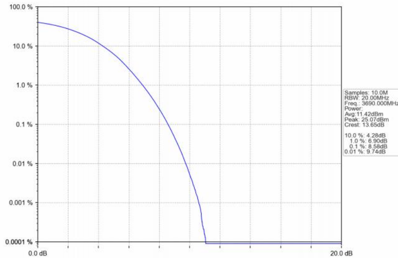
Band48_20MHz_256QAM_HCH_3690MHz_RB_100_0_NTNV
