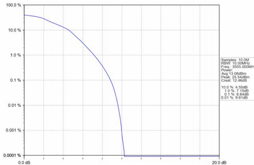
Band48_10MHz_16QAM_LCH_3555MHz_RB_50_0_NTNV
