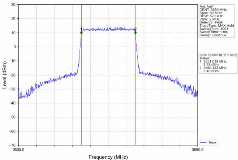
Band48_20MHz_256QAM_LCH_3560MHz_RB_100_0_NTNV
