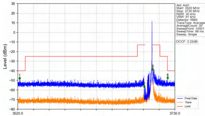
Band48_10MHz_QPSK_HCH_3695MHz_RB_1_49_NTNV
