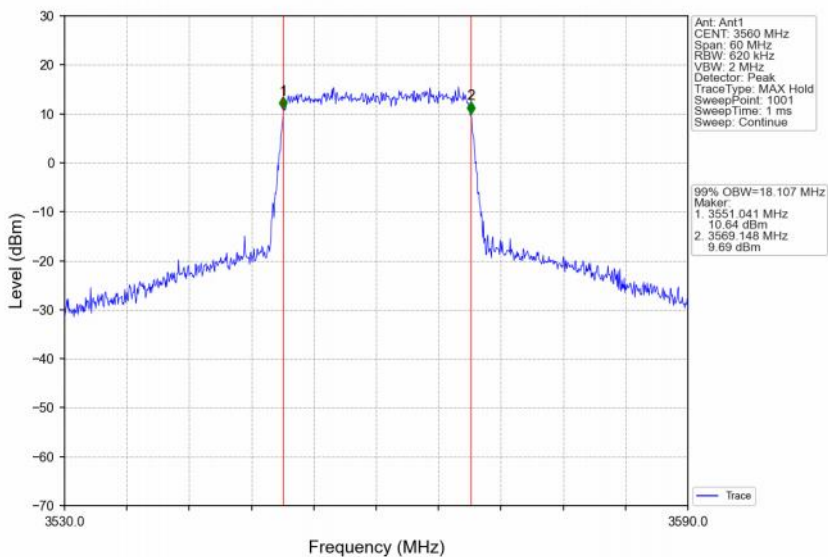
Band48_20MHz_16QAM_LCH_3560MHz_RB_100_0_NTNV
