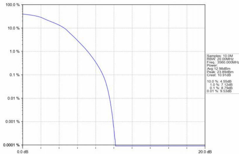
Band48_20MHz_16QAM_LCH_3560MHz_RB_100_0_NTNV
