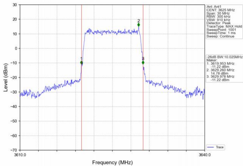
Band48_10MHz_QPSK_MCH_3625MHz_RB_50_0_NTNV
