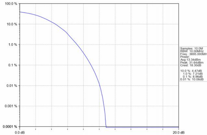
Band48_10MHz_QPSK_HCH_3695MHz_RB_50_0_NTNV
