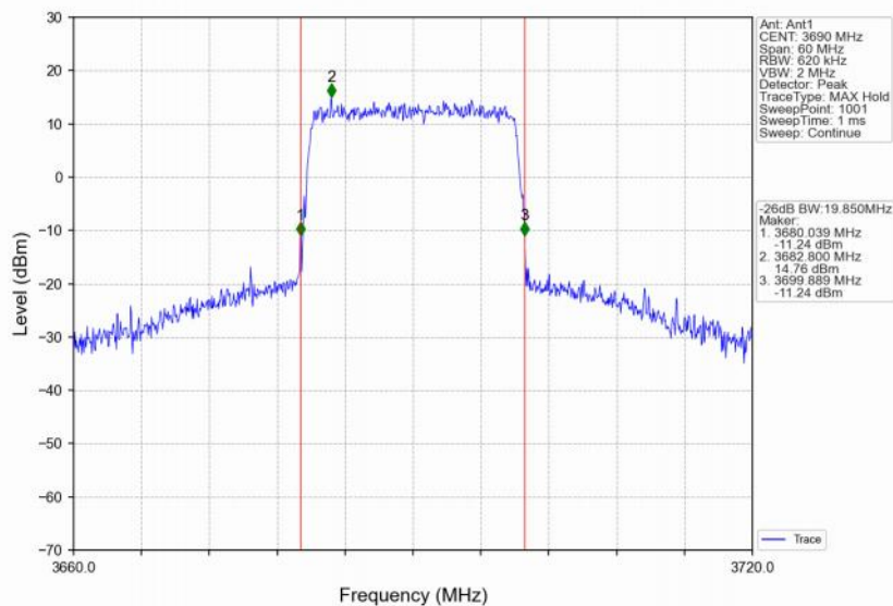
Band48_20MHz_16QAM_HCH_3690MHz_RB_100_0_NTNV
