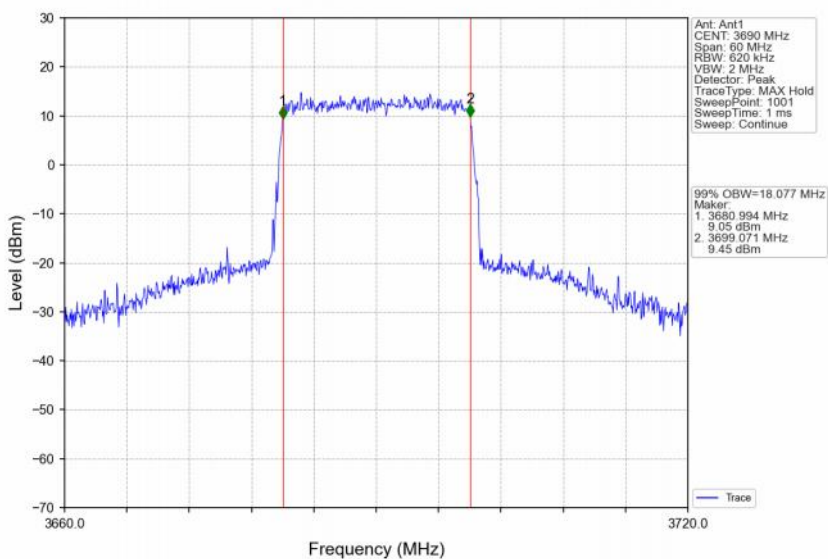
Band48_20MHz_16QAM_HCH_3690MHz_RB_100_0_NTNV
