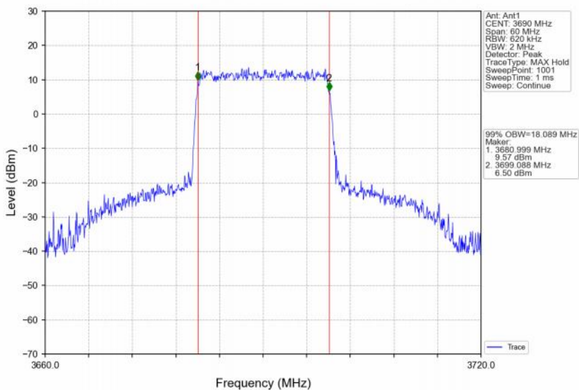
Band48_20MHz_256QAM_HCH_3690MHz_RB_100_0_NTNV
