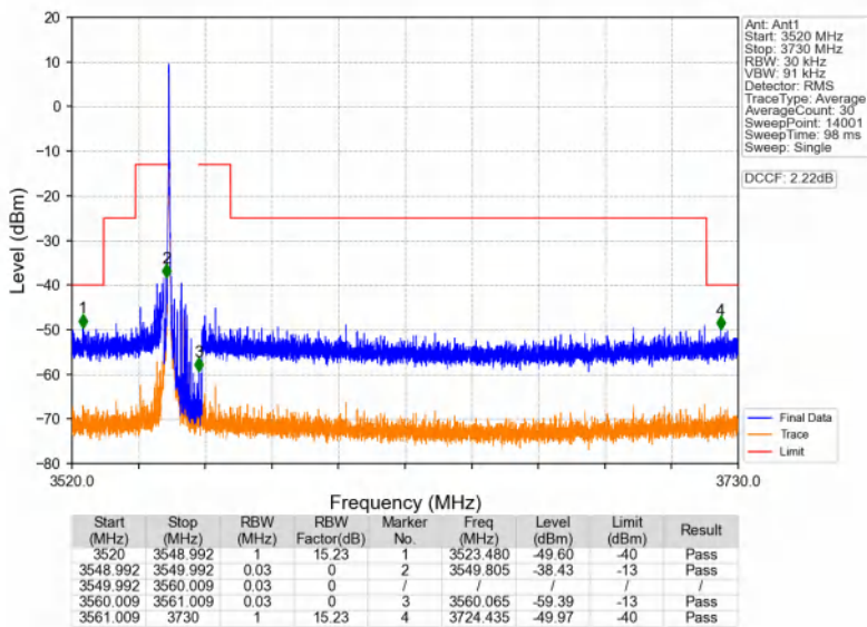
Band48_10MHz_16QAM_LCH_3555MHz_RB_1_0_NTNV
