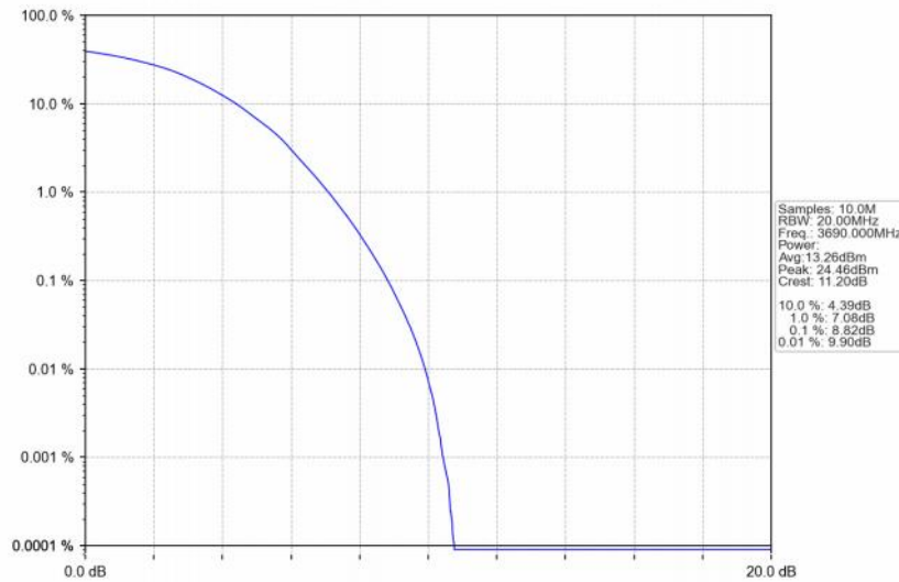
Band48_20MHz_QPSK_HCH_3690MHz_RB_100_0_NTNV
