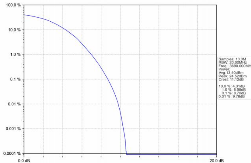
Band48_20MHz_16QAM_HCH_3690MHz_RB_100_0_NTNV
