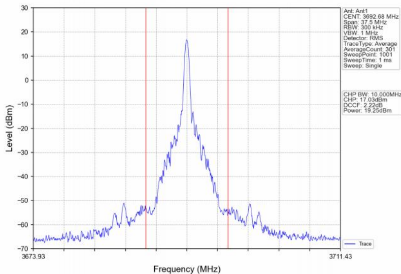
Band48_15MHz_QPSK_HCH_3692.5MHz_RB_1_38_NTNV
