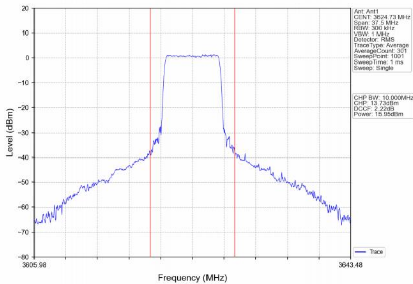
Band48_15MHz_64QAM_MCH_3625MHz_RB_36_18_NTNV
