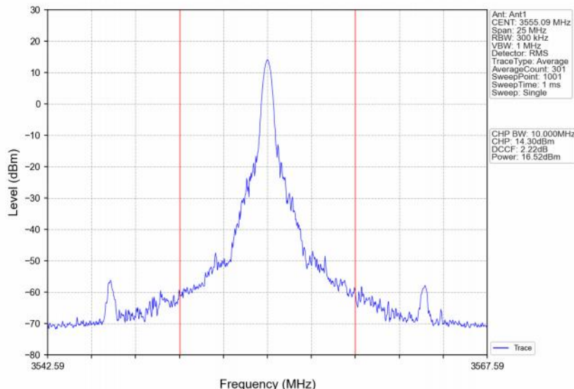
Band48_10MHz_16QAM_LCH_3555MHz_RB_1_49_NTNV
