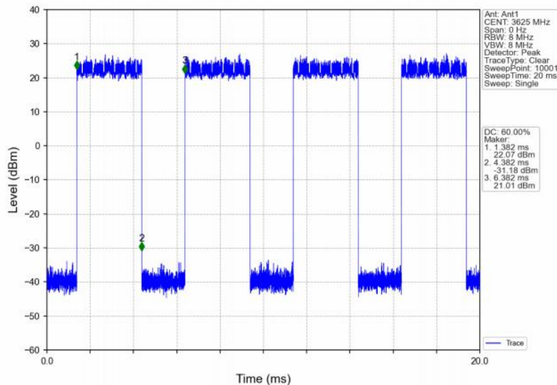
Band48_20MHz_256QAM_MCH_3625MHz_RB_50_50_NTNV
