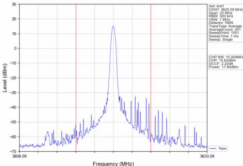
Band48_10MHz_16QAM_MCH_3625MHz_RB_1_25_NTNV
