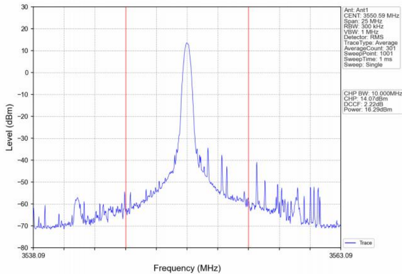
Band48_10MHz_16QAM_LCH_3555MHz_RB_1_0_NTNV
