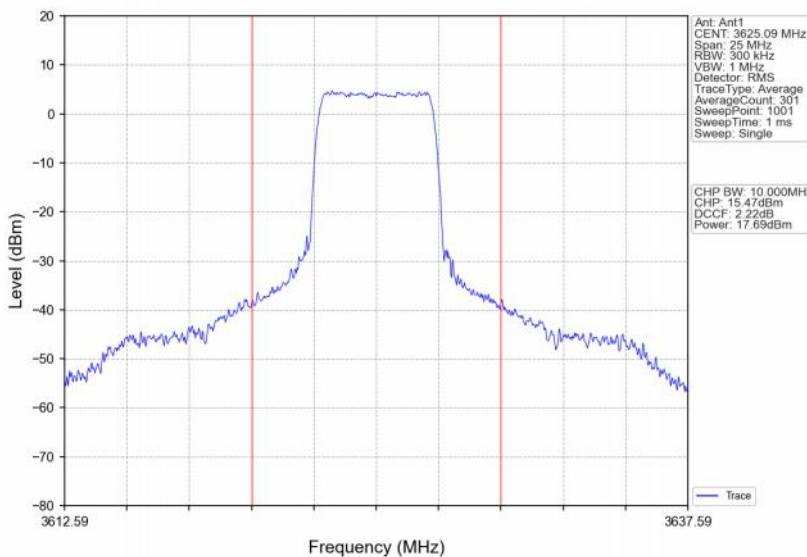
Band48_10MHz_QPSK_MCH_3625MHz_RB_25_13_NTNV
