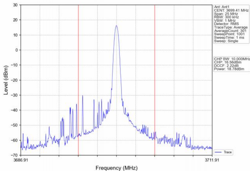
Band48_10MHz_16QAM_HCH_3695MHz_RB_1_49_NTNV
