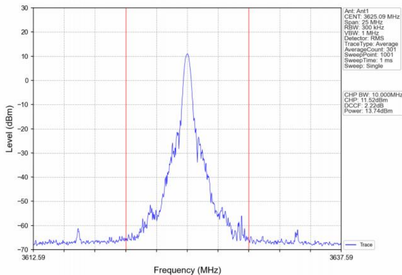
Band48_10MHz_256QAM_MCH_3625MHz_RB_1_25_NTNV
