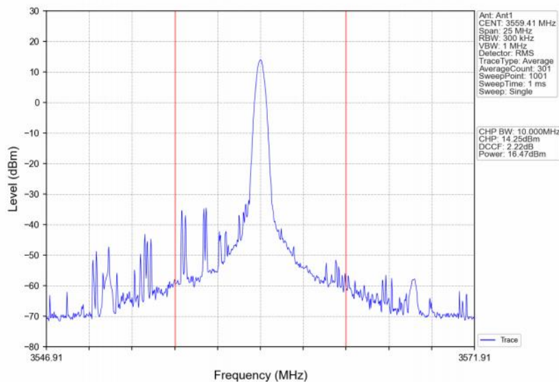
Band48_10MHz_16QAM_LCH_3555MHz_RB_1_49_NTNV
