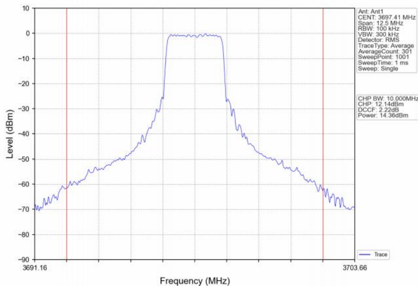
Band48_5MHz_256QAM_HCH_3697.5MHz_RB_12_6_NTNV
