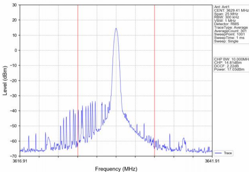
Band48_10MHz_64QAM_MCH_3625MHz_RB_1_49_NTNV
