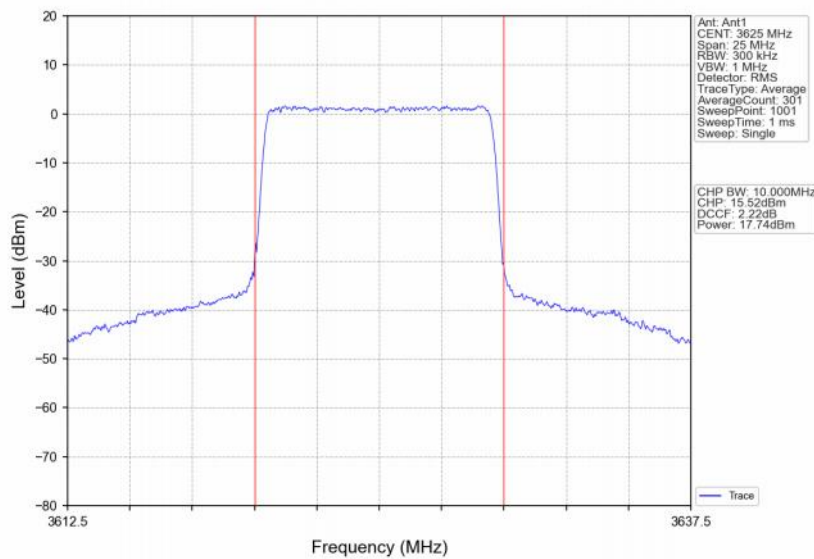
Band48_10MHz_QPSK_MCH_3625MHz_RB_50_0_NTNV
