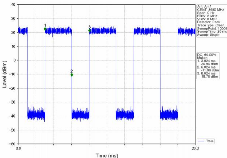
Band48_20MHz_256QAM_HCH_3690MHz_RB_100_0_NTNV
