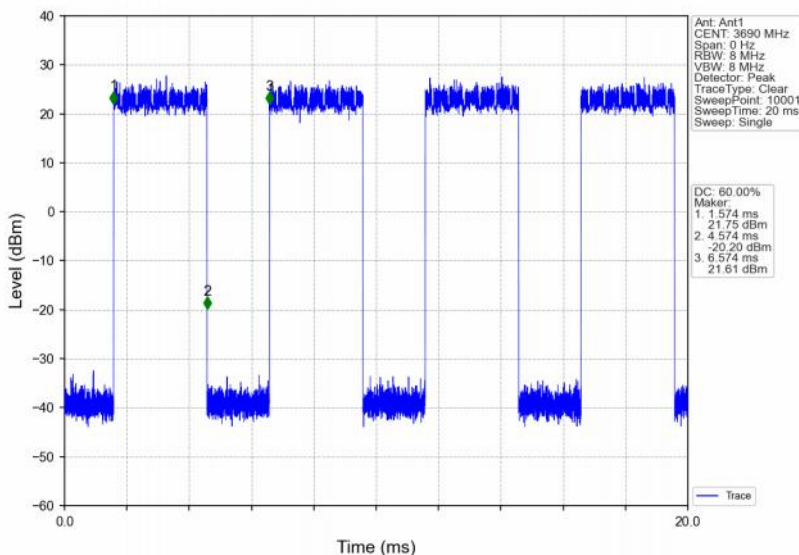
Band48_20MHz_256QAM_HCH_3690MHz_RB_50_25_NTNV
