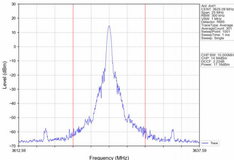
Band48_10MHz_64QAM_MCH_3625MHz_RB_1_49_NTNV
