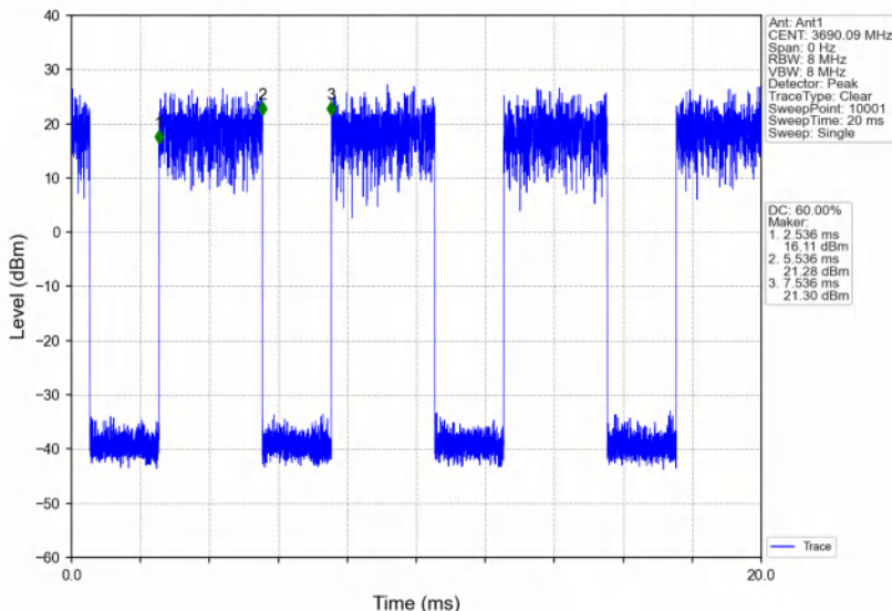
Band48_20MHz_256QAM_HCH_3690MHz_RB_1_99_NTNV
