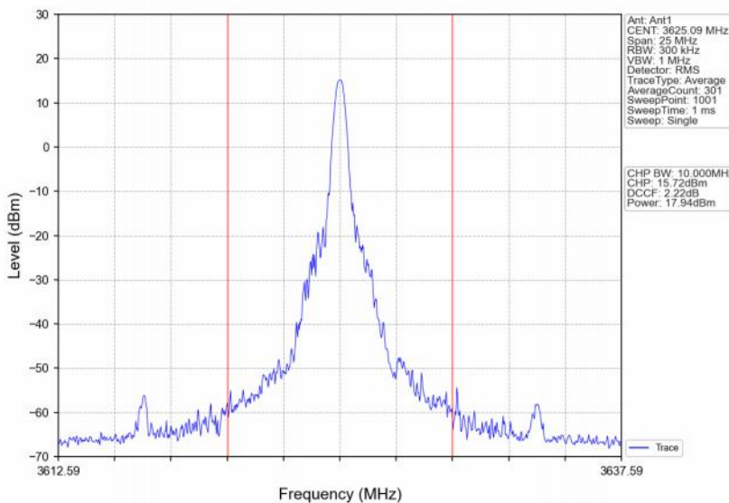
Band48_10MHz_16QAM_MCH_3625MHz_RB_1_25_NTNV
