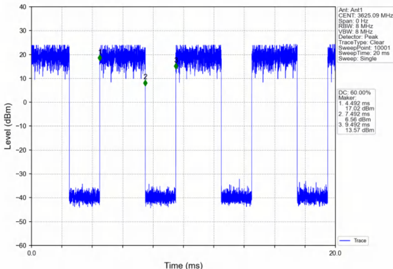
Band48_20MHz_QPSK_MCH_3625MHz_RB_1_99_NTNV
