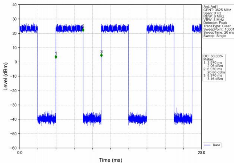
Band48_20MHz_64QAM_MCH_3625MHz_RB_50_25_NTNV
