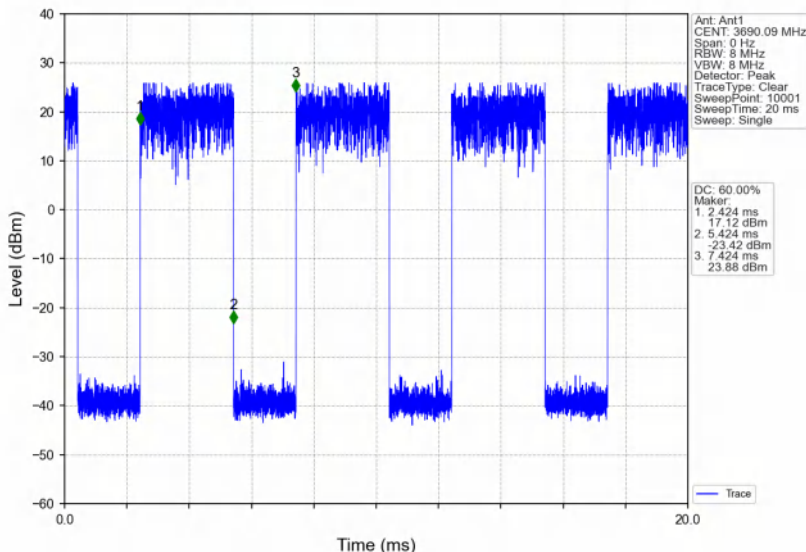
Band48_20MHz_16QAM_HCH_3690MHz_RB_1_99_NTNV
