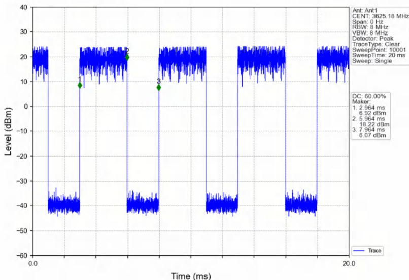
Band48_15MHz_QPSK_MCH_3625MHz_RB_1_74_NTNV
