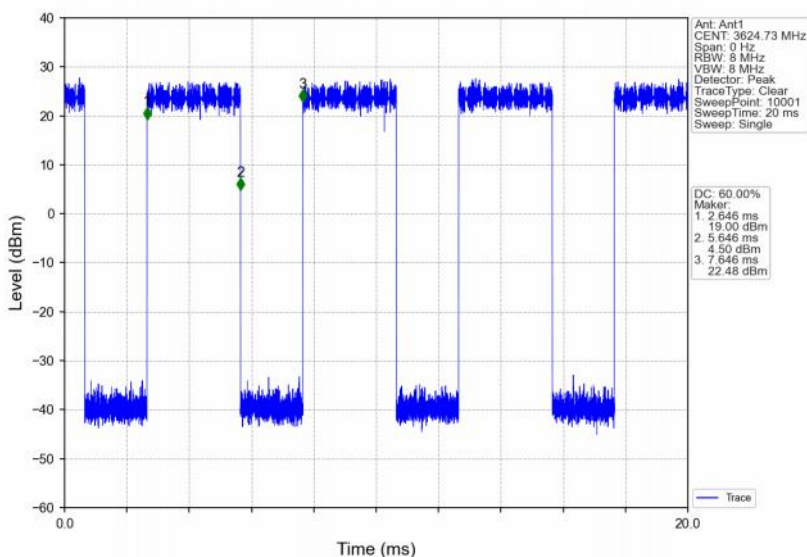
Band48_15MHz_64QAM_MCH_3625MHz_RB_36_18_NTNV
