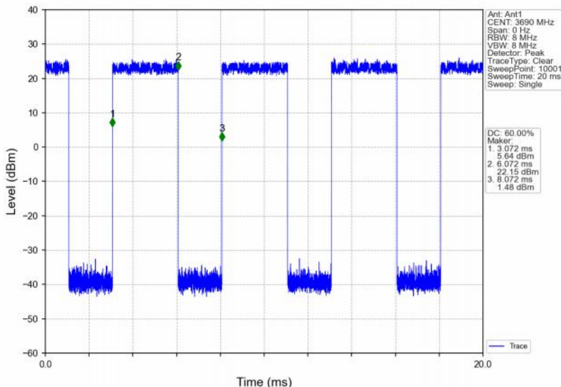
Band48_20MHz_QPSK_HCH_3690MHz_RB_50_50_NTNV
