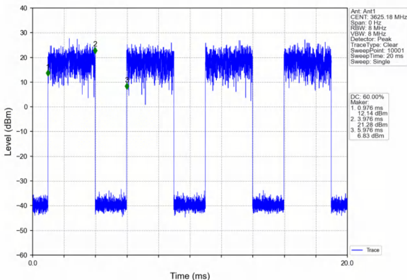
Band48_15MHz_256QAM_MCH_3625MHz_RB_1_38_NTNV
