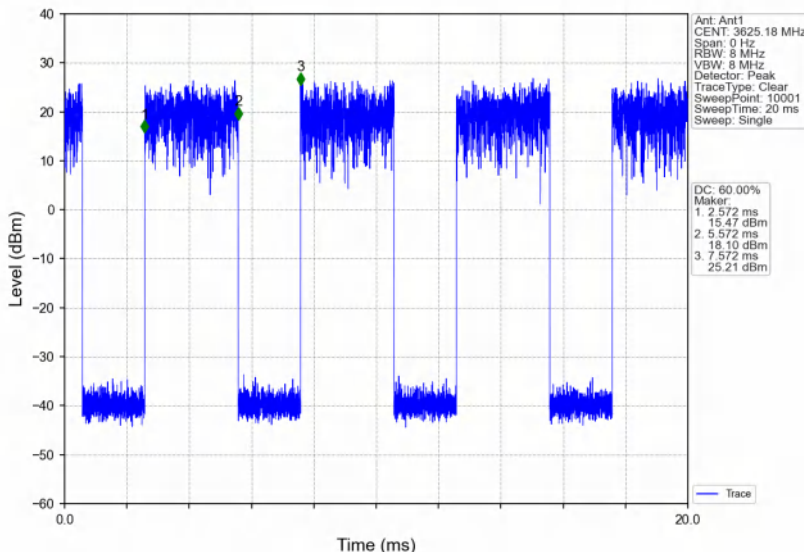
Band48_15MHz_64QAM_MCH_3625MHz_RB_1_74_NTNV
