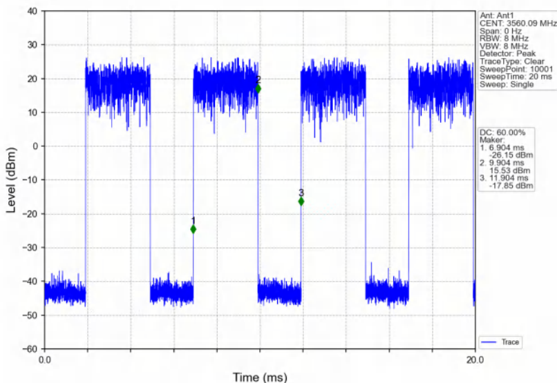
Band48_20MHz_64QAM_LCH_3560MHz_RB_1_50_NTNV
