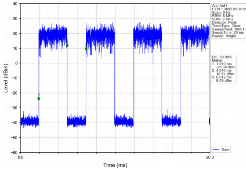
Band48_15MHz_256QAM_HCH_3692.5MHz_RB_1_74_NTNV
