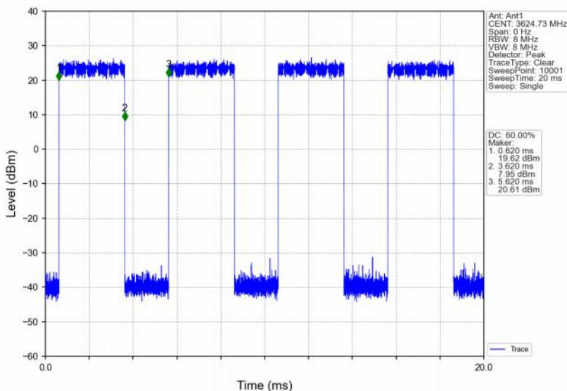
Band48_15MHz_QPSK_MCH_3625MHz_RB_36_18_NTNV
