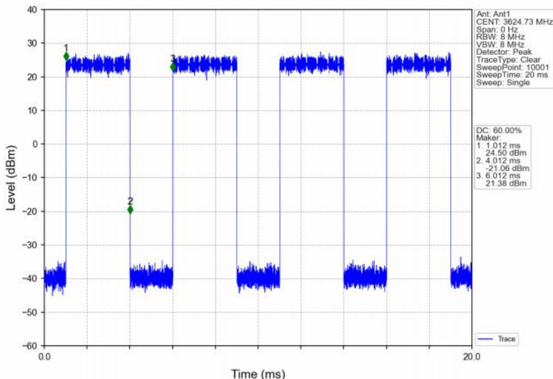
Band48_15MHz_16QAM_MCH_3625MHz_RB_36_39_NTNV
