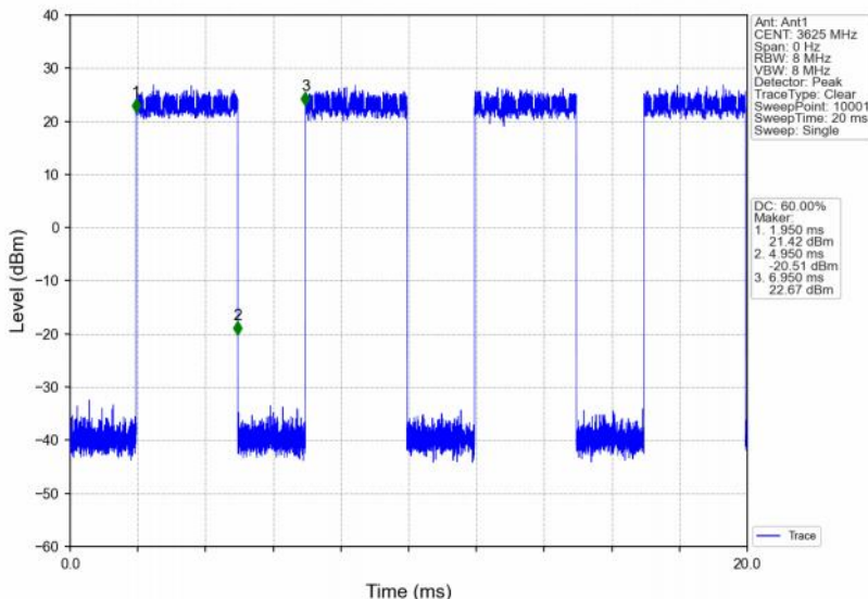
Band48_20MHz_16QAM_MCH_3625MHz_RB_50_50_NTNV
