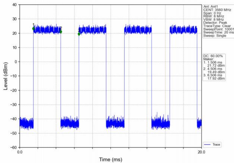
Band48_20MHz_256QAM_LCH_3560MHz_RB_50_25_NTNV
