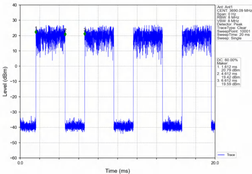
Band48_20MHz_64QAM_HCH_3690MHz_RB_1_50_NTNV
