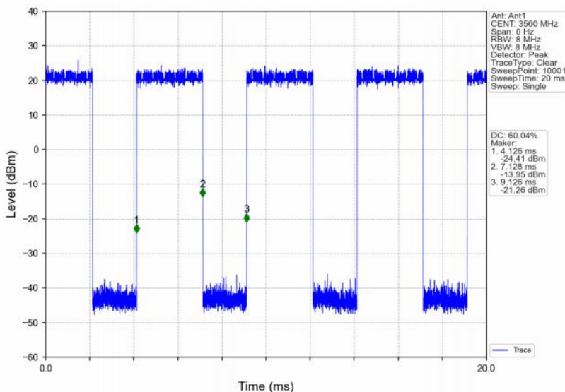
Band48_20MHz_16QAM_LCH_3560MHz_RB_100_0_NTNV
