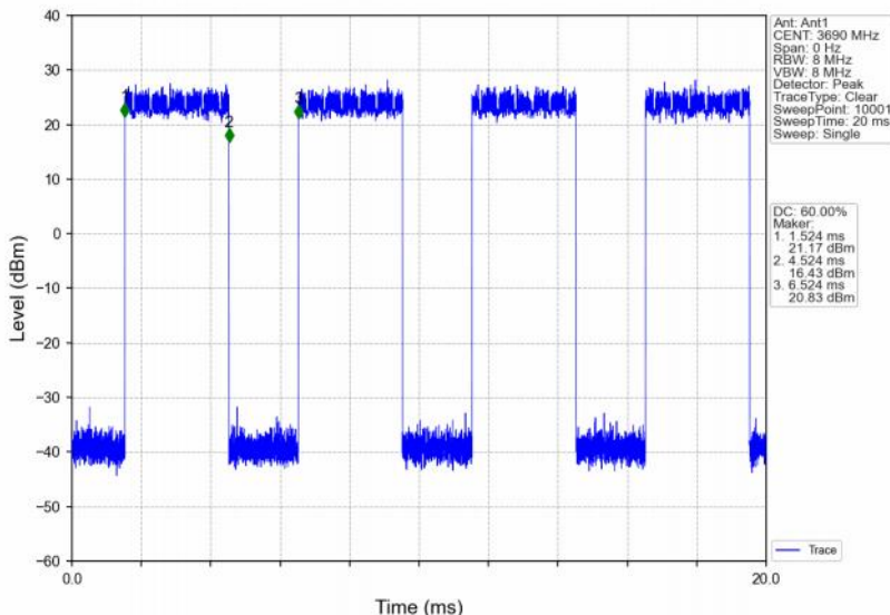
Band48_20MHz_64QAM_HCH_3690MHz_RB_50_50_NTNV
