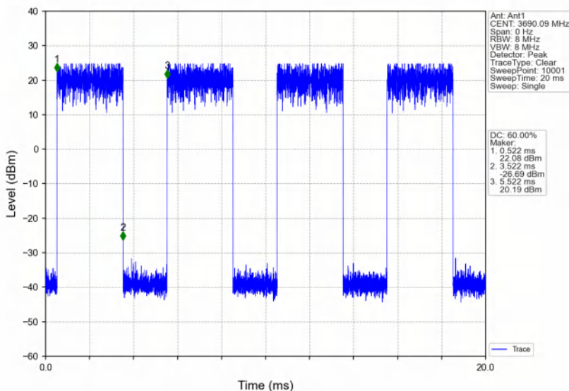
Band48_20MHz_QPSK_HCH_3690MHz_RB_1_50_NTNV
