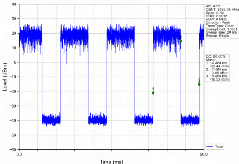
Band48_20MHz_64QAM_MCH_3625MHz_RB_1_99_NTNV
