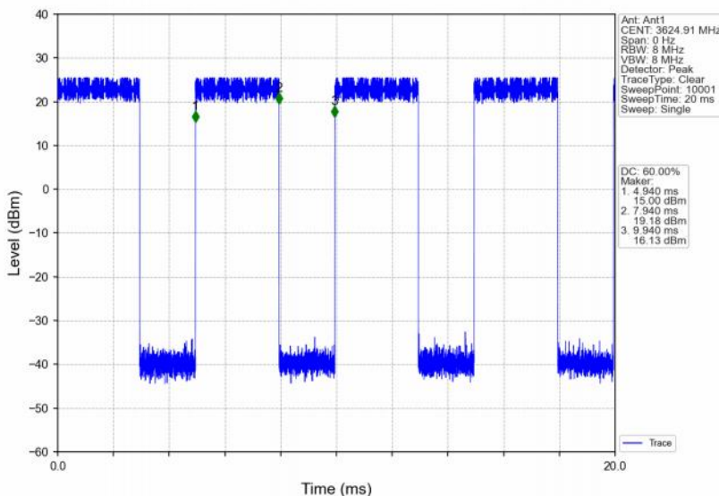
Band48_5MHz_QPSK_MCH_3625MHz_RB_12_6_NTNV
