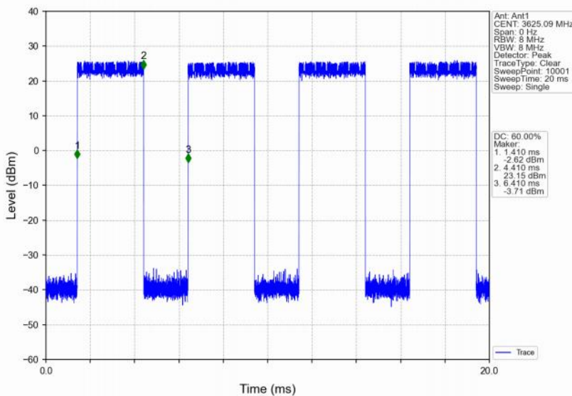
Band48_10MHz_QPSK_MCH_3625MHz_RB_25_13_NTNV
