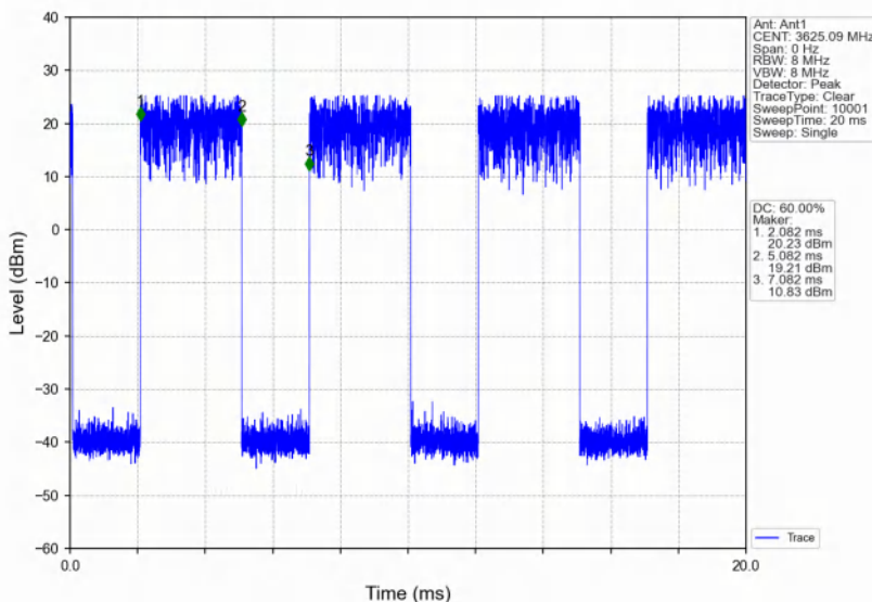
Band48_10MHz_16QAM_MCH_3625MHz_RB_1_25_NTNV
