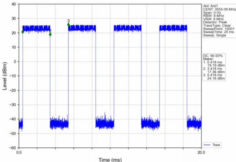
Band48_10MHz_QPSK_LCH_3555MHz_RB_25_25_NTNV
