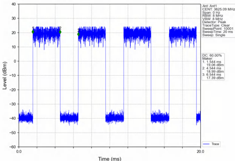
Band48_10MHz_QPSK_MCH_3625MHz_RB_1_49_NTNV
