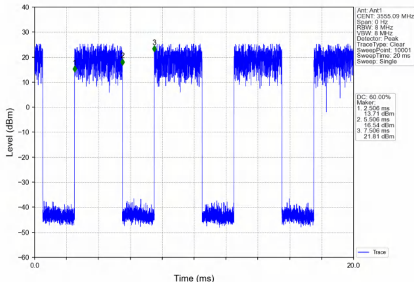
Band48_10MHz_16QAM_LCH_3555MHz_RB_1_49_NTNV
