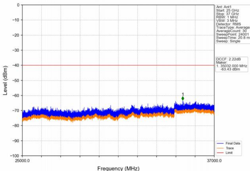
Band48_15MHz_QPSK_MCH_3625MHz_RB_1_0_NTNV
