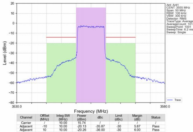
Band48_10MHz_256QAM_LCH_3555MHz_RB_50_0_NTNV
