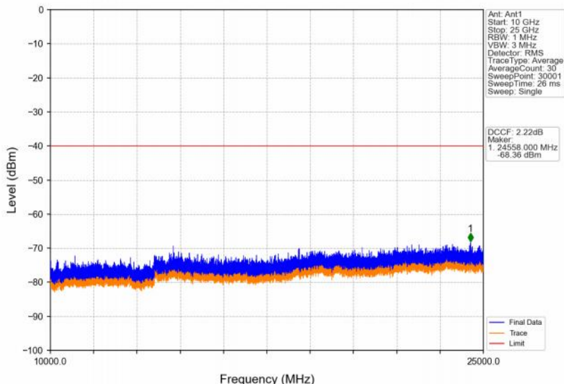
Band48_15MHz_QPSK_MCH_3625MHz_RB_1_0_NTNV
