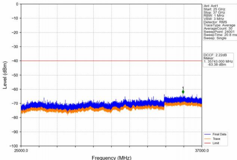
Band48_20MHz_16QAM_HCH_3690MHz_RB_1_0_NTNV
