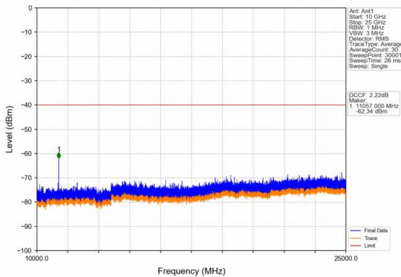
Band48_15MHz_QPSK_HCH_3692.5MHz_RB_1_0_NTNV
