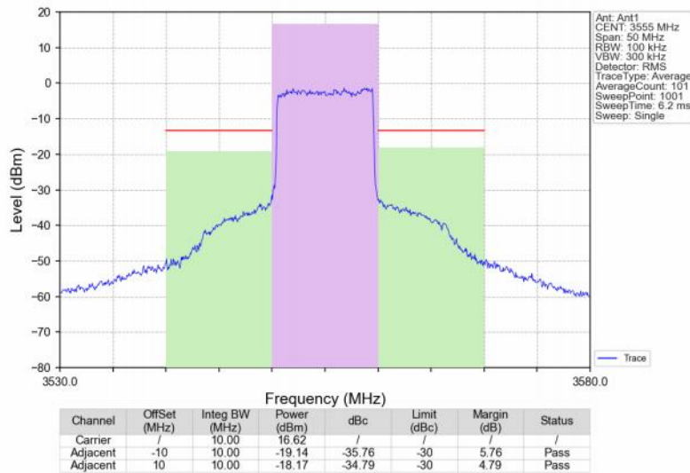
Band48_10MHz_16QAM_LCH_3555MHz_RB_50_0_NTNV
