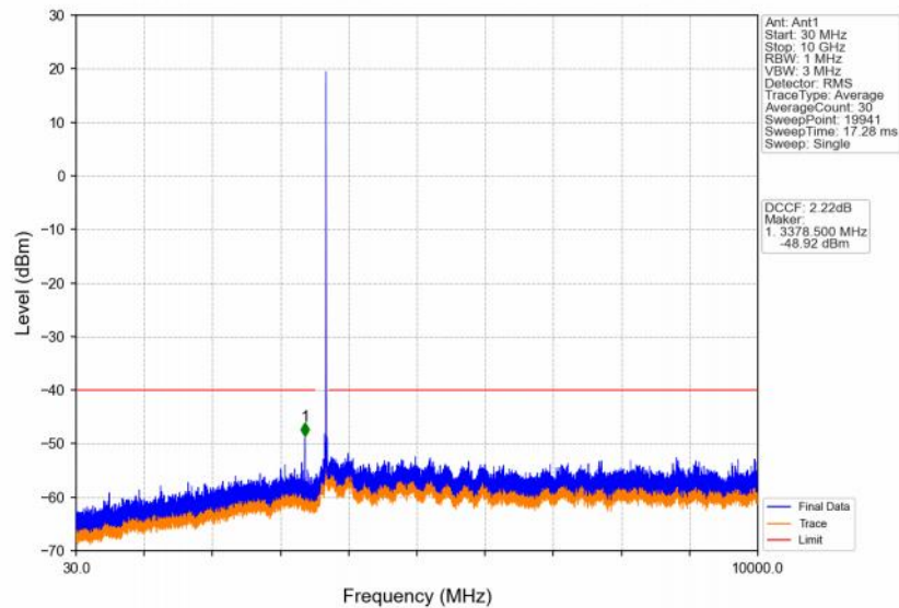
Band48_15MHz_QPSK_HCH_3692.5MHz_RB_1_0_NTNV
