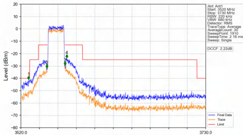
Band48_20MHz_256QAM_LCH_3560MHz_RB_100_0_NTNV
