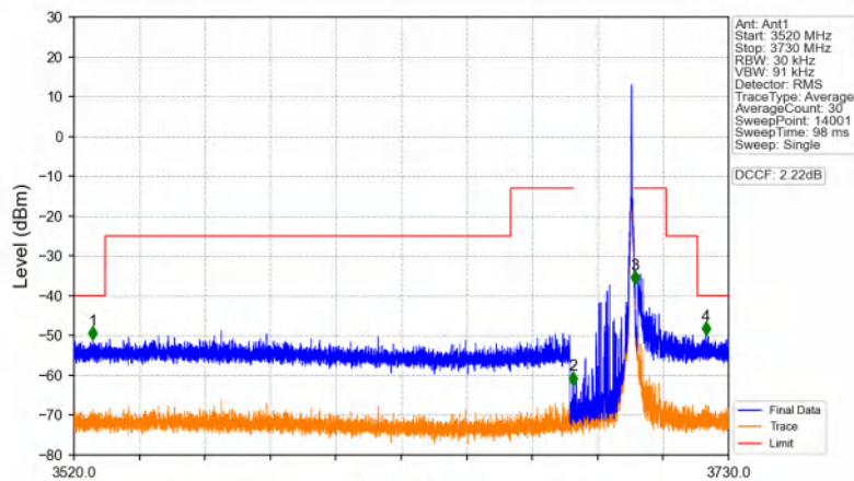
Band48_20MHz_64QAM_HCH_3690MHz_RB_1_99_NTNV
