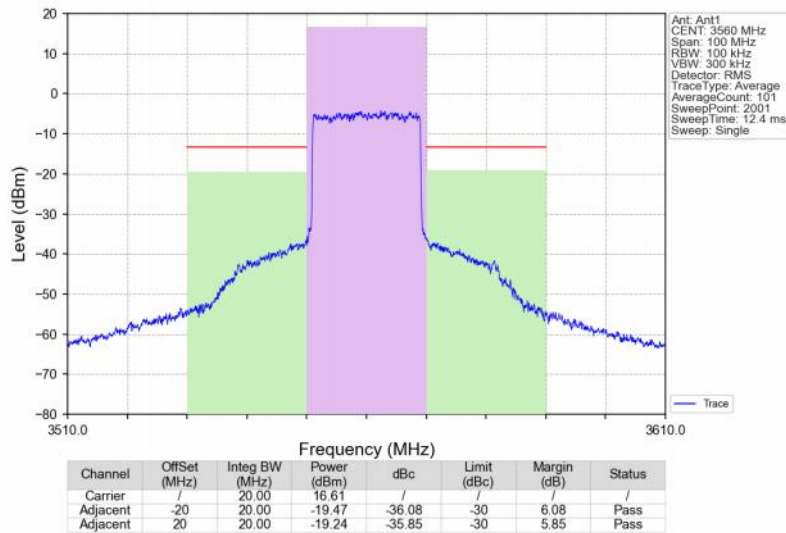
Band48_20MHz_16QAM_LCH_3560MHz_RB_100_0_NTNV
