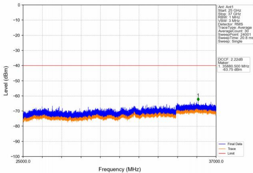
Band48_20MHz_QPSK_MCH_3625MHz_RB_1_0_NTNV
