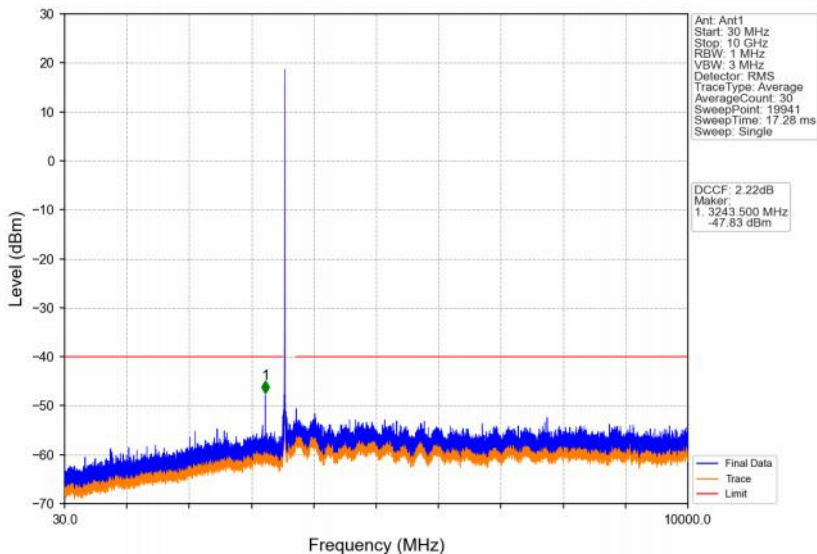
Band48_20MHz_16QAM_LCH_3560MHz_RB_1_0_NTNV
