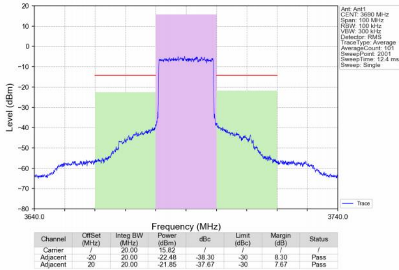
Band48_20MHz_QPSK_HCH_3690MHz_RB_100_0_NTNV
