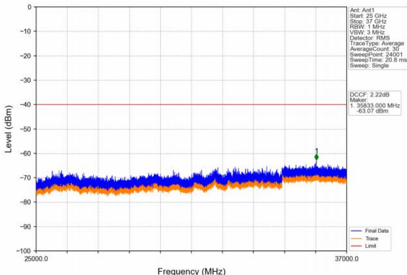
Band48_20MHz_16QAM_LCH_3560MHz_RB_100_0_NTNV
