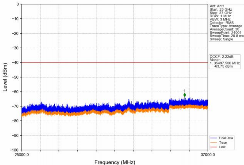
Band48_15MHz_QPSK_HCH_3692.5MHz_RB_1_74_NTNV
