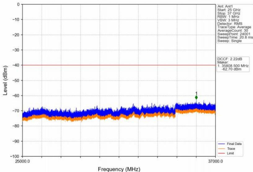
Band48_10MHz_64QAM_HCH_3695MHz_RB_1_49_NTNV
