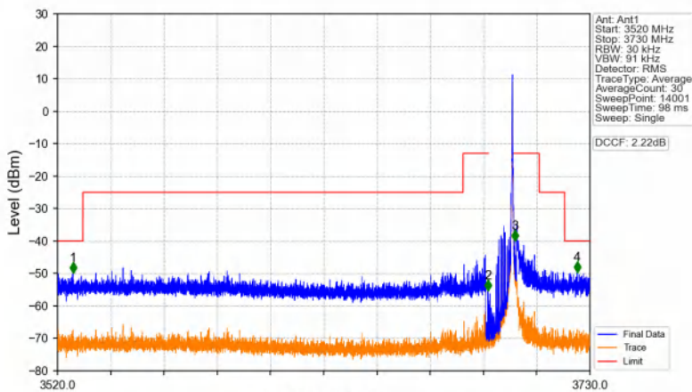
Band48_10MHz_64QAM_HCH_3695MHz_RB_1_49_NTNV
