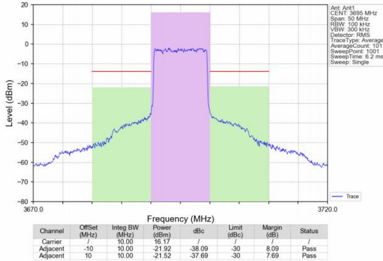
Band48_10MHz_QPSK_HCH_3695MHz_RB_50_0_NTNV
