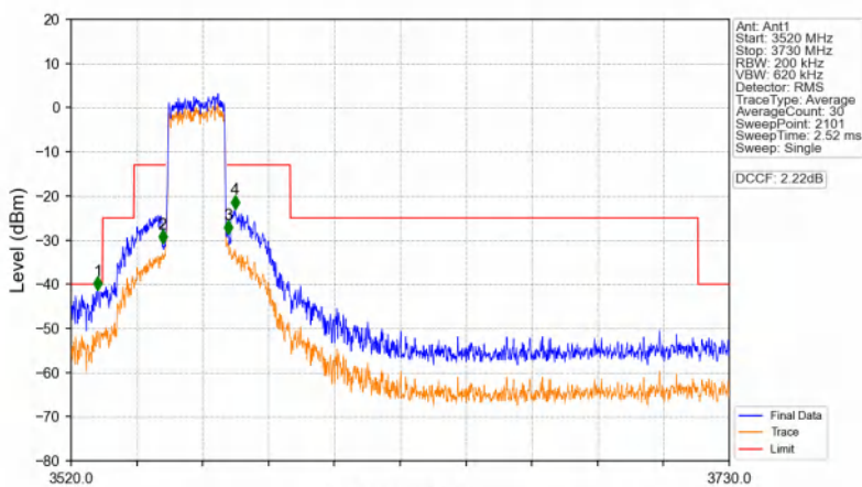
Band48_20MHz_16QAM_LCH_3560MHz_RB_100_0_NTNV
