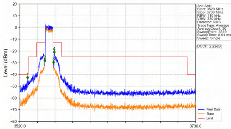
Band48_10MHz_256QAM_LCH_3555MHz_RB_50_0_NTNV
