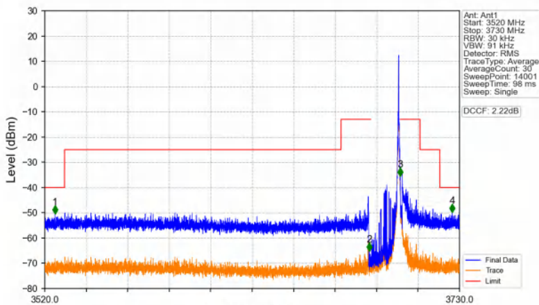
Band48_15MHz_QPSK_HCH_3692.5MHz_RB_1_74_NTNV
