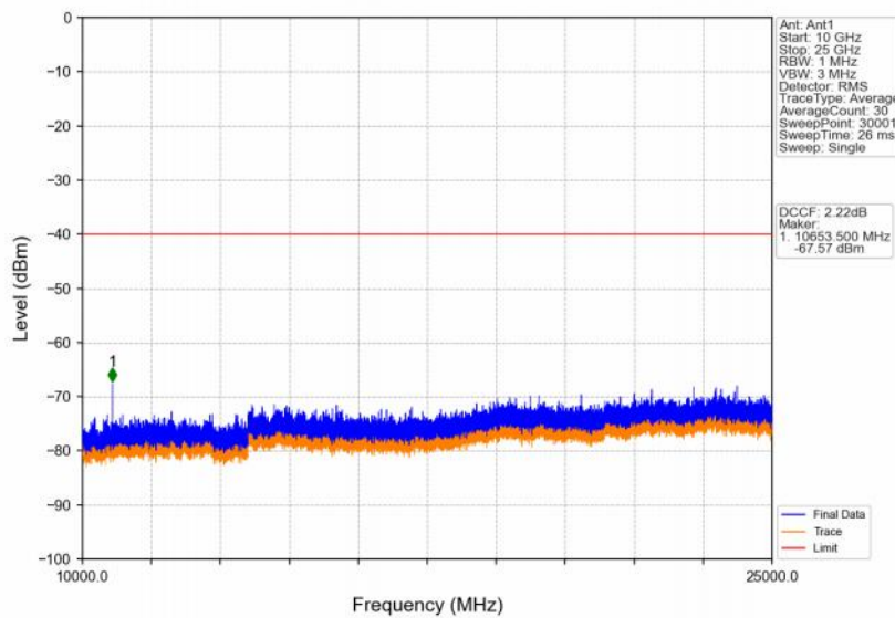
Band48_20MHz_256QAM_LCH_3560MHz_RB_1_0_NTNV
