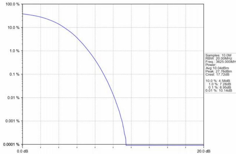
Band48_20MHz_256QAM_MCH_3625MHz_RB_100_0_NTNV
