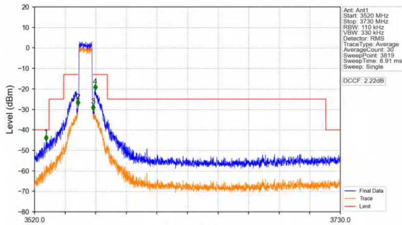
Band48_10MHz_16QAM_LCH_3555MHz_RB_50_0_NTNV
