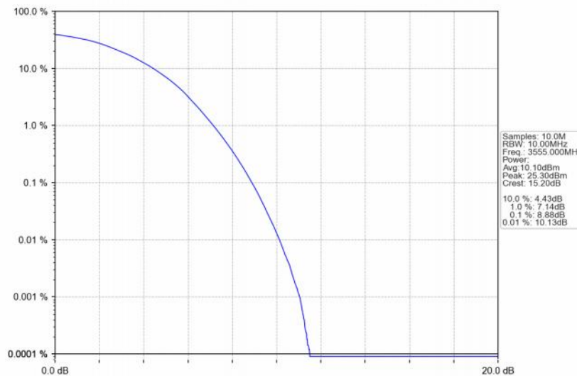
Band48_10MHz_256QAM_LCH_3555MHz_RB_50_0_NTNV
