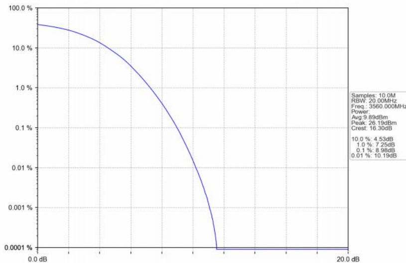
Band48_20MHz_256QAM_LCH_3560MHz_RB_100_0_NTNV
