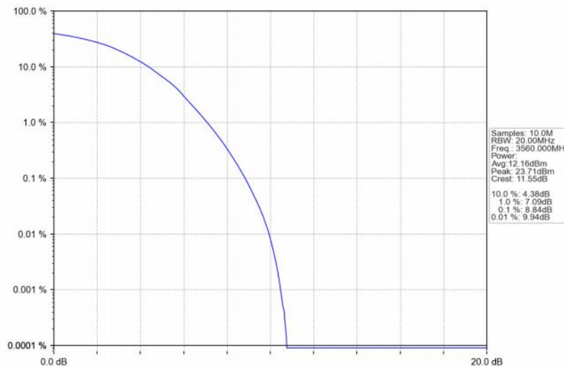
Band48_20MHz_16QAM_LCH_3560MHz_RB_100_0_NTNV
