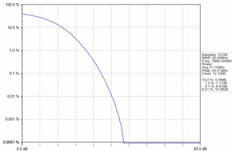
Band48_20MHz_256QAM_HCH_3690MHz_RB_100_0_NTNV
