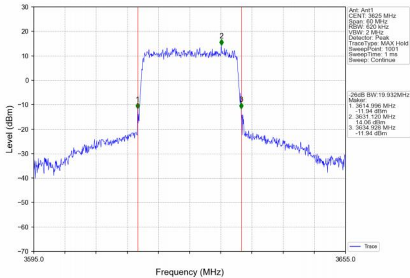
Band48_20MHz_QPSK_MCH_3625MHz_RB_100_0_NTNV
