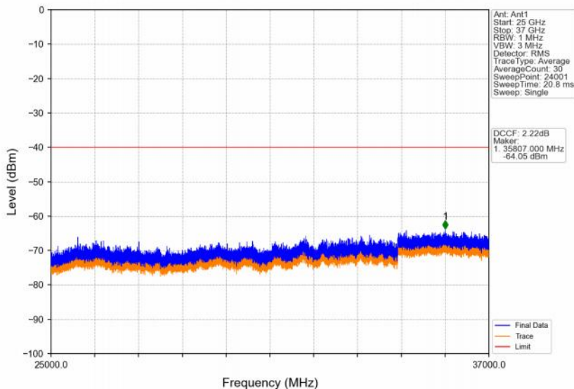
Band48_10MHz_QPSK_HCH_3695MHz_RB_1_49_NTNV
