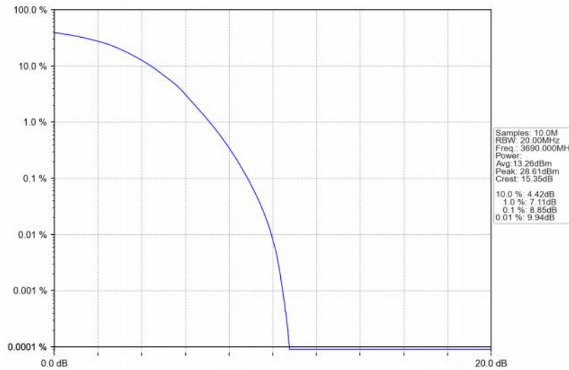
Band48_20MHz_QPSK_HCH_3690MHz_RB_100_0_NTNV
