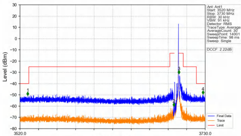
Band48_5MHz_QPSK_HCH_3697.5MHz_RB_1_24_NTNV
