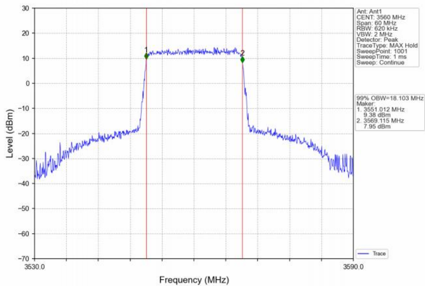
Band48_20MHz_256QAM_LCH_3560MHz_RB_100_0_NTNV
