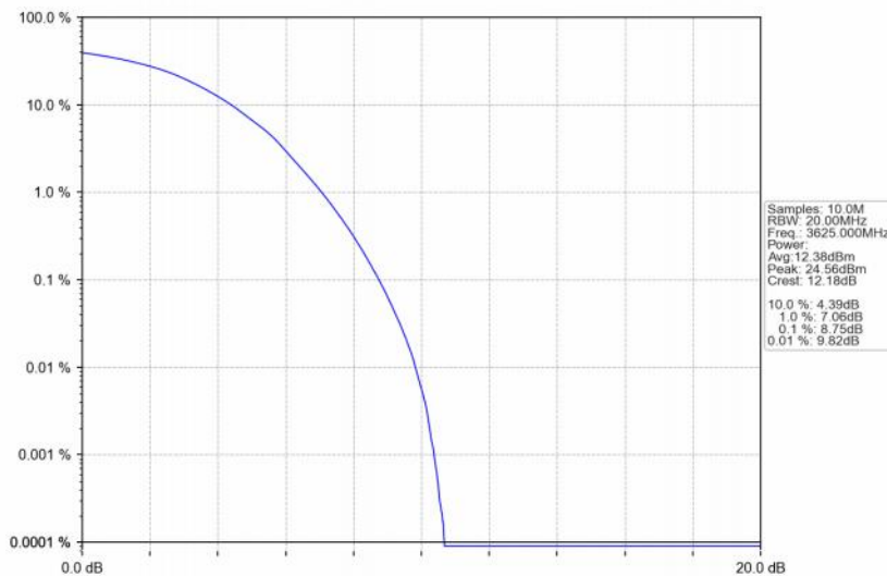
Band48_20MHz_16QAM_MCH_3625MHz_RB_100_0_NTNV
