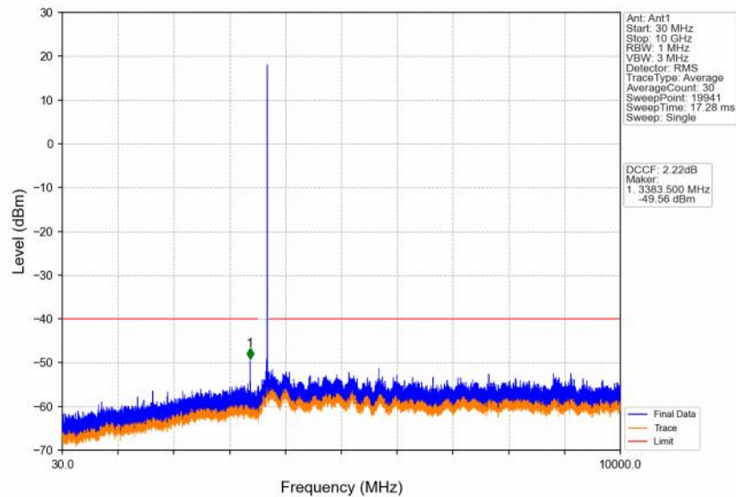
Band48_10MHz_QPSK_HCH_3695MHz_RB_1_0_NTNV
