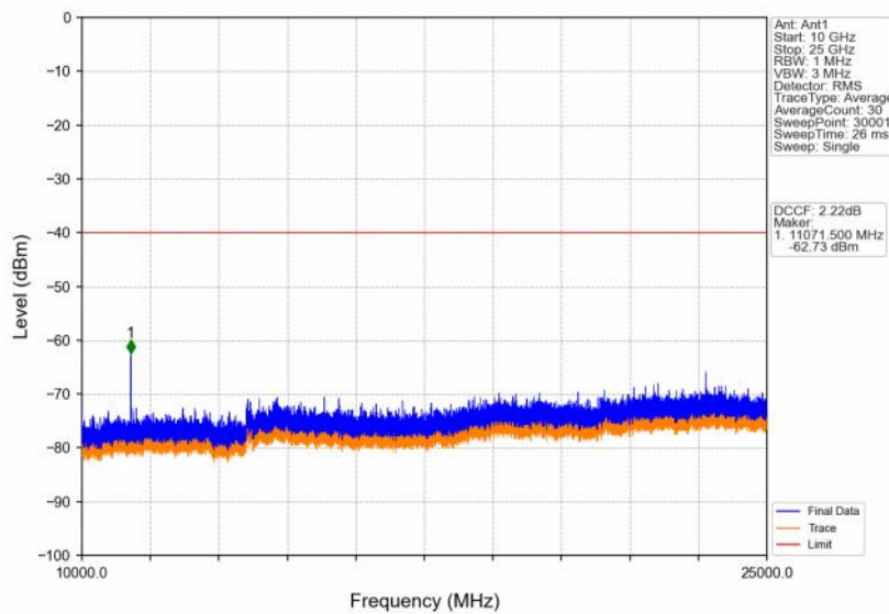
Band48_10MHz_QPSK_HCH_3695MHz_RB_1_0_NTNV
