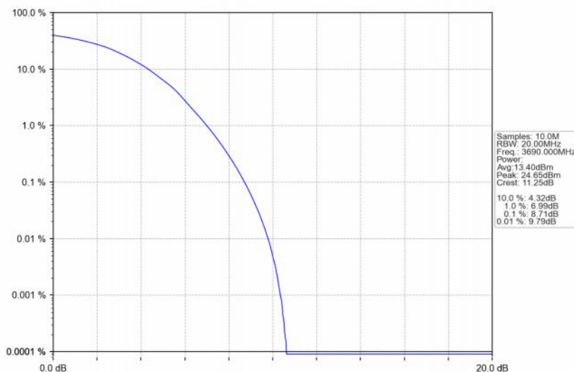
Band48_20MHz_16QAM_HCH_3690MHz_RB_100_0_NTNV
