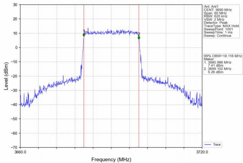
Band48_20MHz_256QAM_HCH_3690MHz_RB_100_0_NTNV
