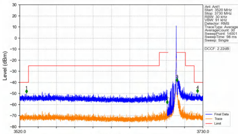
Band48_10MHz_QPSK_HCH_3695MHz_RB_1_49_NTNV
