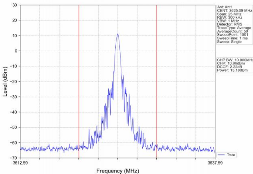
Band48_10MHz_256QAM_MCH_3625MHz_RB_1_25_NTNV
