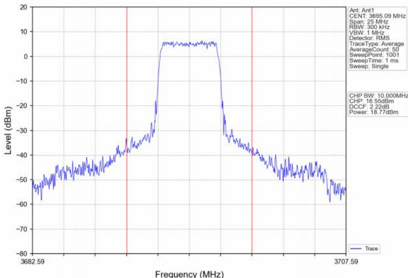
Band48_10MHz_QPSK_HCH_3695MHz_RB_25_25_NTNV
