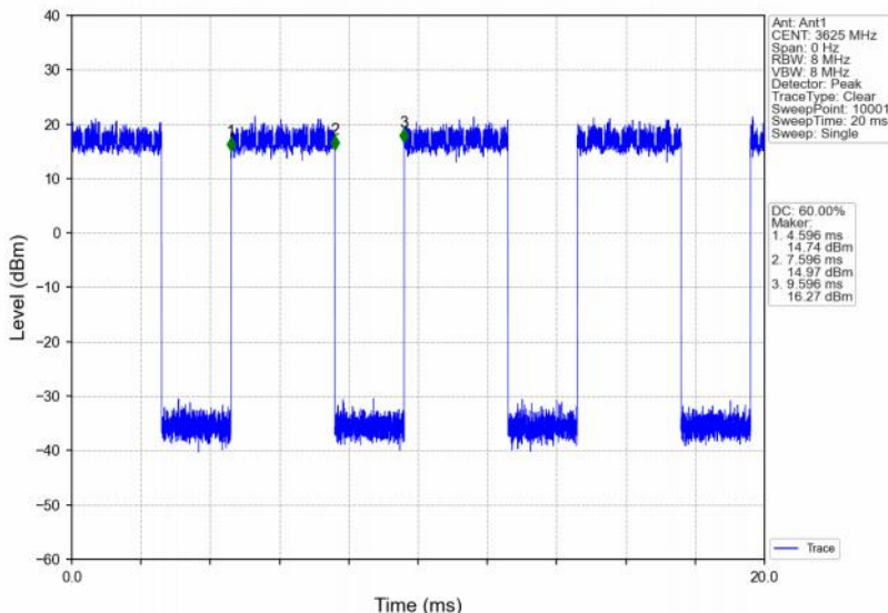
Band48_20MHz_256QAM_MCH_3625MHz_RB_50_50_NTNV
