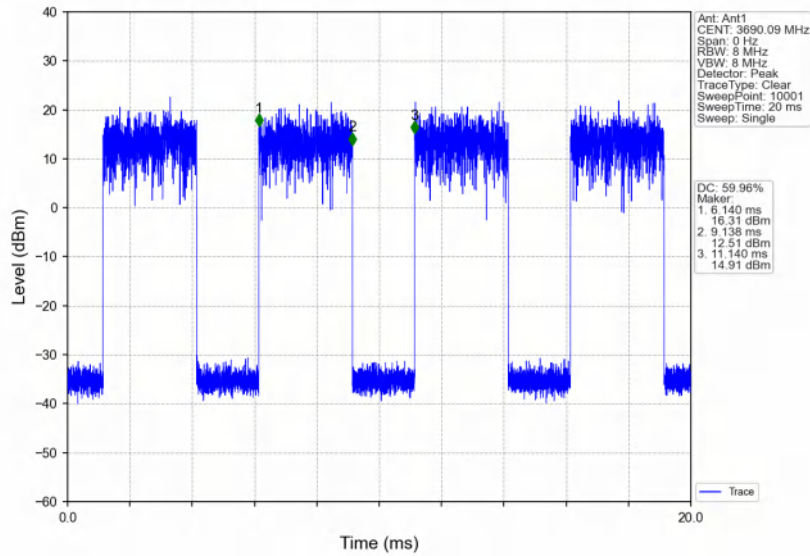
Band48_20MHz_256QAM_HCH_3690MHz_RB_1_99_NTNV
