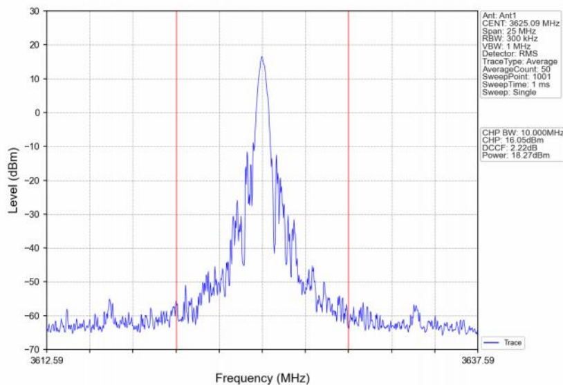
Band48_10MHz_16QAM_MCH_3625MHz_RB_1_25_NTNV
