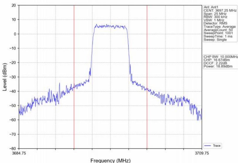
Band48_10MHz_QPSK_HCH_3695MHz_RB_25_25_NTNV
