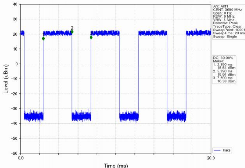
Band48_20MHz_QPSK_HCH_3690MHz_RB_50_50_NTNV
