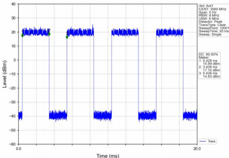
Band48_20MHz_64QAM_LCH_3560MHz_RB_50_50_NTNV
