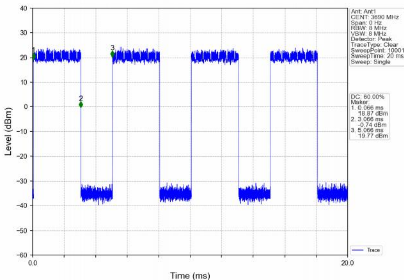
Band48_20MHz_16QAM_HCH_3690MHz_RB_50_25_NTNV
