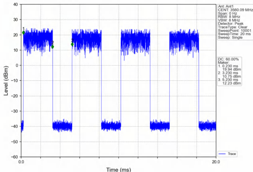
Band48_20MHz_16QAM_LCH_3560MHz_RB_1_99_NTNV
