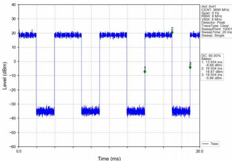
Band48_20MHz_16QAM_HCH_3690MHz_RB_100_0_NTNV
