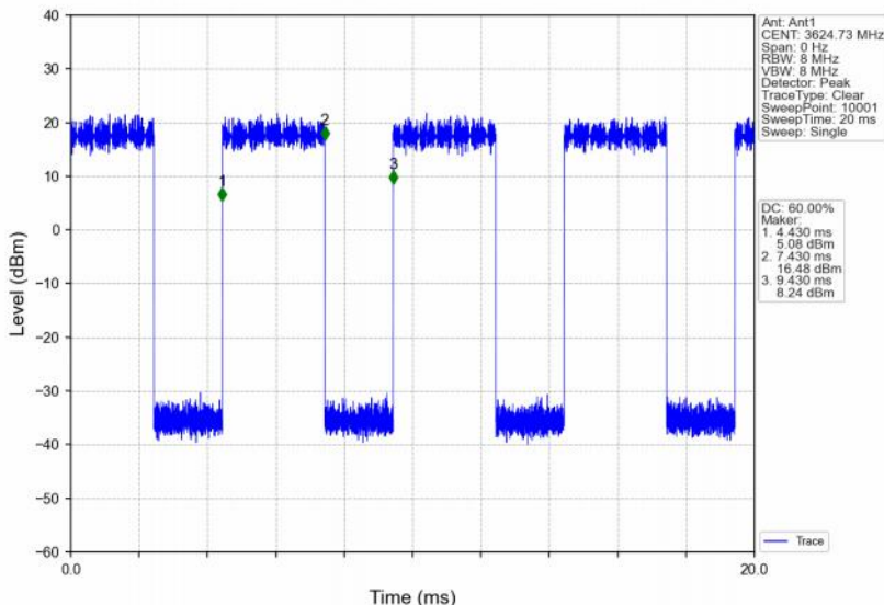
Band48_15MHz_256QAM_MCH_3625MHz_RB_36_39_NTNV
