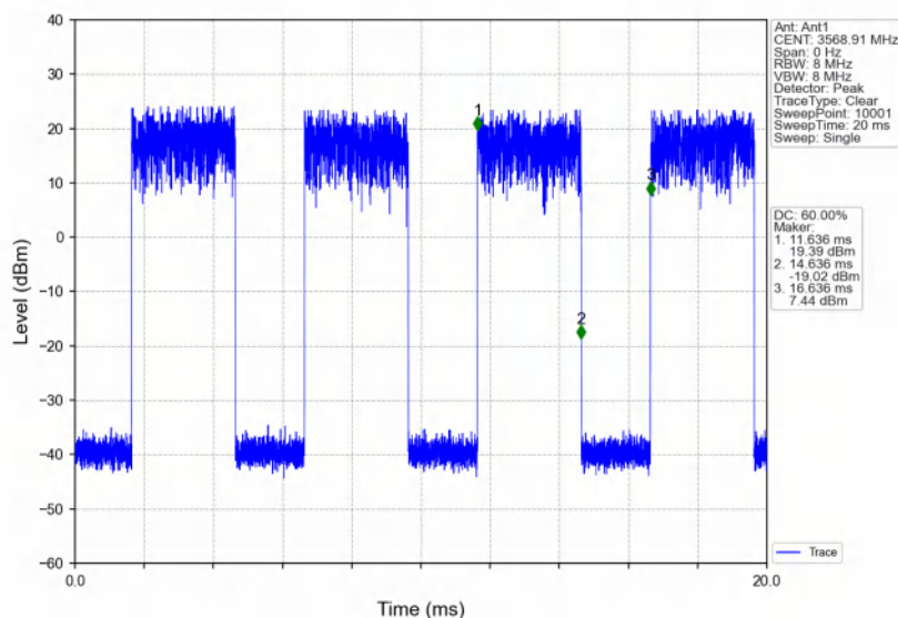
Band48_20MHz_16QAM_LCH_3560MHz_RB_1_99_NTNV
