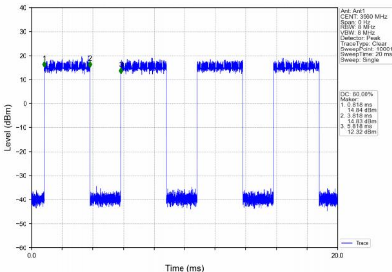
Band48_20MHz_256QAM_LCH_3560MHz_RB_100_0_NTNV
