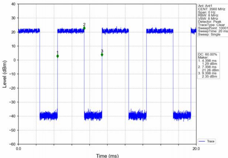
Band48_20MHz_QPSK_LCH_3560MHz_RB_50_50_NTNV
