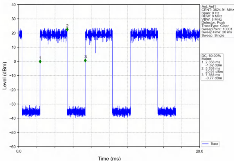
Band48_5MHz_64QAM_MCH_3625MHz_RB_12_6_NTNV
