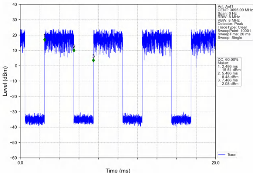
Band48_10MHz_16QAM_HCH_3695MHz_RB_1_49_NTNV
