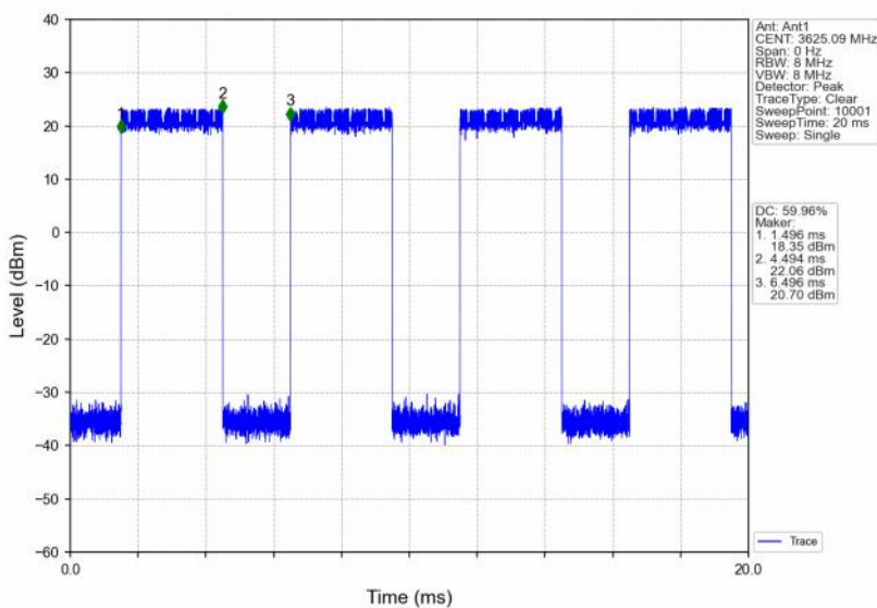
Band48_10MHz_QPSK_MCH_3625MHz_RB_25_13_NTNV
