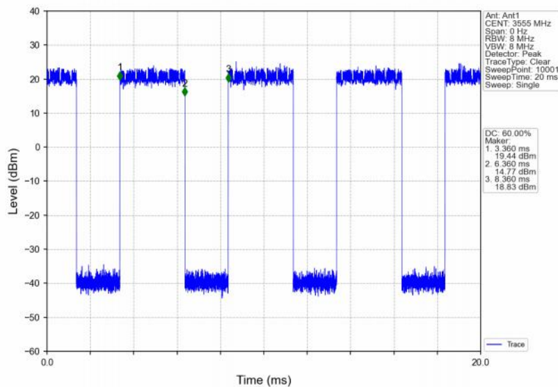
Band48_10MHz_16QAM_LCH_3555MHz_RB_50_0_NTNV
