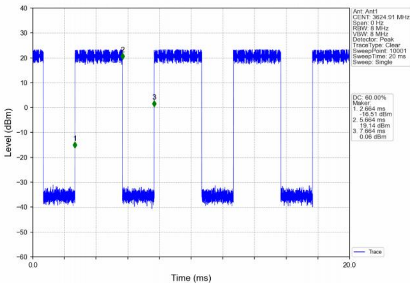
Band48_5MHz_QPSK_MCH_3625MHz_RB_12_6_NTNV
