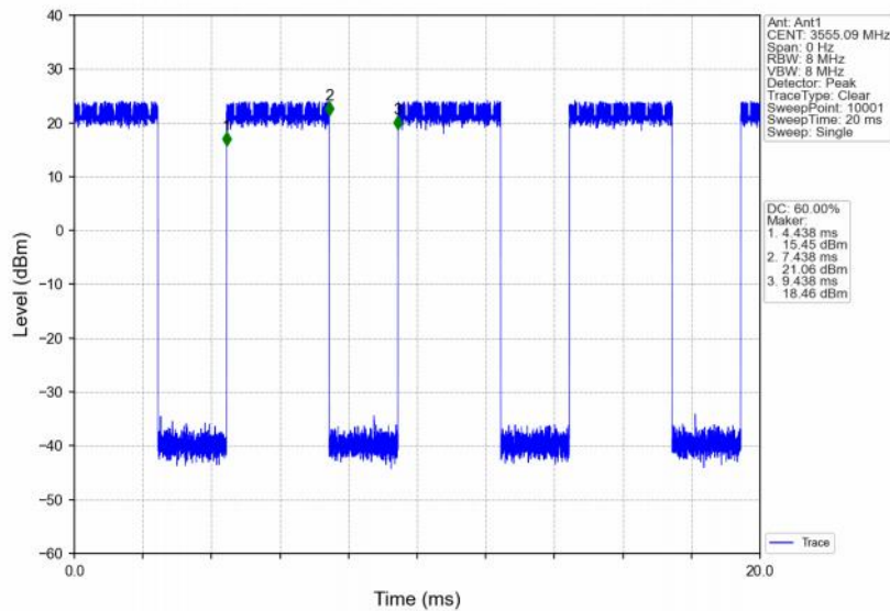
Band48_10MHz_QPSK_LCH_3555MHz_RB_25_25_NTNV
