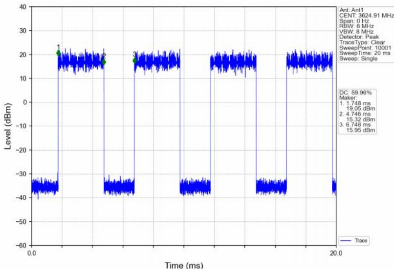
Band48_5MHz_256QAM_MCH_3625MHz_RB_12_13_NTNV
