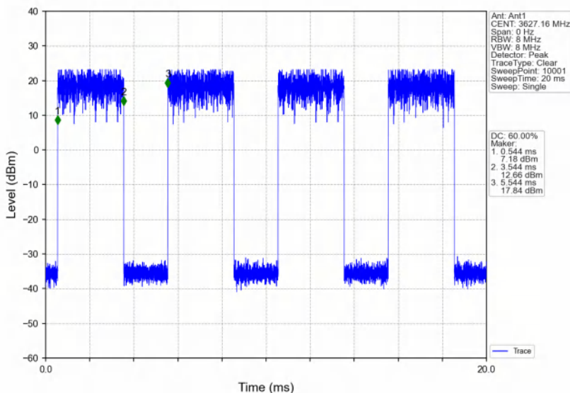
Band48_5MHz_QPSK_MCH_3625MHz_RB_1_24_NTNV
