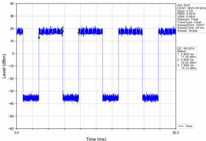
Band48_10MHz_256QAM_MCH_3625MHz_RB_25_25_NTNV
