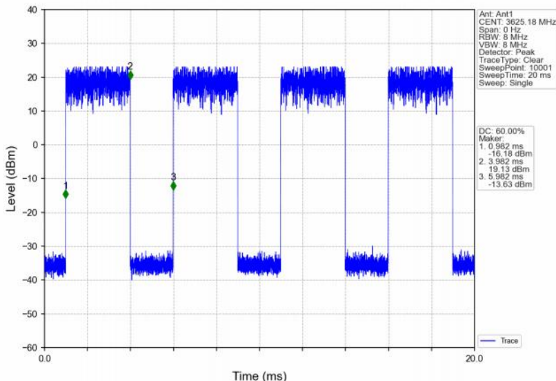
Band48_5MHz_QPSK_MCH_3625MHz_RB_1_24_NTNV
