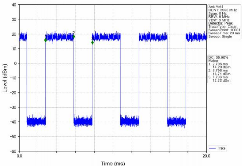
Band48_10MHz_256QAM_LCH_3555MHz_RB_50_0_NTNV
