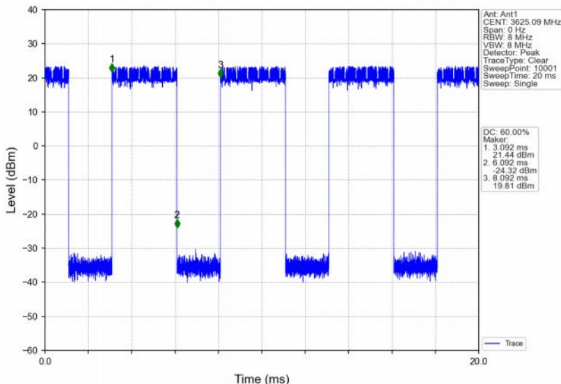
Band48_10MHz_16QAM_MCH_3625MHz_RB_25_25_NTNV
