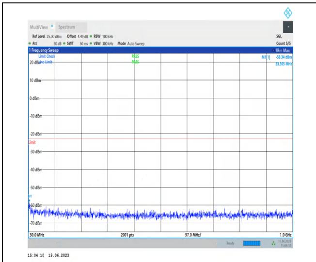
1-N66-PC3-15-40-M-1-DFT-PI2BPSK-Inner_1RB_L eft-1 @ 1-30-1000-Ant3-33.40--58.34--23-PASS
