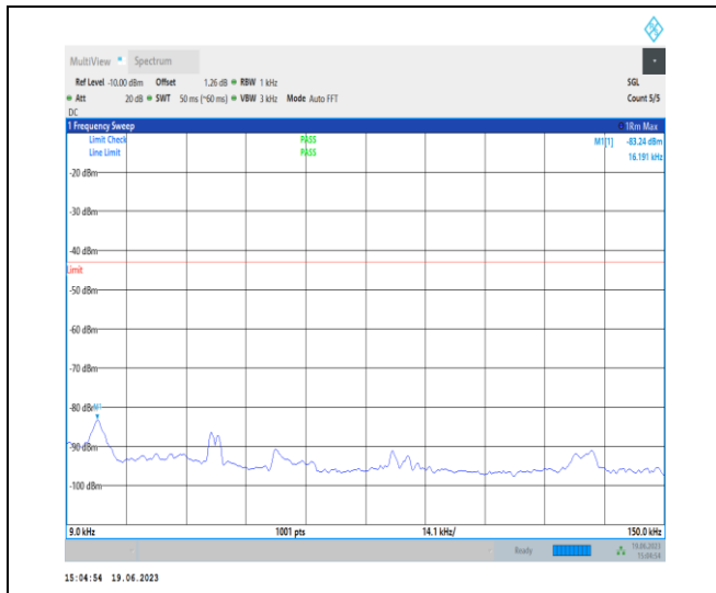
1-N66-PC3-15-40-H-1-DFT-PI2BPSK-Inner_1RB_L eft-1@1-0.009-0.15-Ant3-0.02--83.24--43-PASS
