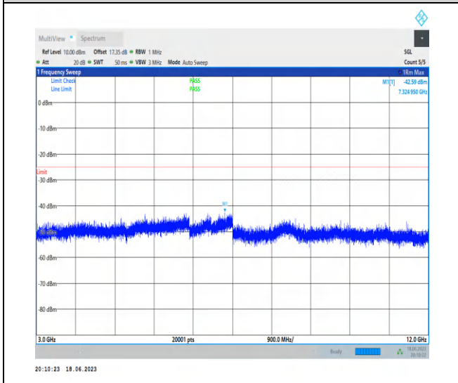
1-N41-PC3-30-100-M-1-N/A-DFT-PI2BPSK-Inner_1 RB_Left-1@1-3000-12000-Ant0-7324.95--42.59--25 -PASS
