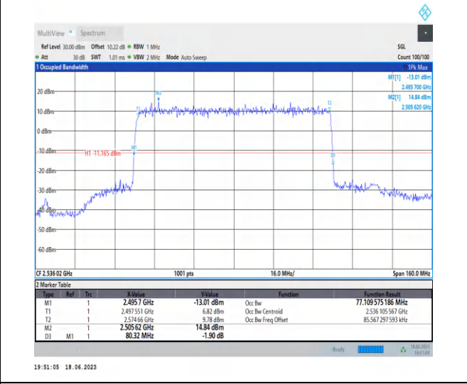
1-N41-PC3-30-80-L-2-DFT-QPSK-Outer_Full-216@ 0-Ant0-77.11-80.320-≤80-PASS
