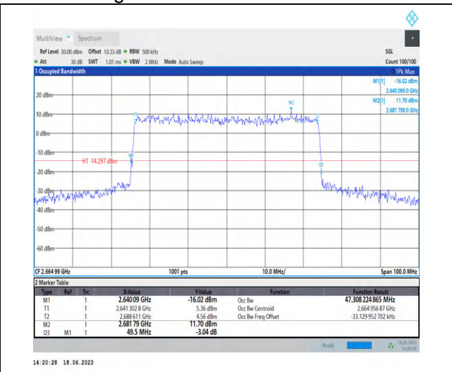
1-N41-PC3-30-50-H-7-CP-16QAM-Outer_Full-133@0 -Ant0-47.308-49.500-≤50-PASS
