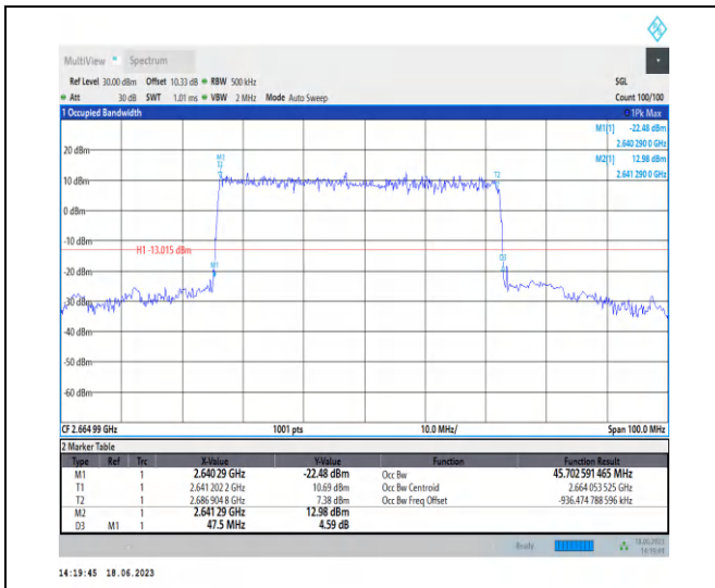
1-N41-PC3-30-50-H-2-DFT-QPSK-Outer_Full-128@ @0-Ant0-45.703-47.500-≤50-PASS
