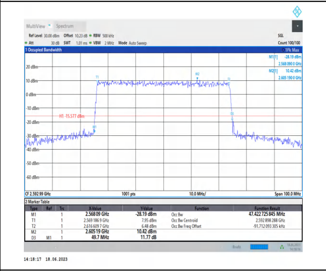
1-N41-PC3-30-50-M-6-CP-QPSK-Outer_Full-133 @ 0-Ant0-47.423-49.700-≤50-PASS
