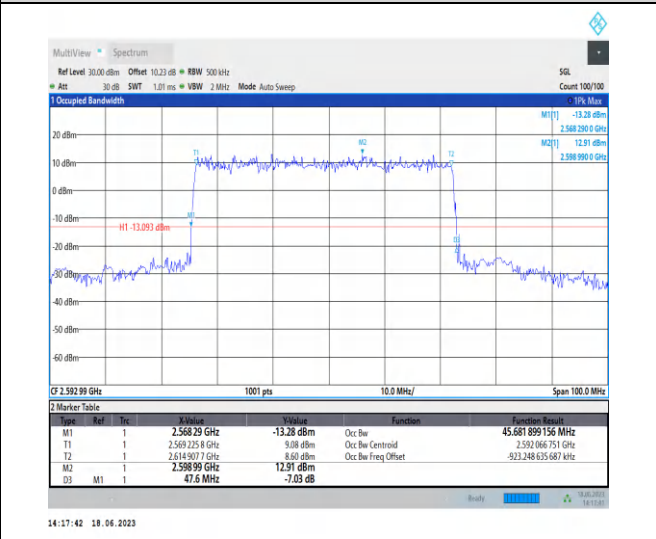
1-N41-PC3-30-50-M-2-DFT-QPSK-Outer_Full-128@ 0-Ant0-45.682-47.600-≤50-PASS
