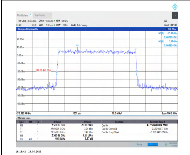
1-N41-PC3-30-50-M-9-CP-256QAM-Outer_Full-133 @0-Ant0-47.558-49.500-≤50-PASS
