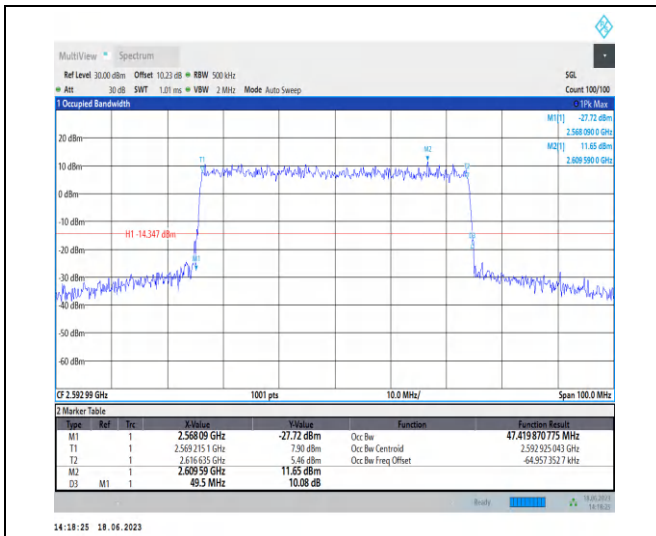
1-N41-PC3-30-50-M-7-CP-16QAM-Outer_Full-133@ 0-Ant0-47.42-49.500-≤50-PASS
