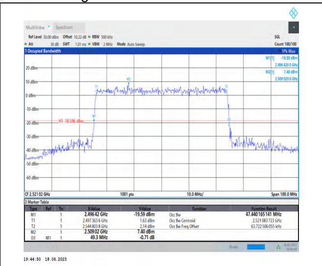
1-N41-PC3-30-50-L-9-CP-256QAM-Outer_Full-133 @0-Ant0-47.44-49.300-≤50-PASS
