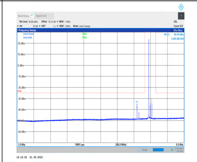
1-N38-PC3-30-40-M-1-N/A-DFT-PI2BPSK-Inner_1R B_Left-1@1-1000-3000-Ant0-2801.00--36.33--25-PASS
