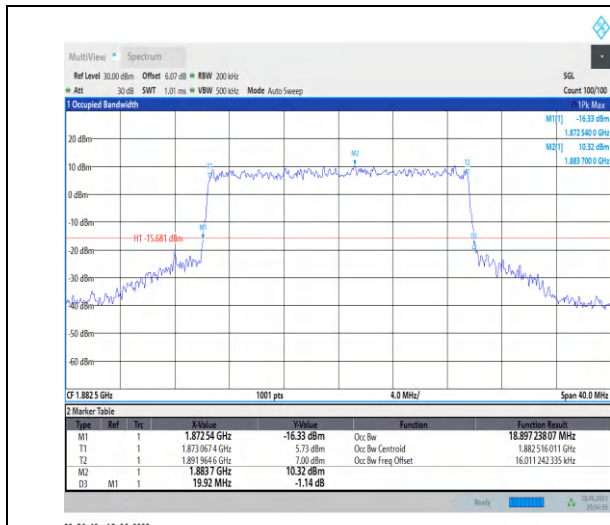
1-N25-PC3-15-20-M-7-CP-16QAM-Outer_Full-106@ -0-Ant3-18.897-19.920-<20-PASS
