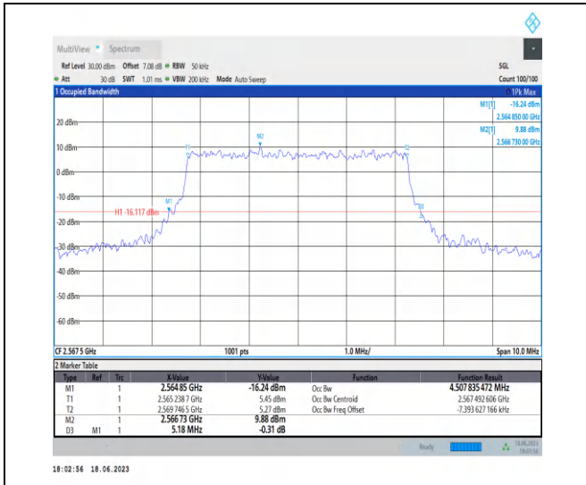
1-N7-PC3-15-5-H-7-CP-16QAM-Outer_Full-25@0-A nt0-4.508-5.180-≤5-PASS
