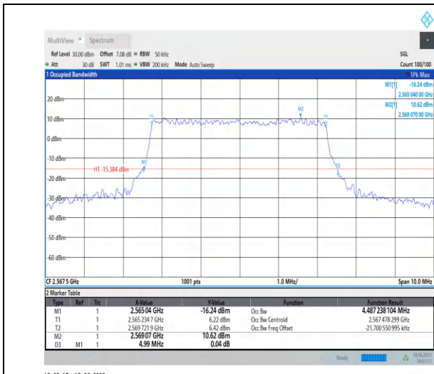
1-N7-PC3-15-5-H-3-DFT-16QAM-Outer_Full-25@0-A nt0-4.487-4.990 \leq 5 -PASS
