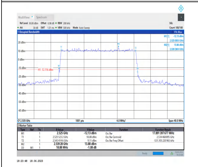
1-N7-PC3-15-20-M-1-DFT-QPSK-Outer_Full-100@ 0-Ant0-17.891-18.880-≤20-PASS
