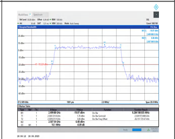
1-N7-PC3-15-10-L-9-CP-256QAM-Outer_Full-52@0-A Ant0-9.284-10.100≤10-PASS
