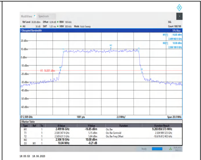
1-N7-PC3-15-10-L-7-CP-16QAM-Outer_Full-52@0-A nt0-9.284-10.040≤10-PASS
