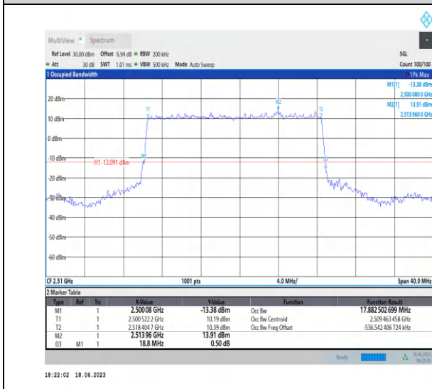
1-N7-PC3-15-20-L-2-DFT-PI2BPSK-Outer_Full-100@0-Ant0-17.883-18.800-≤20-PASS
