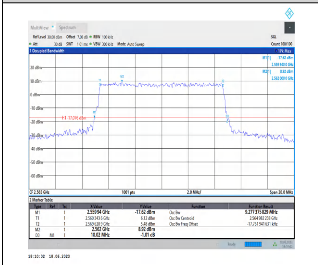
1-N7-PC3-15-10-H-6-CP-QPSK-Outer_Full-52@0-A nt0-9.277-10.020-≤10-PASS
