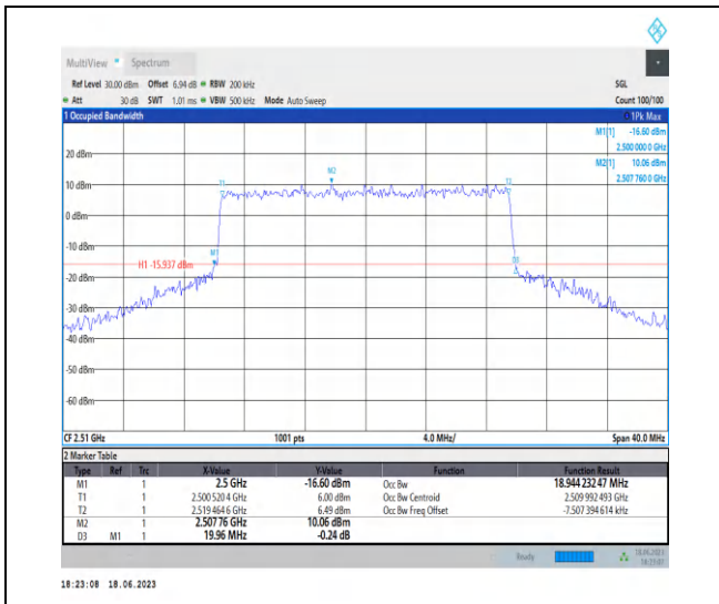
1-N7-PC3-15-20-L-8-CP-64QAM-Outer_Full-106@ 0-Ant0-18.944-19.960-≤20-PASS
