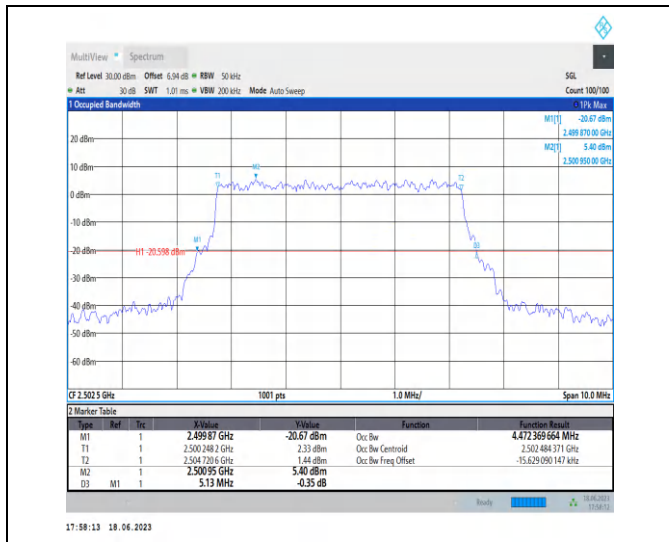
1-N7-PC3-15-5-L-9-CP-256QAM-Outer_Full-25@0-A Ant0-4.472-5.130-≤5-PASS
