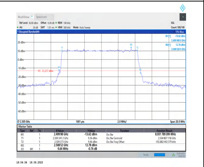
1-N7-PC3-15-10-L-1-DFT-QPSK-Outer_Full-50@0-A nt0-8.932-9.640-≤10-PASS
