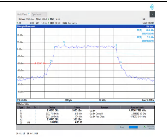
1-N7-PC3-15-5-M-9-CP-256QAM-Outer_Full-25@0-A nt0-4.477-5.090-≤5-PASS
