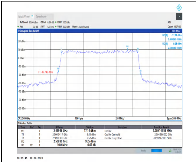
1-N7-PC3-15-10-L-6-CP-QPSK-Outer_Full-52@0-A nt0-9.289-10.000≤10-PASS
