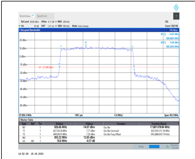
1-N5-PC3-15-20-M-3-DFT-16QAM-Outer_Full-100@ 0-Ant0-17.801-18.600-<20-PASS
