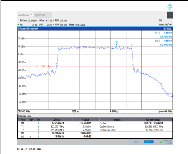
1-N5-PC3-15-20-M-7-CP-16QAM-Outer_Full-106@0 -Ant0-18.879-19.800-≤20-PASS
