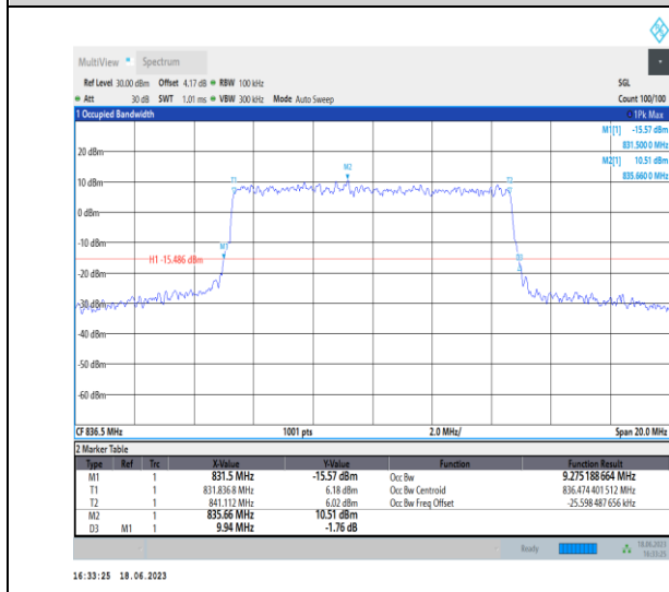
1-N5-PC3-15-10-M-7-CP-16QAM-Outer_Full-52@0-A nt0-9.275-9.940-≤10-PASS
