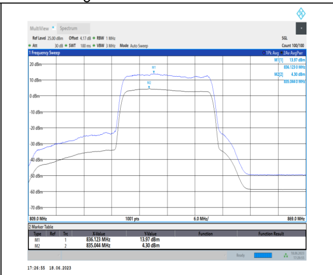
1-N5-PC3-15-20-H-2-CP-256QAM-Outer_Full-106@ 0-Ant0-9.67-100%-0.00-9.67-PASS-≤13
