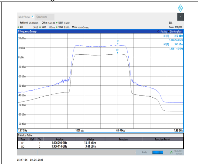
1-N2-PC3-15-20-H-2-CP-256QAM-Outer_Full-106@ 0-Ant3-9.72-100%-0.00-9.72-PASS-≤13
