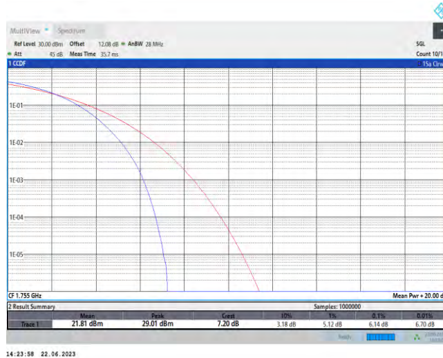
66-66-20MHz-20MHz-QPSK-QPSK-132323-132521-100RB#0-100RB#0
