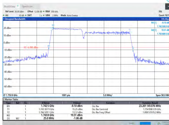
66-66-10MHz-15MHz-QPSK-QPSK-132351-132471-50RB#0-75RB#0
