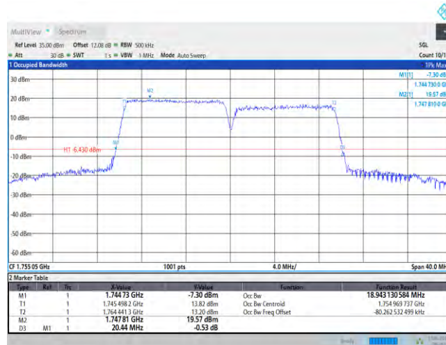
66-66-10MHz-10MHz-QPSK-QPSK-132373-132472-50RB#0-50RB#0
