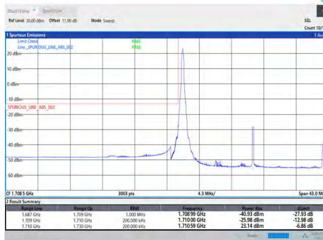
66-66-10MHz-10MHz-QPSK-QPSK-132022-132121-50RB#0-50RB#0
