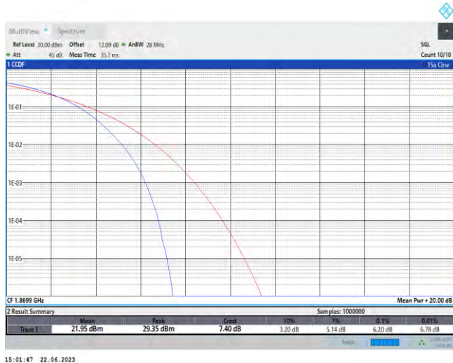
2-2-20MHz-20MHz-QPSK-QPSK-18801-18999-100RB#0-100RB#0
