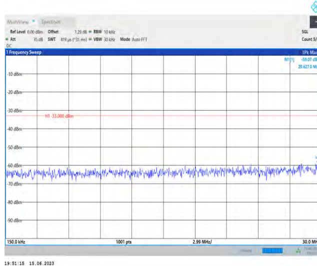
Band43-20MHz-QPSK-44690-1RB#0-Range2:0.15~30MHz
