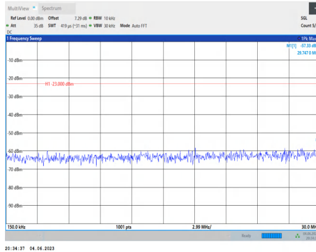
Band26-10MHz-QPSK-26740-1RB#0-Range2:0.15~30MHz
