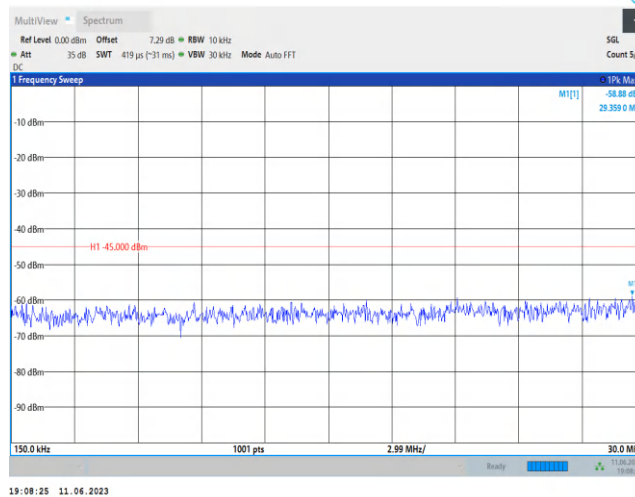
Band7-20MHz-QPSK-20850-1RB#0-Range2:0.15~30MHz
