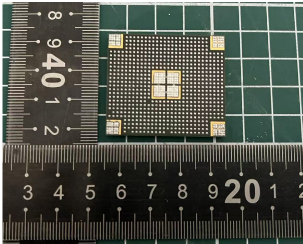
EUT
