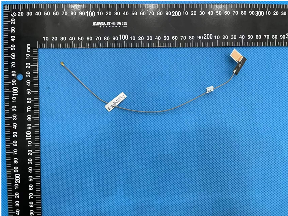
BT/WIFI ANT1
