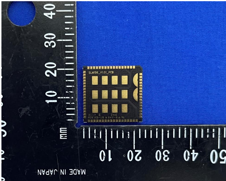
(2) EUT Photo
