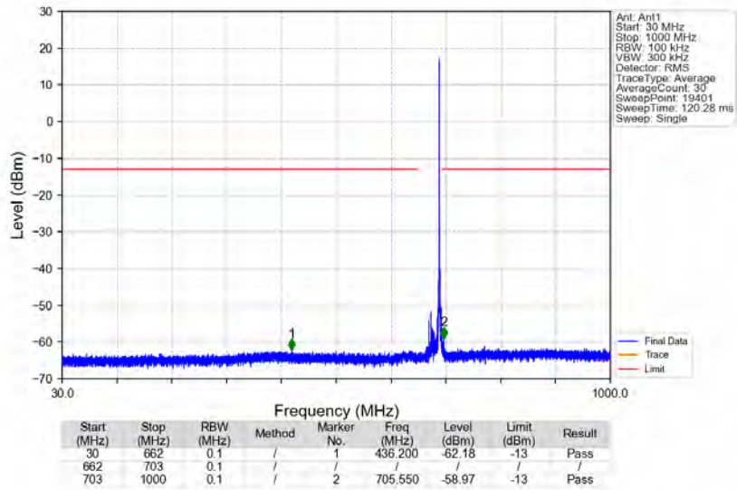
n71_15kHz_SISO_NTNV_20MHz_CP-OFDM QPSK_688MHz_Edge_1RB_Right
