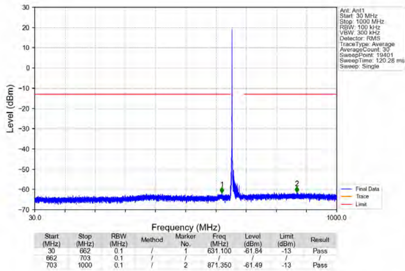
n71_15kHz_SISO_NTNV_20MHz_DFT-s-OFDM QPSK_673MHz_Edge_1RB_Left
