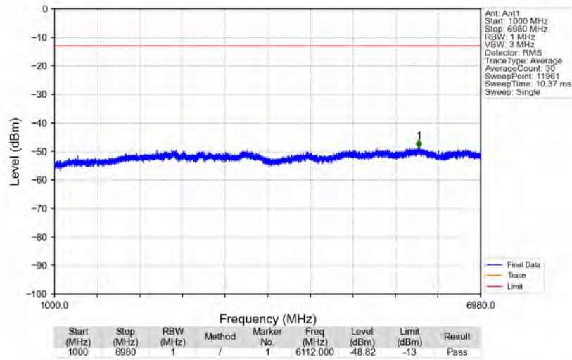
n71_15kHz_SISO_NTNV_20MHz_CP-OFDM QPSK_673MHz_Edge_1RB_Left
