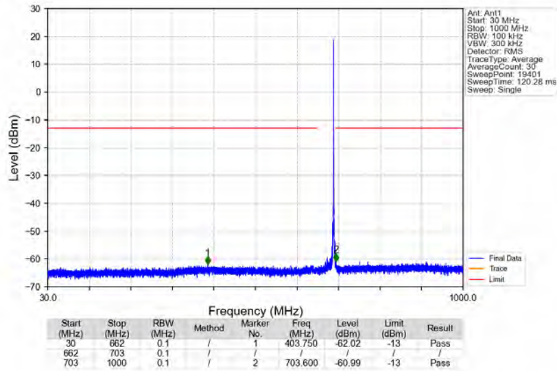
n71_15kHz_SISO_NTNV_20MHz_DFT-s-OFDM QPSK_688MHz_Edge_1RB_Right
