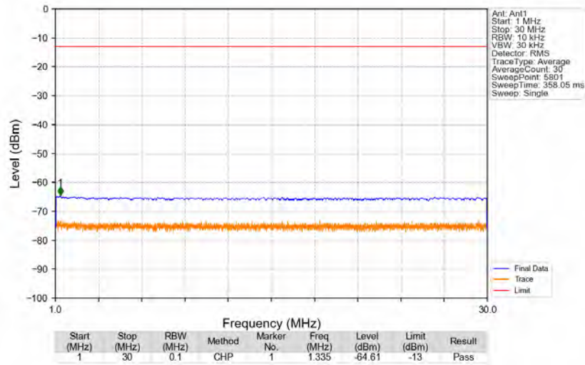
n71_15kHz_SISO_NTNV_20MHz_DFT-s-OFDM QPSK_673MHz_Edge_1RB_Left
