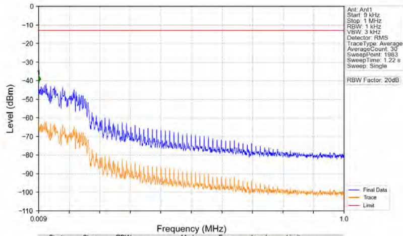
n71_15kHz_SISO_NTNV_20MHz_CP-OFDM QPSK_688MHz_Edge_1RB_Right
