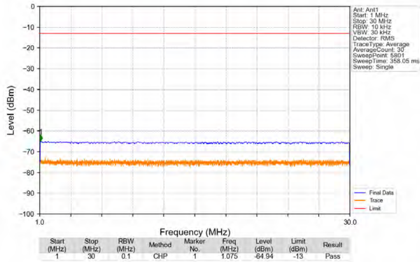
n71_15kHz_SISO_NTNV_20MHz_CP-OFDM QPSK_673MHz_Edge_1RB_Left
