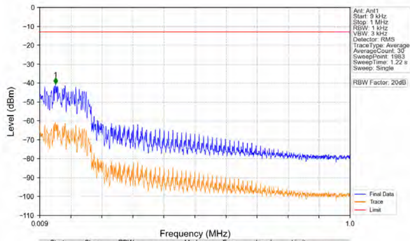
n71_15kHz_SISO_NTNV_20MHz_DFT-s-OFDM QPSK_688MHz_Edge_1RB_Right
