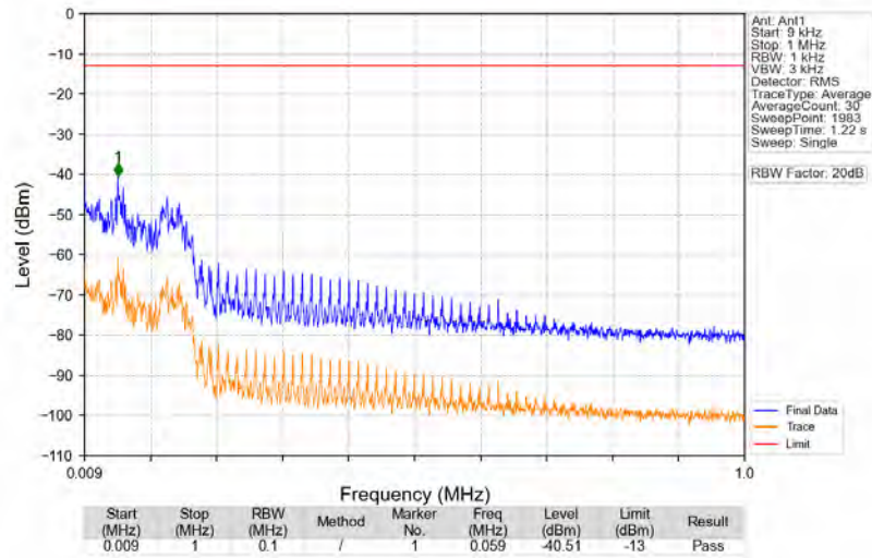
n71_15kHz_SISO_NTV_20MHz_DFT-s-OFDM PI/2 BPSK_680.5MHz_Edge_1RB_Left
