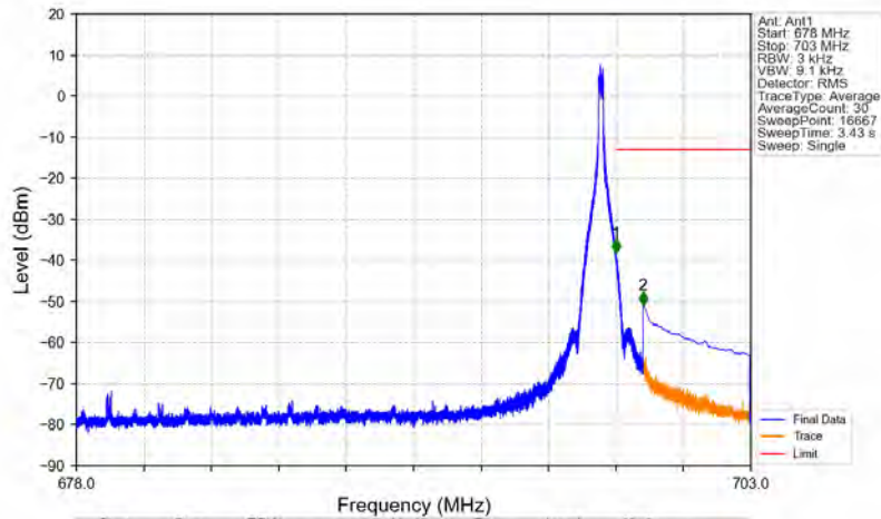
n71_15kHz_SISO_NTNV_20MHz_DFT-s-OFDM QPSK_688MHz_Edge_1RB_Right
