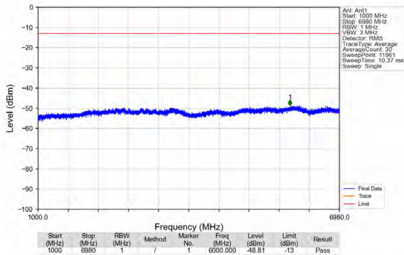
n71_15kHz_SISO_NTNV_20MHz_CP-OFDM QPSK_688MHz_Edge_1RB_Right
