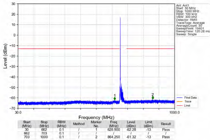
n71_15kHz_SISO_NTNV_20MHz_CP-OFDM QPSK_673MHz_Edge_1RB_Left
