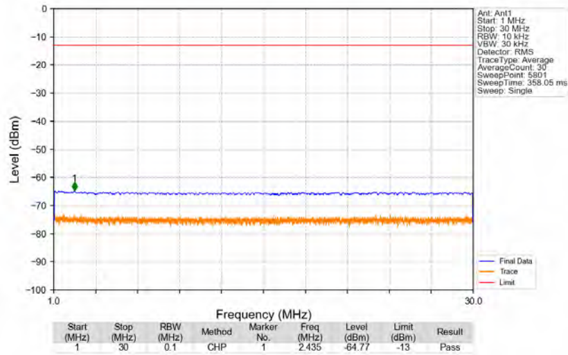
n71_15kHz_SISO_NTNV_20MHz_DFT-s-OFDM QPSK_688MHz_Edge_1RB_Right
