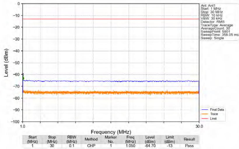
n71_15kHz_SISO_NTNV_20MHz_DFT-s-OFDM PI/2 BPSK_673MHz_Edge_1RB_Left
