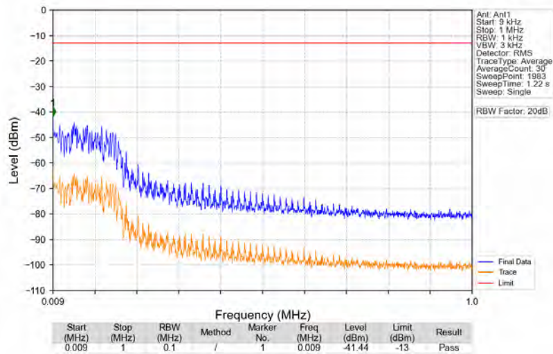
n71_15kHz_SISO_NTV_20MHz_DFT-s-OFDM QPSK_673MHz_Edge_1RB_Left
