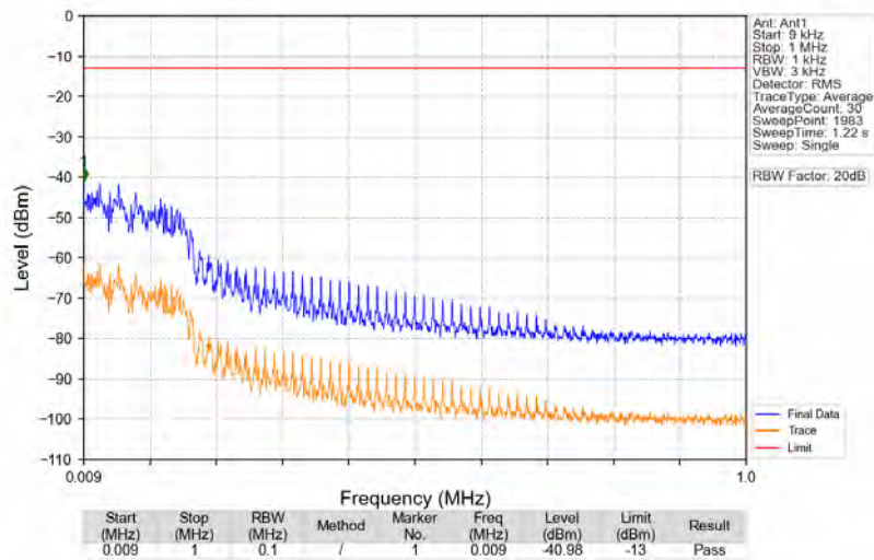
n71_15kHz_SISO_NTV_10MHz_CP-OFDM QPSK_668MHz_Edge_1RB_Left
