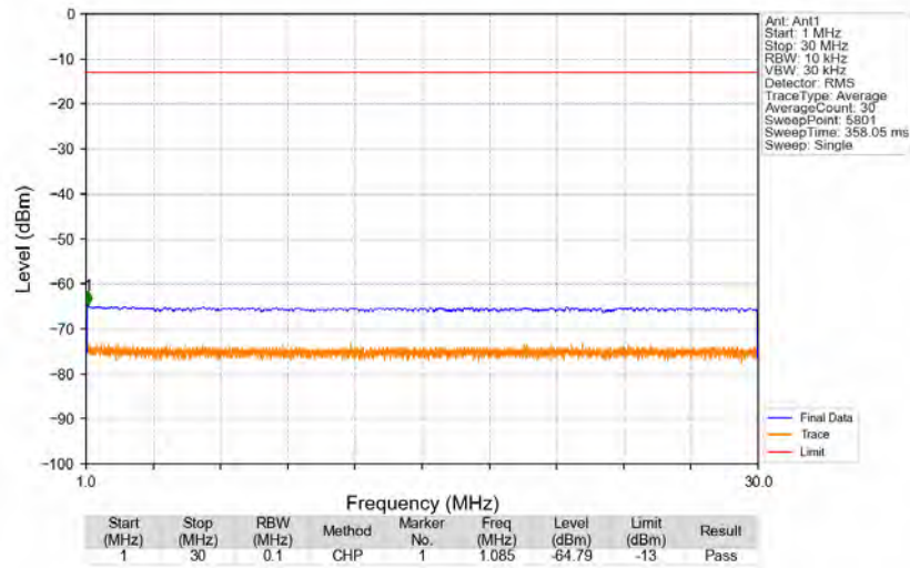
n71_15kHz_SISO_NTV_20MHz_DFT-s-OFDM PI/2 BPSK_680.5MHz_Edge_1RB_Left
