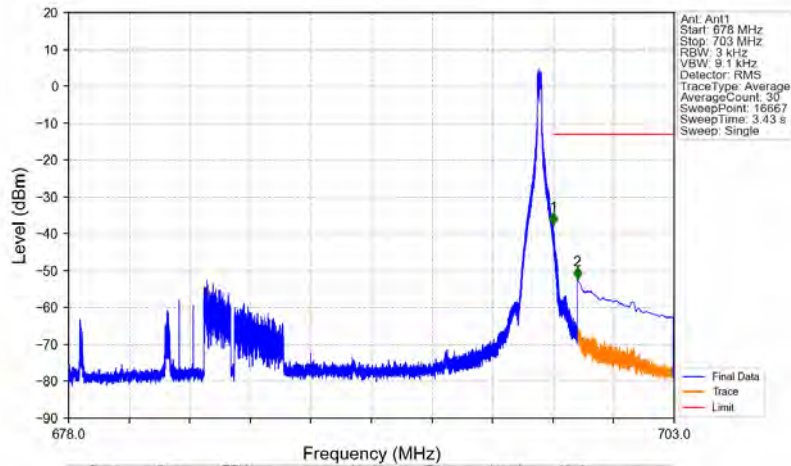
n71_15kHz_SISO_NTNV_20MHz_CP-OFDM QPSK_688MHz_Edge_1RB_Right
