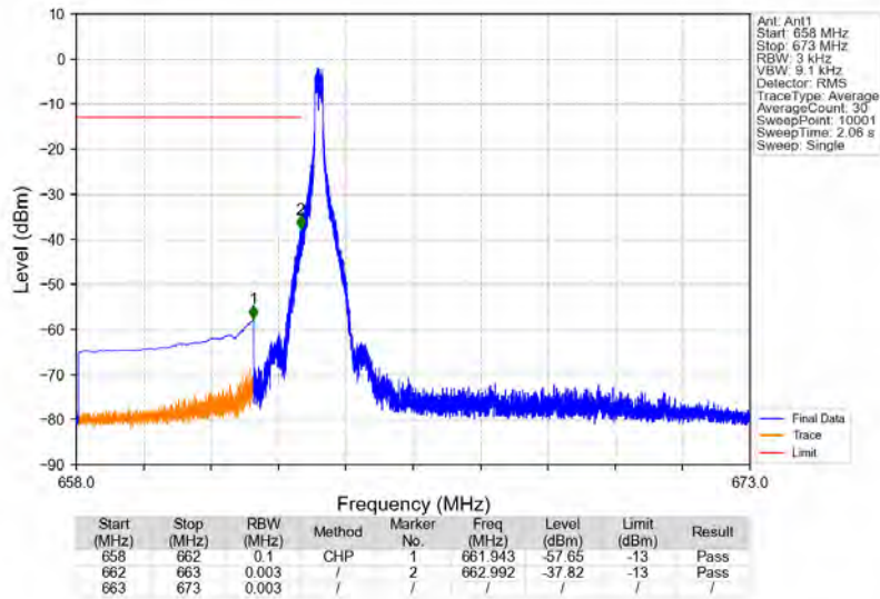
n71_15kHz_SISO_NTV_10MHz_CP-OFDM QPSK_668MHz_Edge_1RB_Left
