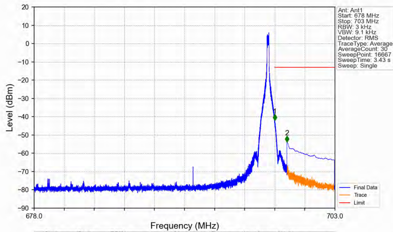
n71_15kHz_SISO_NTNV_20MHz_DFT-s-OFDM PI/2 BPSK_688MHz_Edge_1RB_Right
