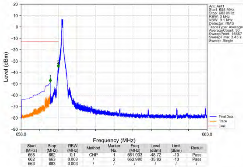
n71_15kHz_SISO_NTNV_20MHz_DFT-s-OFDM PI/2 BPSK_673MHz_Edge_1RB_Left
