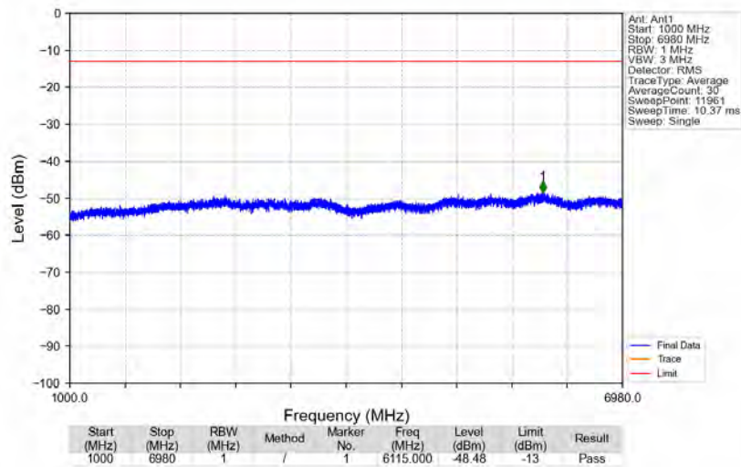
n71_15kHz_SISO_NTNV_20MHz_DFT-s-OFDM QPSK_688MHz_Edge_1RB_Right
