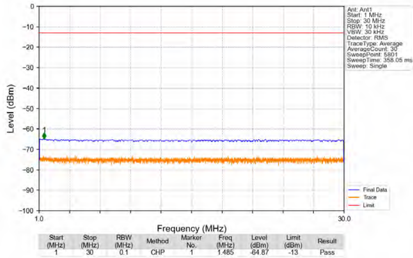
n71_15kHz_SISO_NTNV_10MHz_DFT-s-OFDM PI/2 BPSK_668MHz_Edge_1RB_Left
