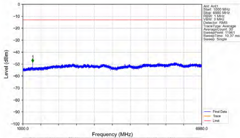
n71_15kHz_SISO_NTNV_20MHz_DFT-s-OFDM PI/2 BPSK_673MHz_Edge_1RB_Left
