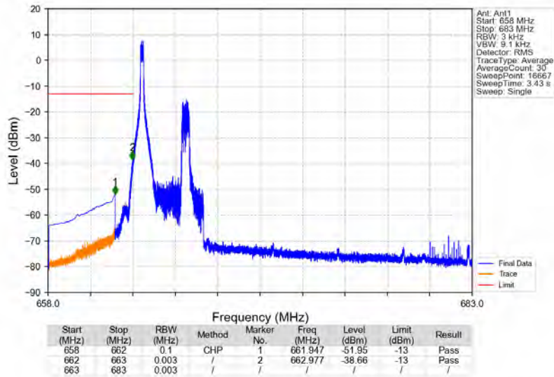
n71_15kHz_SISO_NTV_20MHz_DFT-s-OFDM QPSK_673MHz_Edge_1RB_Left
