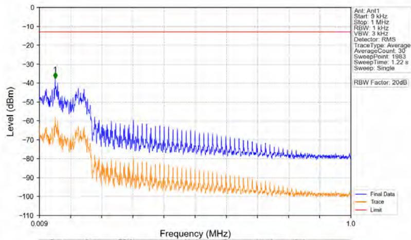
n71_15kHz_SISO_NTNV_20MHz_DFT-s-OFDM PI/2 BPSK_688MHz_Edge_1RB_Right
