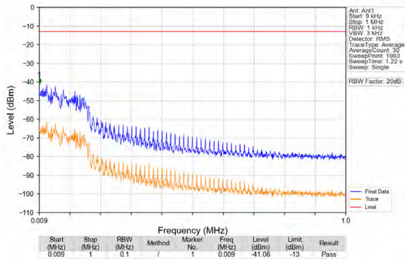
n71_15kHz_SISO_NTV_20MHz_CP-OFDM QPSK_673MHz_Edge_1RB_Left
