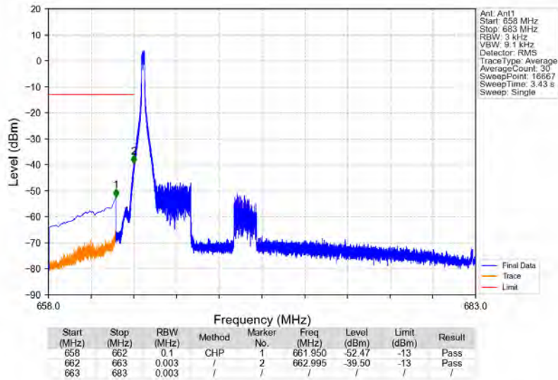
n71_15kHz_SISO_NTV_20MHz_CP-OFDM QPSK_673MHz_Edge_1RB_Left
