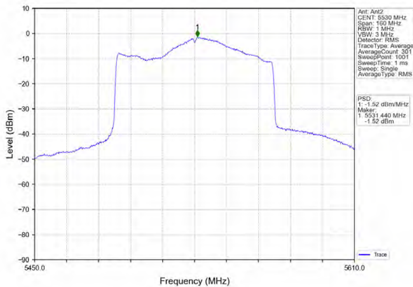
802.11ax(HEW80)_LCH_5530MHz_RU996_Left_Ant2_NTNV
