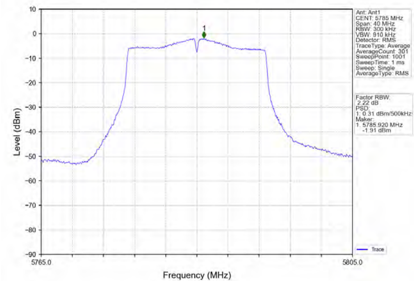
802.11n(HT20)_MCH_5785MHz_Ant1_NTNV
