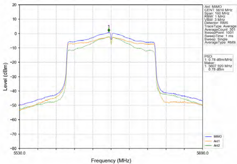
802.11ac(VHT80)_HCH_5610MHz_MIMO_NTNV
