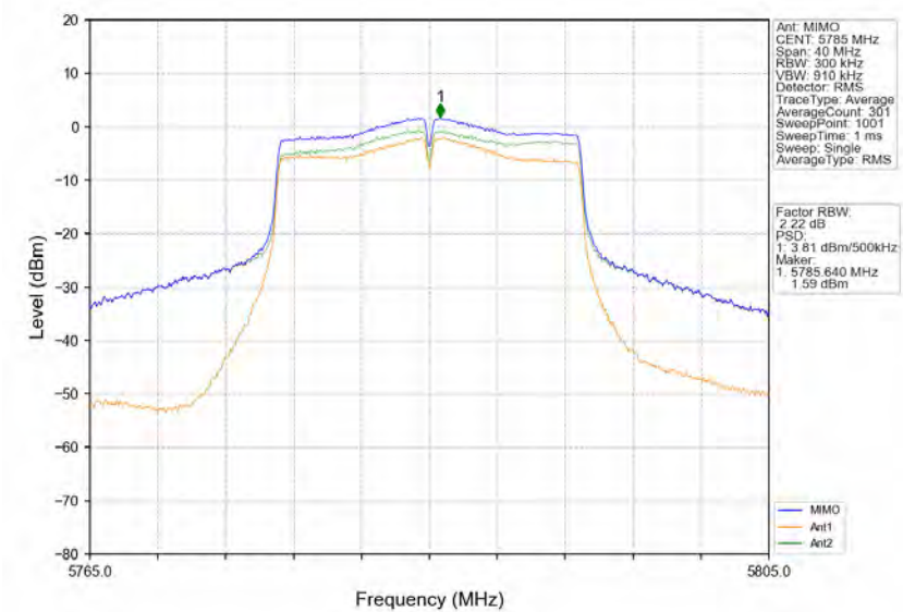
802.11n(HT20)_MCH_5785MHz_MIMO_NTNV
