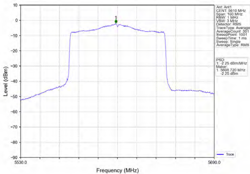
802.11ax(HEW80)_HCH_5610MHz_RU996_Left_Ant1_NTNV
