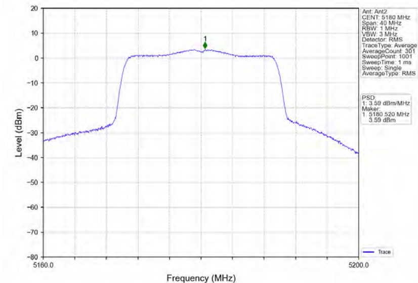
802.11ax(HEW20)_LCH_5180MHz_RU242_Left_Ant2_NTNV
