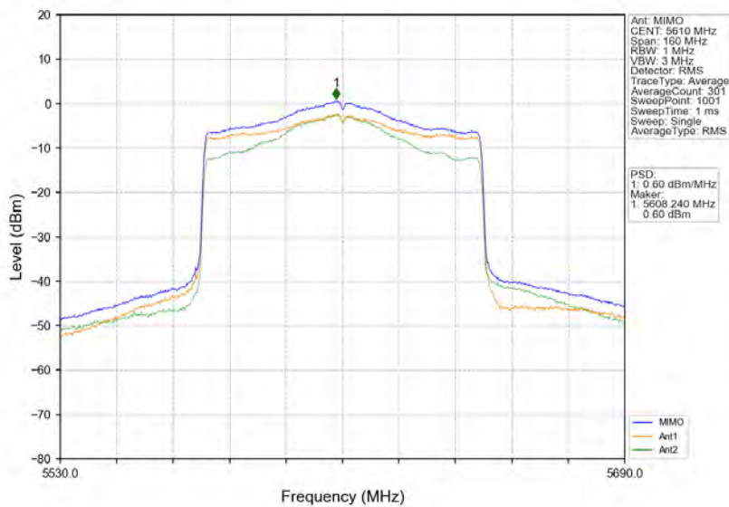
802.11ax(HEW80)_HCH_5610MHz_RU996_Left_MIMO_NTNV
