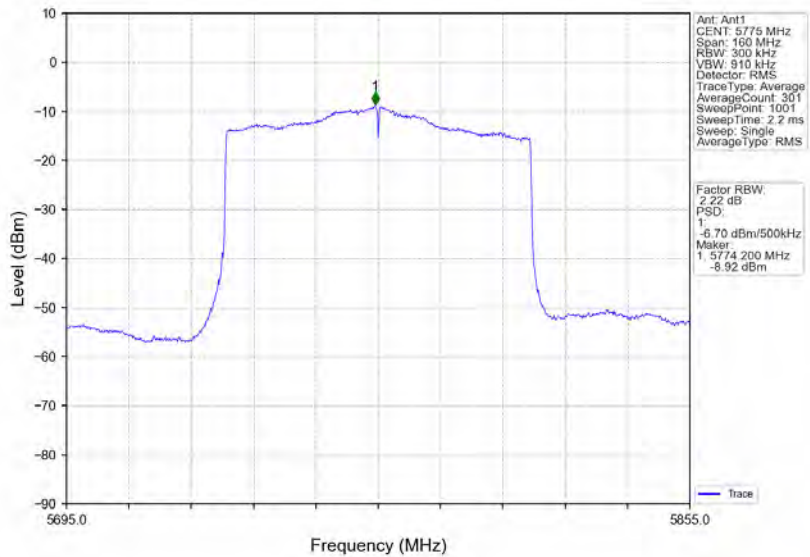
802.11ax(HEW80)_MCH_5775MHz_RU996_Left_Ant1_NTNV
