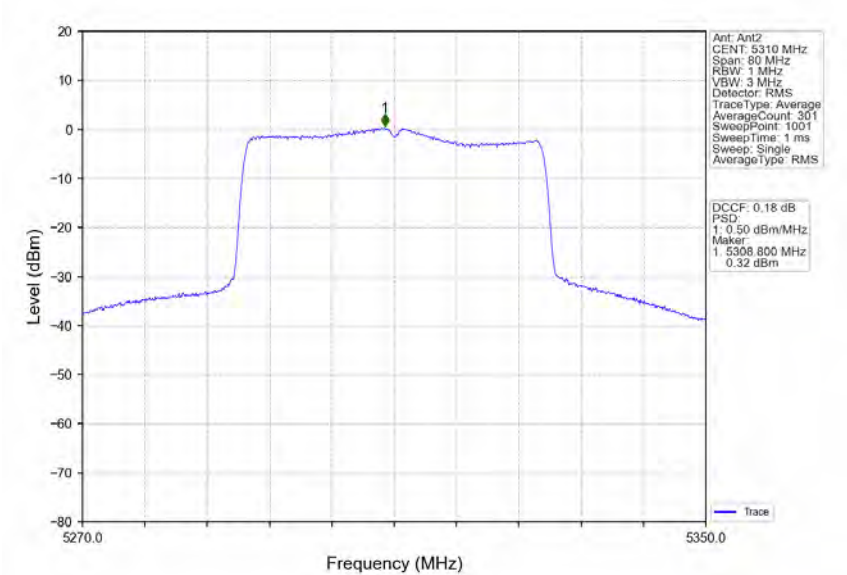
802.11ax(HEW40)_HCH_5310MHz_RU484_Left_Ant2_NTNV
