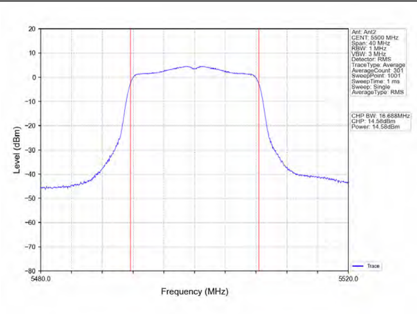
802.11a_LCH_5500MHz_Ant2_NTNV
