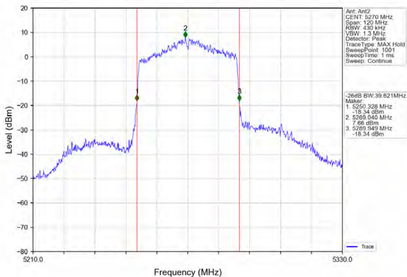
802.11ax(HEW40)_LCH_5270MHz_RU484_Left_Ant2_NTNV
