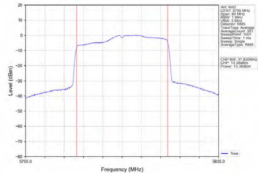
802.11ax(HEW40)_HCH_5795MHz_RU484_Left_Ant2_NTNV
