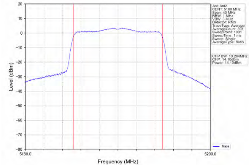
802.11ax(HEW20)_LCH_5180MHz_RU242_Left_Ant2_NTNV
