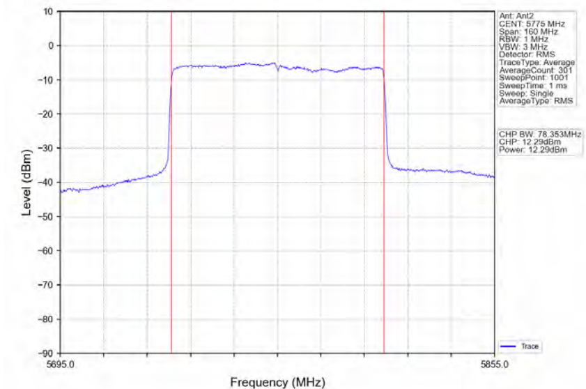
802.11ax(HEW80)_MCH_5775MHz_RU996_Left_Ant2_NTNV
