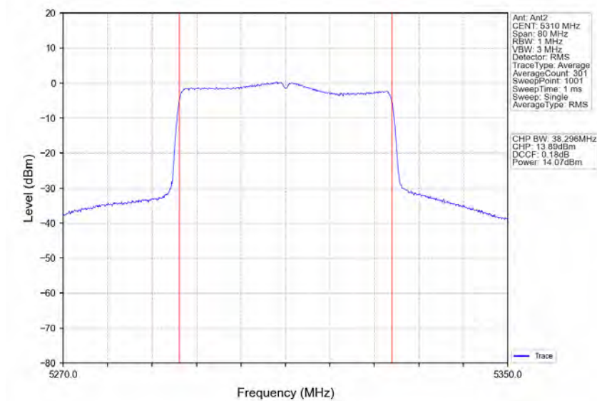
802.11ax(HEW40)_HCH_5310MHz_RU484_Left_Ant2_NTNV
