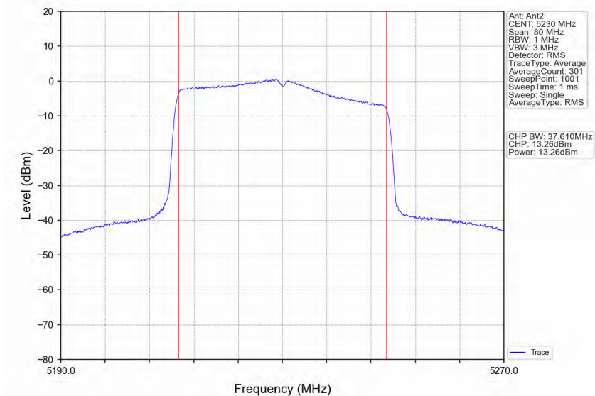
802.11ax(HEW40)_HCH_5230MHz_RU484_Left_Ant2_NTNV
