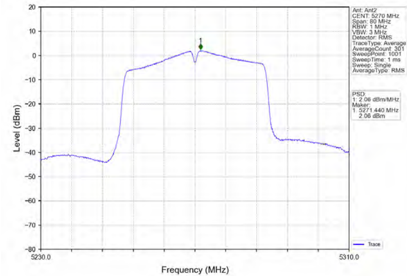
802.11n(HT40)_LCH_5270MHz_MIMO_NTNV
