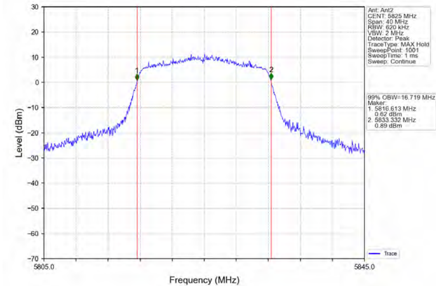
802.11a_HCH_5825MHz_Ant2_NTNV
