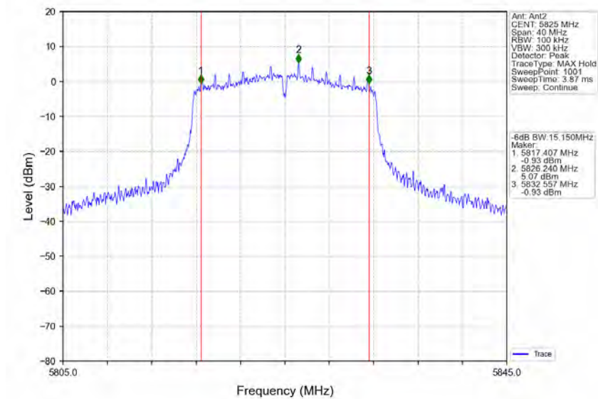
802.11a_HCH_5825MHz_Ant2_NTNV
