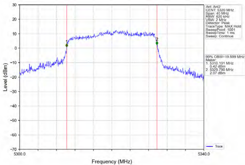
802.11ax(HEW20)_HCH_5320MHz_RU242_Left_Ant2_NTNV
