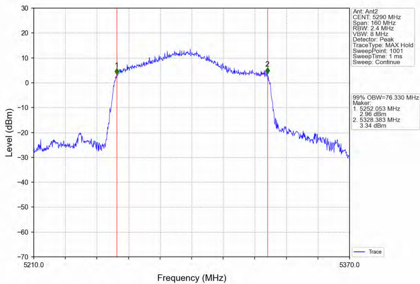
802.11ax(HEW80)_MCH_5290MHz_RU996_Left_Ant2_NTNV
