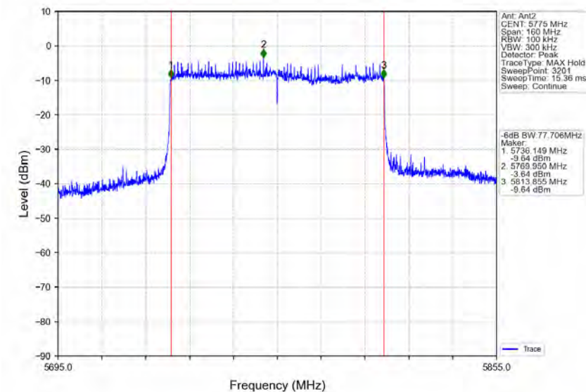
802.11ax(HEW80)_MCH_5775MHz_RU996_Left_Ant2_NTNV
