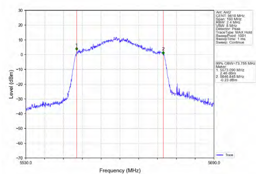
802.11ac(VHT80)_HCH_5610MHz_Ant2_NTNV
