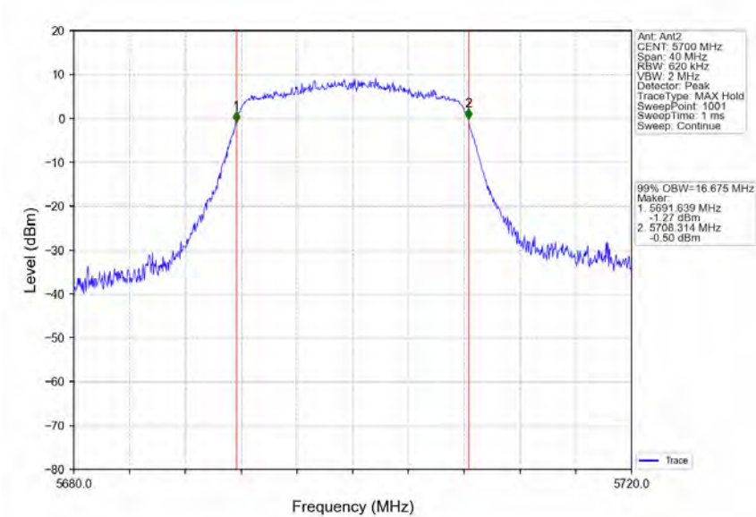
802.11a_HCH_5700MHz_Ant2_NTNV
