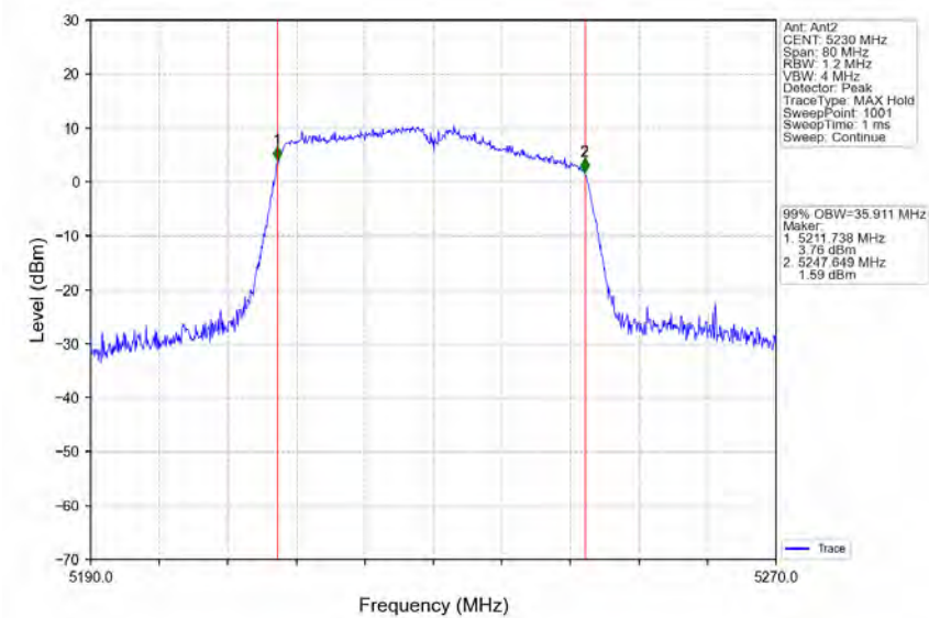
802.11n(HT40)_HCH_5230MHz_Ant2_NTNV
