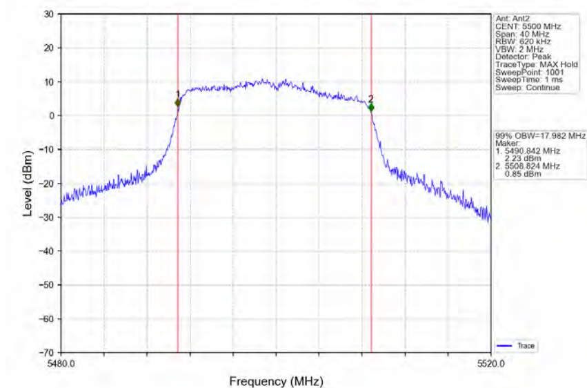
802.11n(HT20)_LCH_5500MHz_Ant2_NTNV
