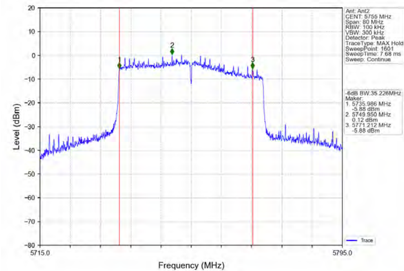
802.11ax(HEW40)_LCH_5755MHz_RU484_Left_Ant2_NTNV
