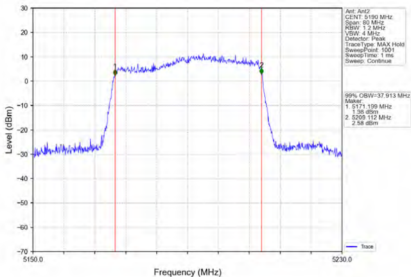
802.11ax(HEW40)_LCH_5190MHz_RU484_Left_Ant2_NTNV
