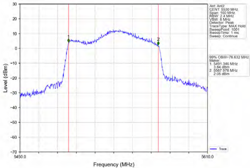
802.11ax(HEW80)_LCH_5530MHz_RU996_Left_Ant2_NTNV
