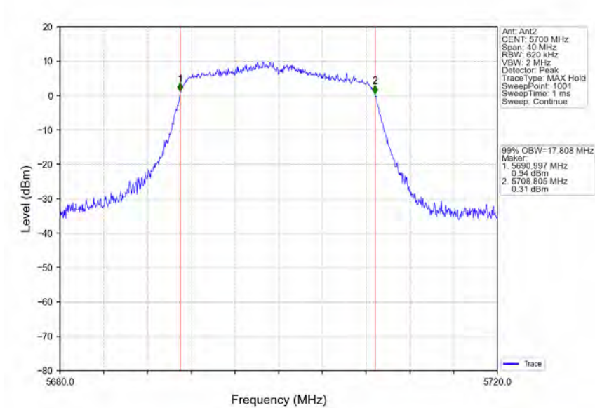
802.11n(HT20)_HCH_5700MHz_Ant2_NTNV
