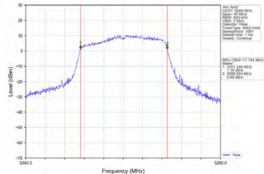
802.11n(HT20)_LCH_5260MHz_Ant2_NTNV
