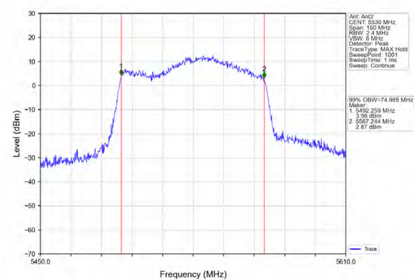
802.11ac(VHT80)_LCH_5530MHz_Ant2_NTNV
