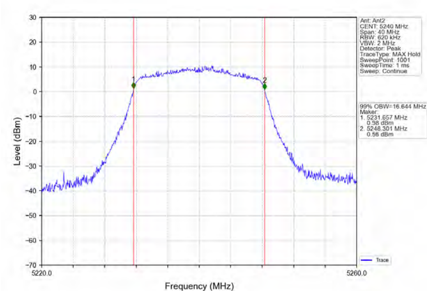
802.11a_HCH_5240MHz_Ant2_NTNV
