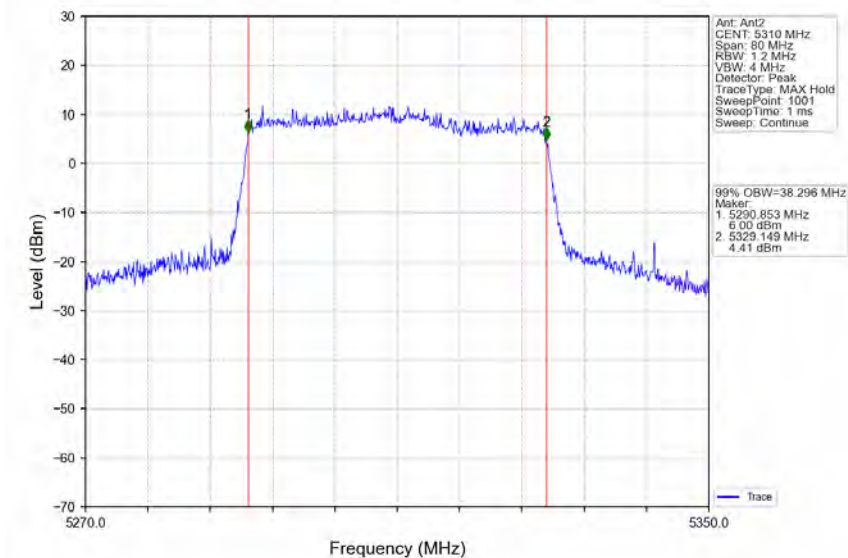
802.11ax(HEW40)_HCH_5310MHz_RU484_Left_Ant2_NTNV
