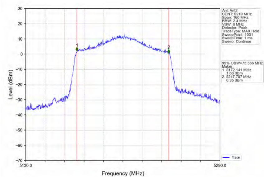
802.11ax(HEW80)_MCH_5210MHz_RU996_Left_Ant2_NTNV
