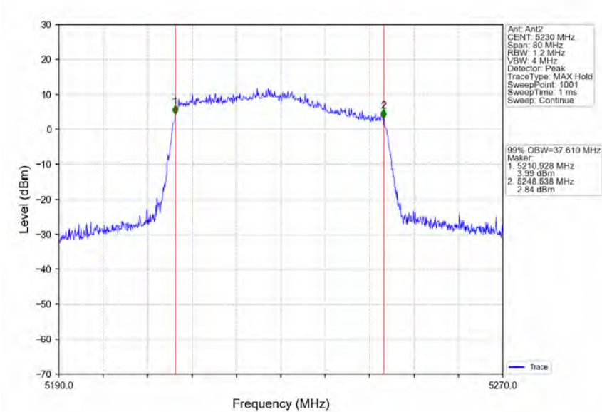
802.11ax(HEW40)_HCH_5230MHz_RU484_Left_Ant2_NTNV
