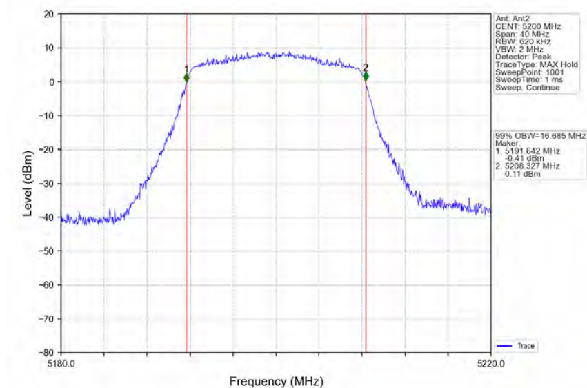
802.11a_MCH_5200MHz_Ant2_NTNV
