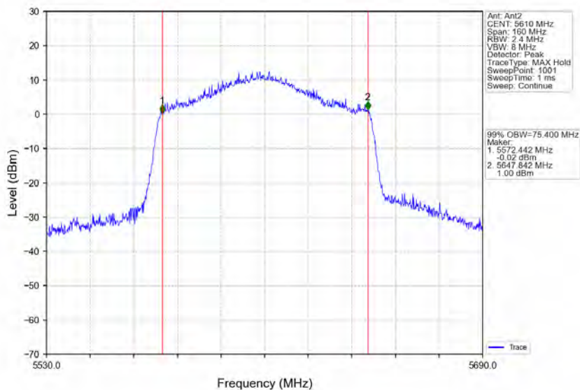
802.11ax(HEW80)_HCH_5610MHz_RU996_Left_Ant2_NTNV
