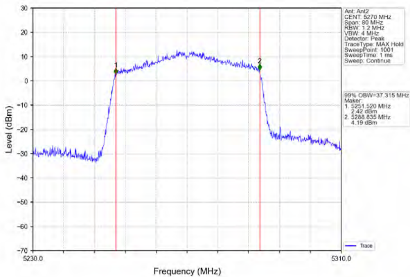
802.11ax(HEW40)_LCH_5270MHz_RU484_Left_Ant2_NTNV
