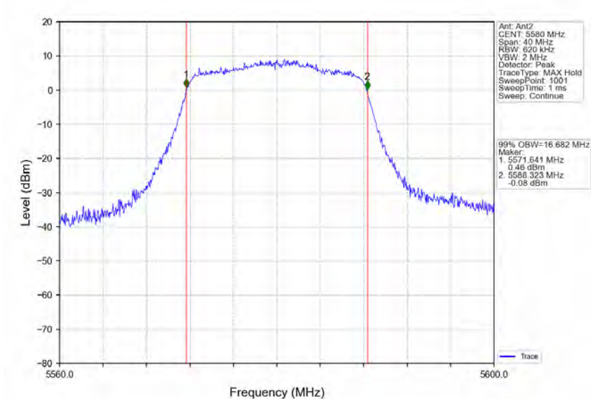
802.11a_MCH_5580MHz_Ant2_NTNV
