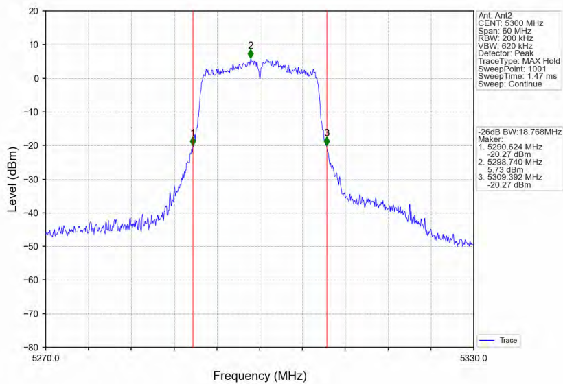
802.11a_MCH_5300MHz_Ant2_NTNV
