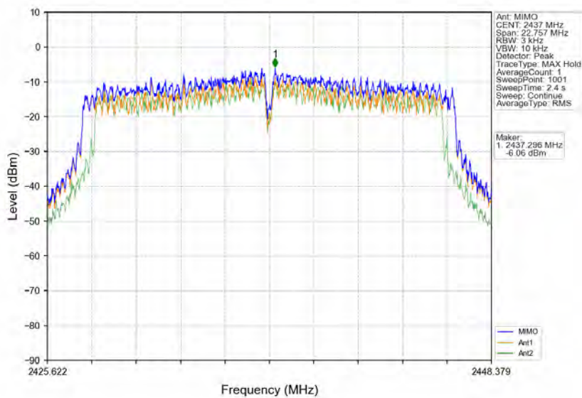
802.11n(HT20)_MCH_2437MHz_MIMO_NTNV
