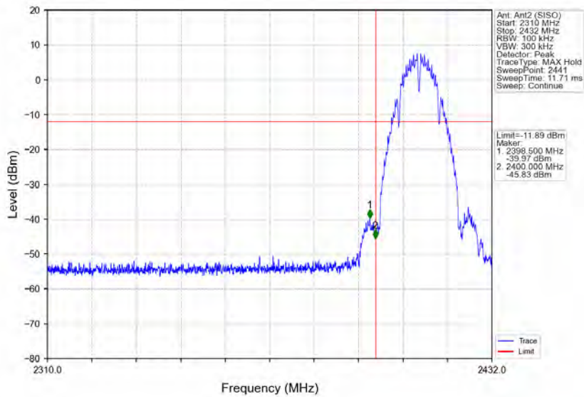
802.11b_LCH_2412MHz_Ant2 (SISO)_NTNV
