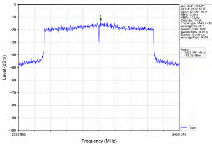
802.11ax(HEW40)_LCH_2422MHz_RU484_Left_Ant1 (MIMO)_NTNV
