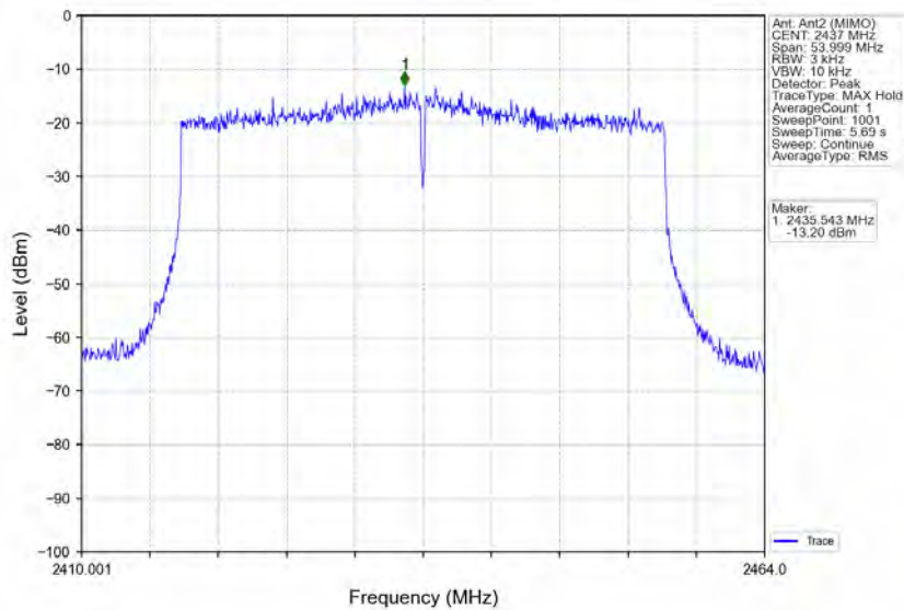
802.11ax(HEW40)_MCH_2437MHz_RU484_Left_Ant2 (MIMO)_NTNV
