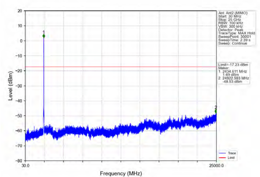
802.11ax(HEW40)_MCH_2437MHz_RU484_Left_Ant2 (MIMO)_NTNV
