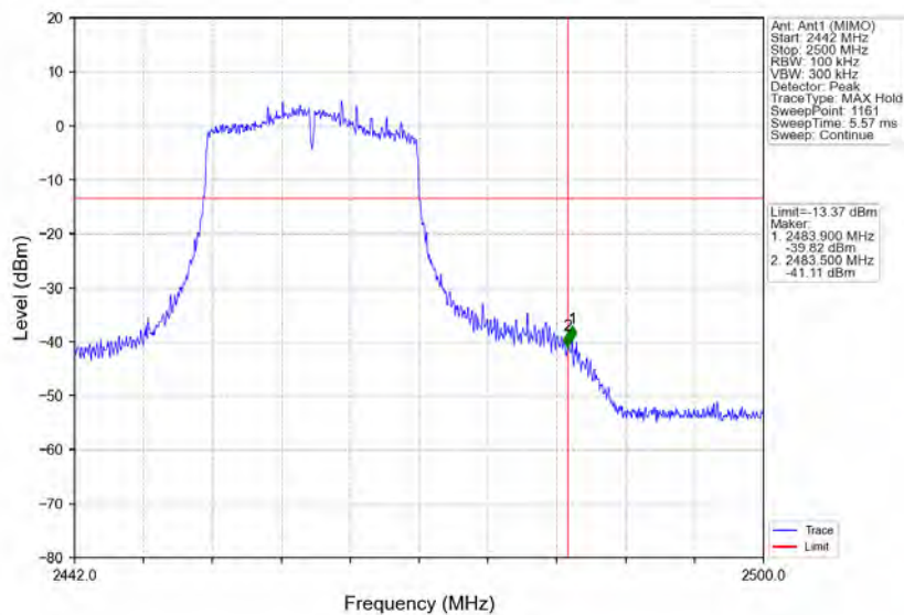
802.11n(HT20)_HCH_2462MHz_Ant1 (MIMO)_NTNV
