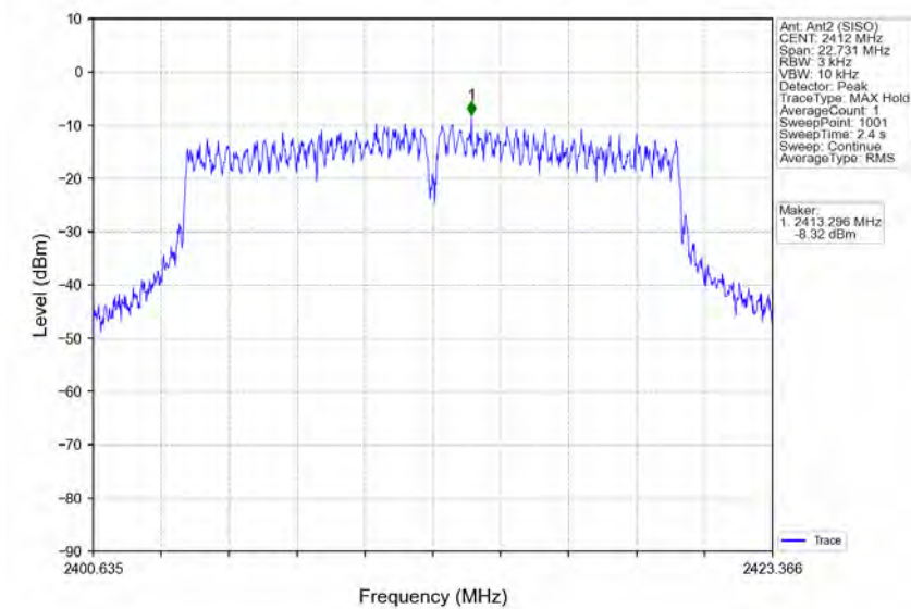
802.11g_LCH_2412MHz_Ant2 (SISO)_NTNV
