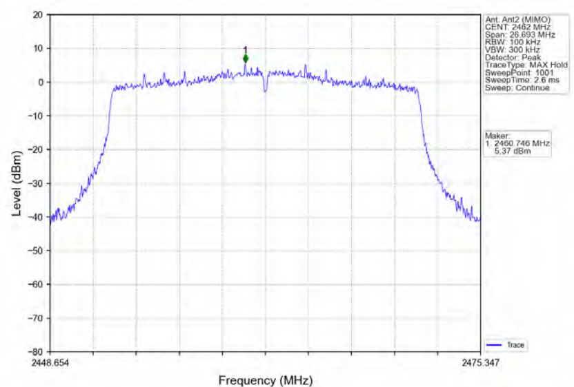
802.11ax(HEW20)_HCH_2462MHz_RU242_Left_Ant2 (MIMO)_NTNV
