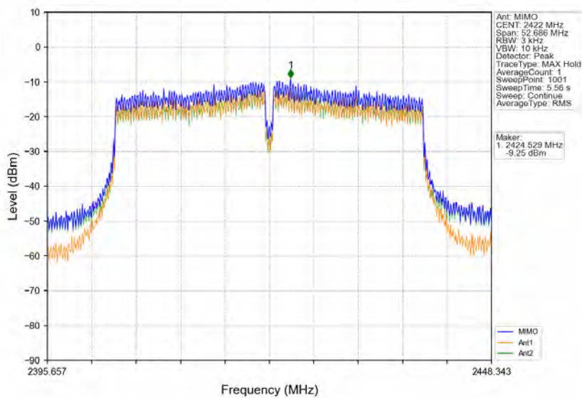
802.11n(HT40)_LCH_2422MHz_MIMO_NTNV
