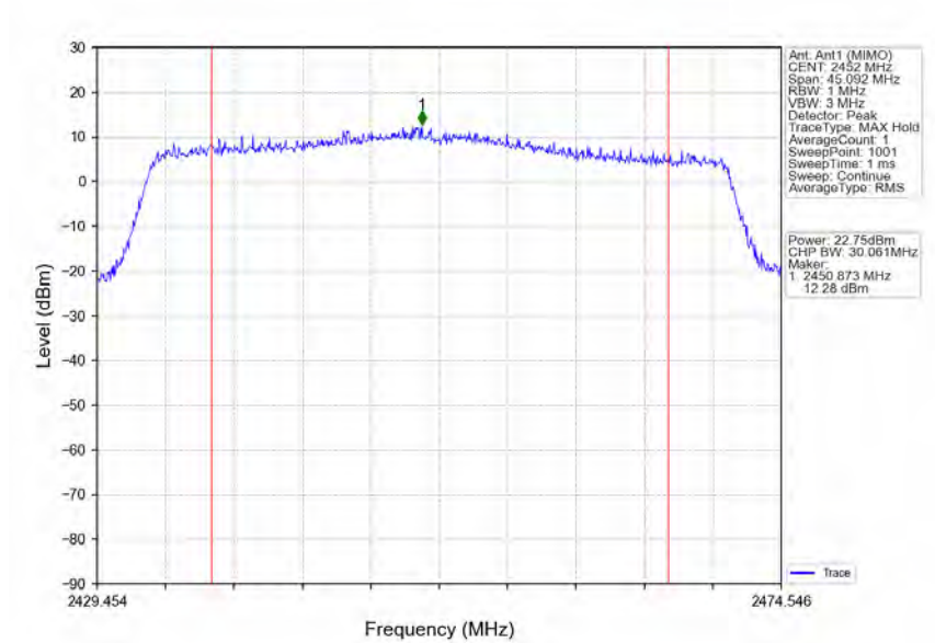
802.11ax(HEW40)_HCH_2452MHz_RU484_Left_Ant1 (MIMO)_NTNV
