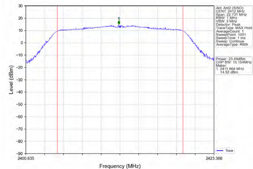
802.11g_LCH_2412MHz_Ant2 (SISO)_NTNV
