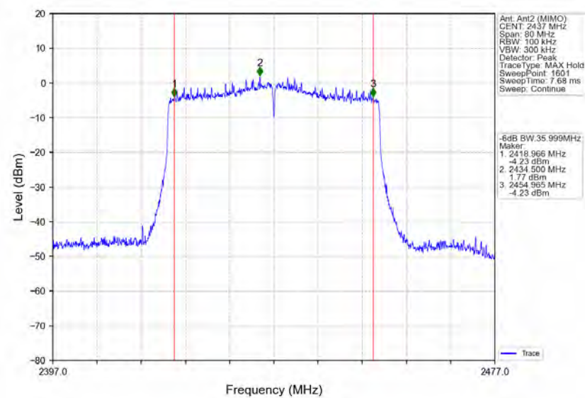
802.11ax(HEW40)_MCH_2437MHz_RU484_Left_Ant2 (MIMO)_NTNV
