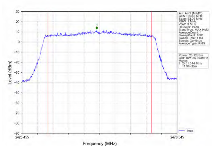
802.11ax(HEW40)_HCH_2452MHz_RU484_Left_Ant2 (MIMO)_NTNV
