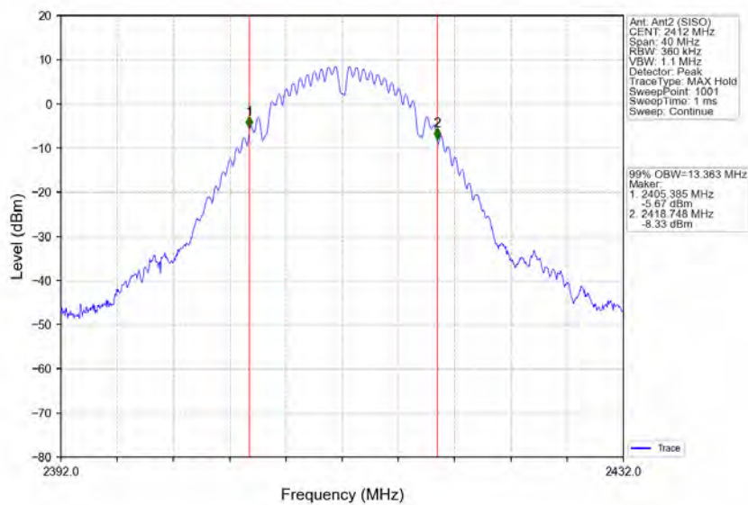
802.11b_LCH_2412MHz_Ant2 (SISO)_NTNV
