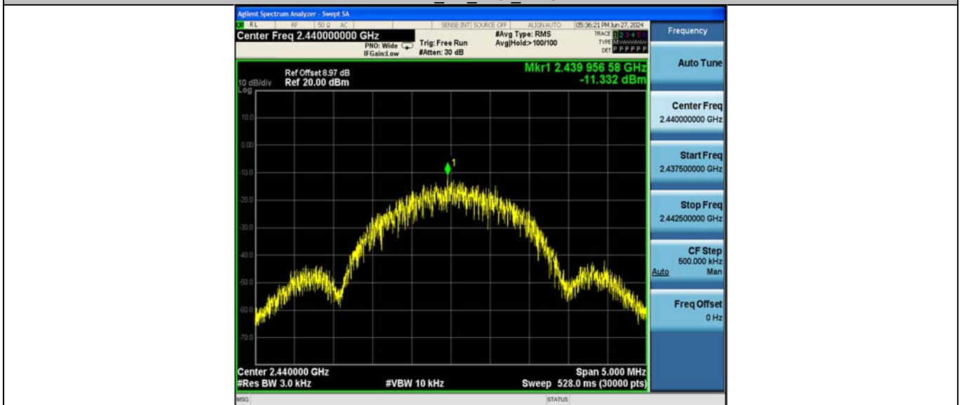
BLE_2M_Ant2_2440
